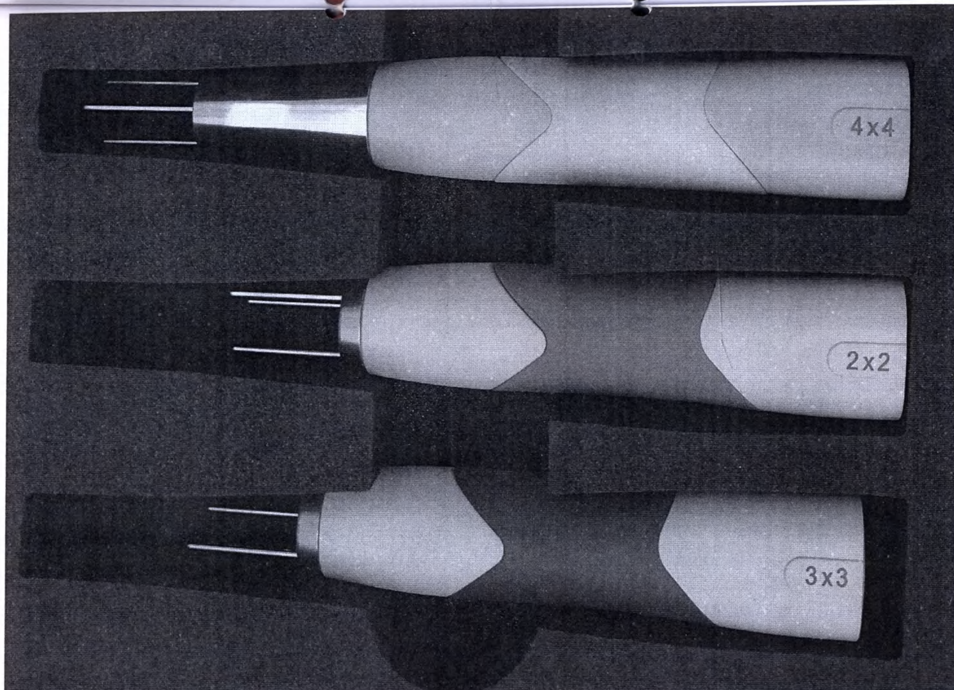
Q-switch насадка с размером пятна 2x2 мм, 3x3 мм, 4x4 мм
