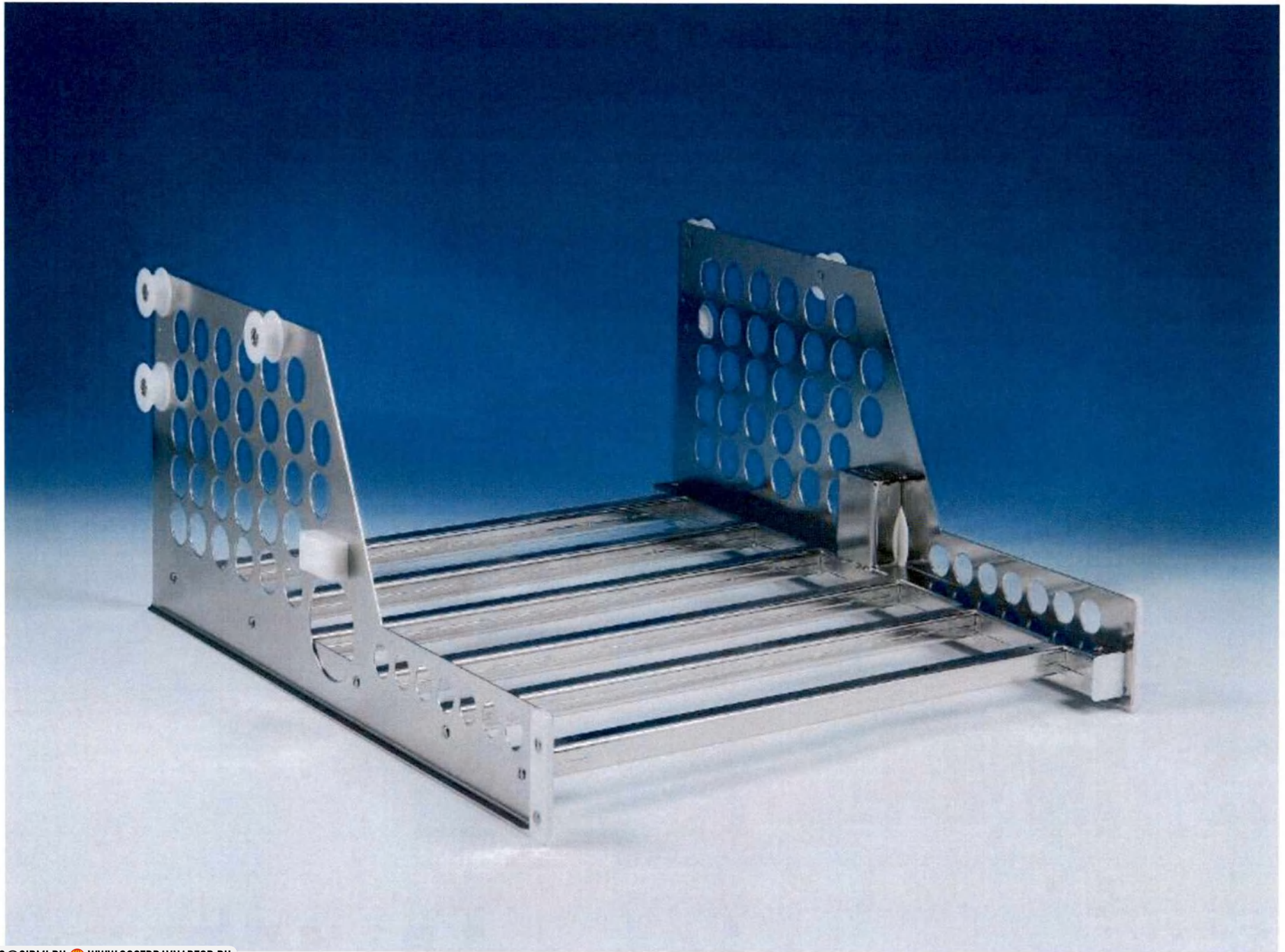
34. Тележка верхняя для кассеты инжекторной (1 шт. или более 1 шт.)
