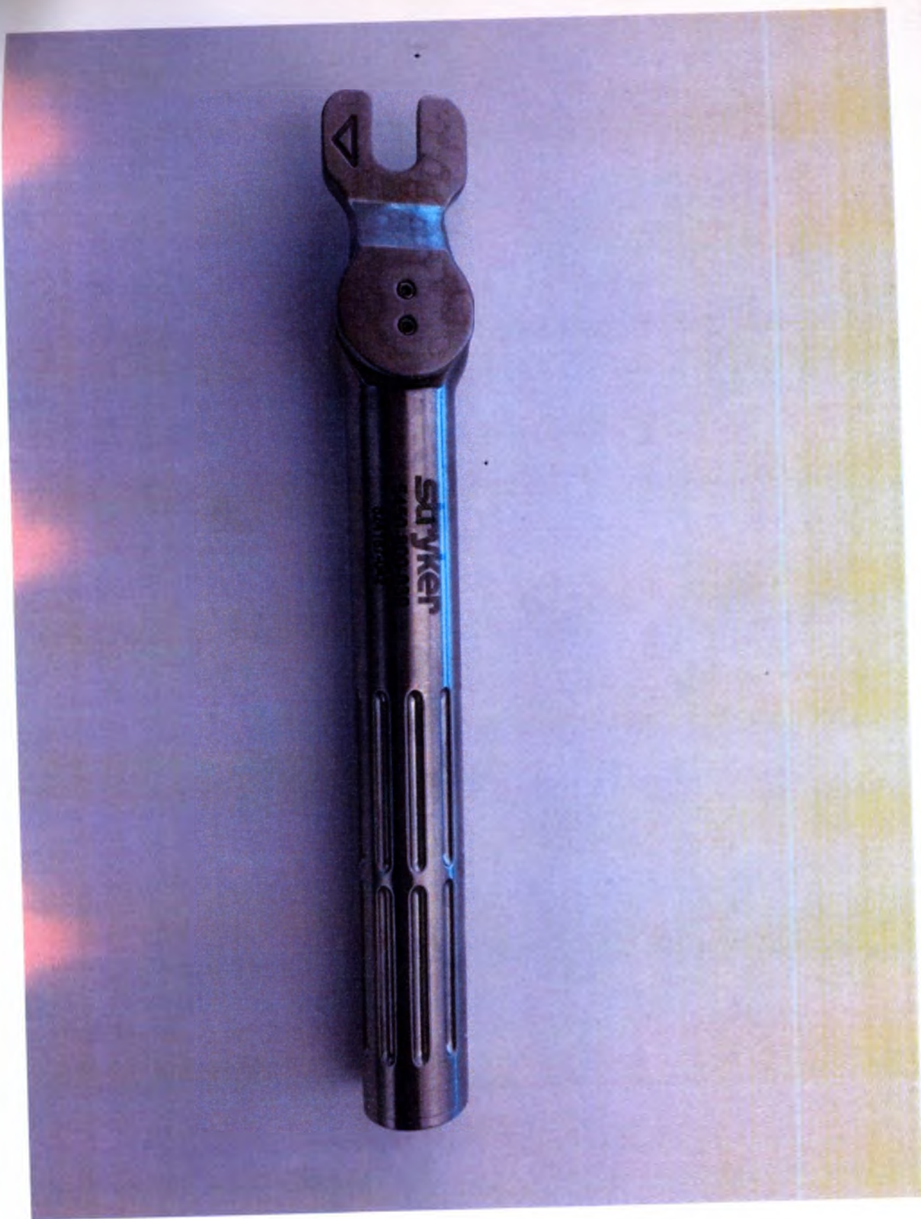
Ключ динамометрический шаговый, 7 мм
