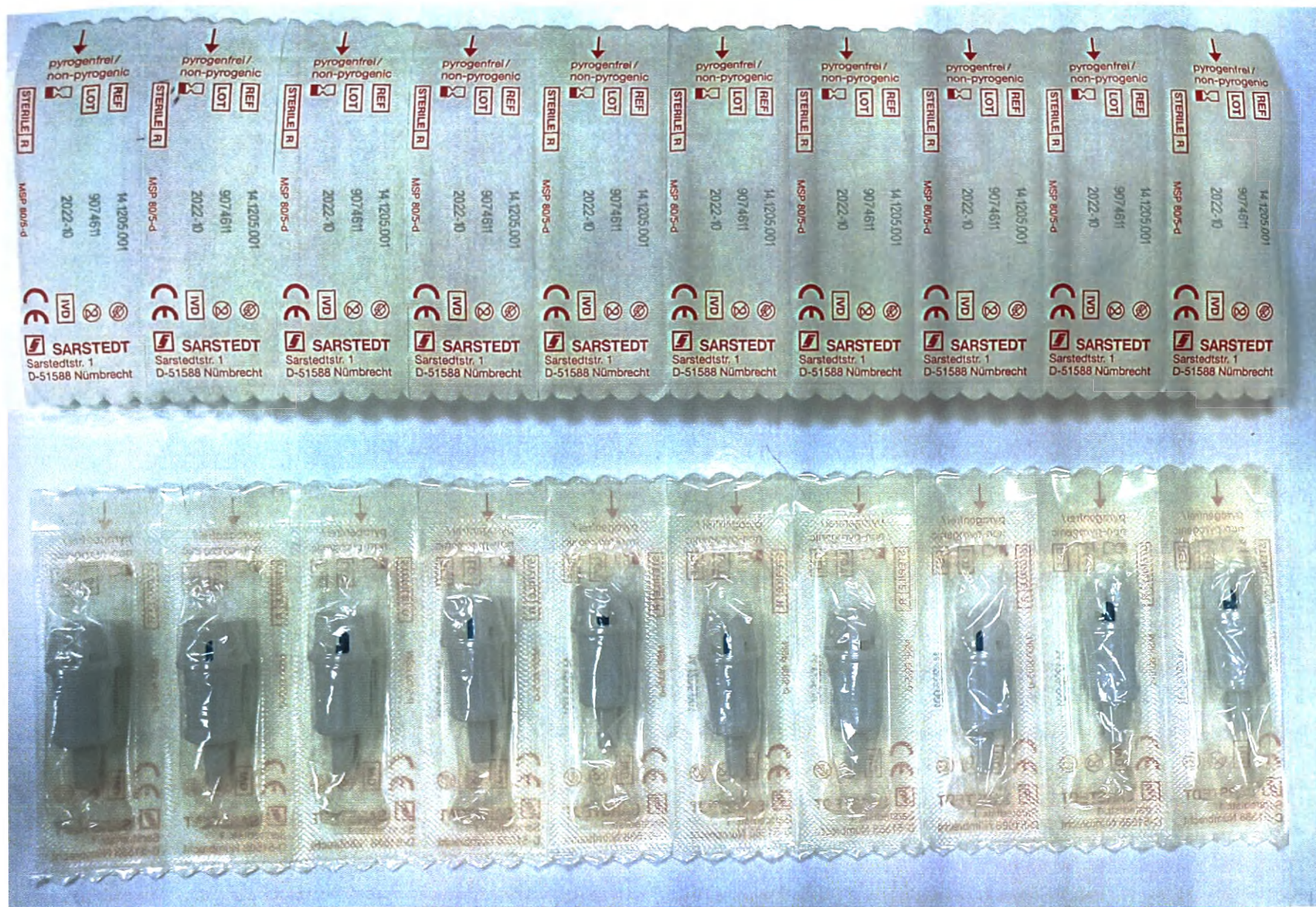
Рис 10. Индивидуальная упаковка. Переходник мульти-адаптер с укороченным наконечником
