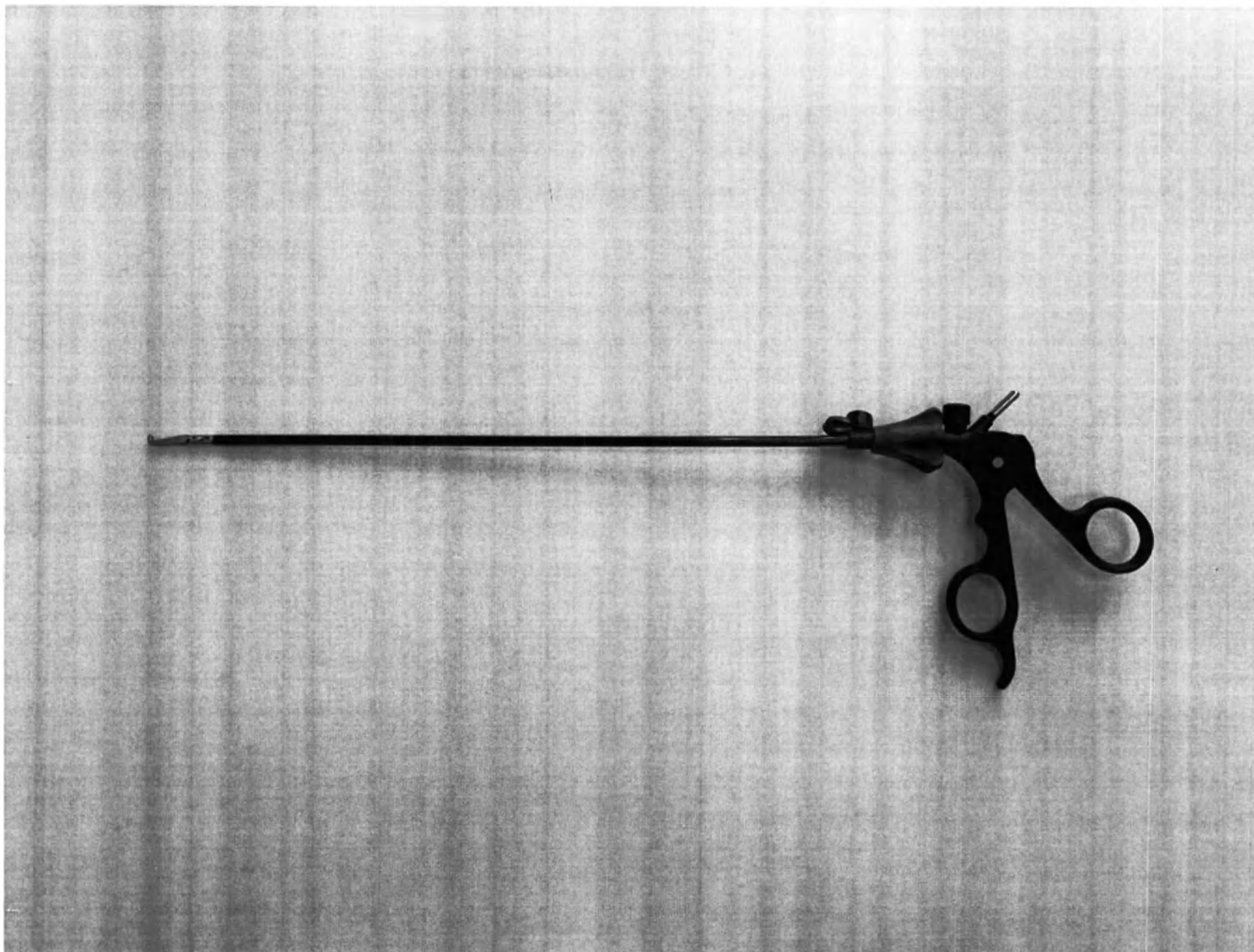
Фотографическое изображение 121. Инструмент электрохирургический с подвижными браншами Исп. 7
