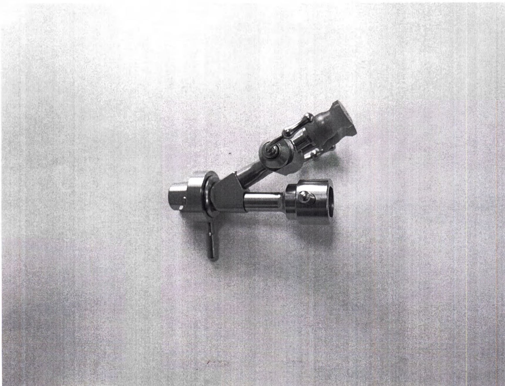
Фотографическое изображение 727. Переходник для введения гибких инструментов Исп.3
