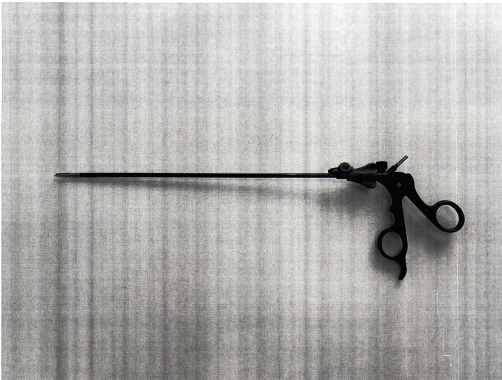
Фотографическое изображение 116. Инструмент электрохирургический с подвижными браншами Исп. 2
