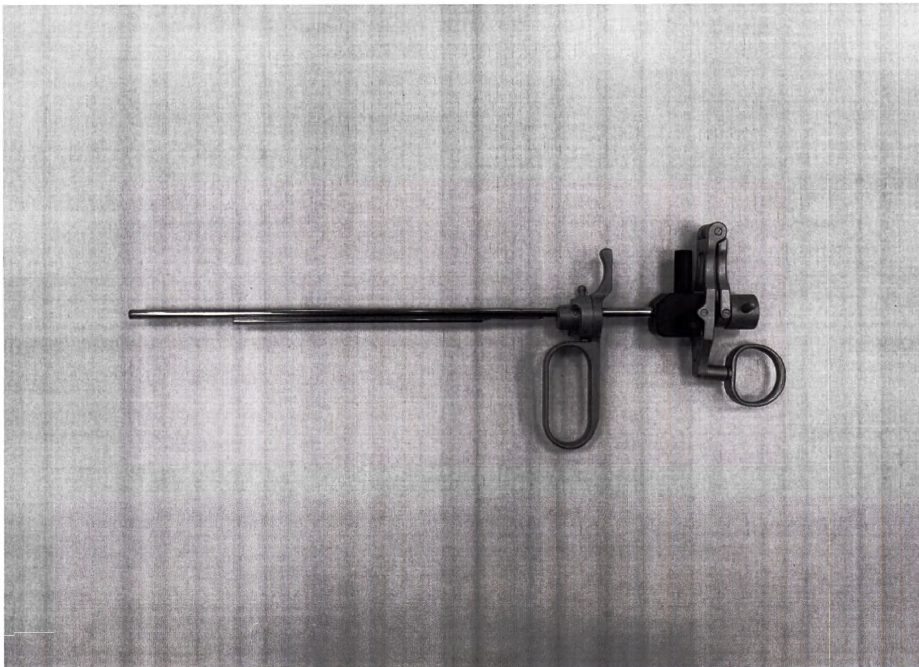
Фотографическое изображение 635. Держатель инструмента электрода с направителем Исп. 1
