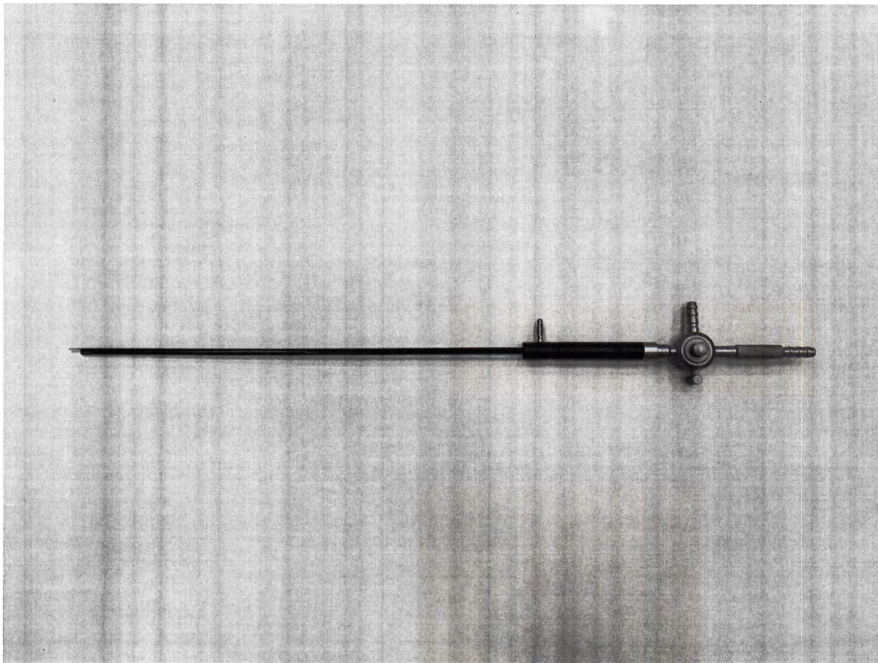
Фотографическое изображение 114. Инструмент электрод с рукояткой Исп. 52
