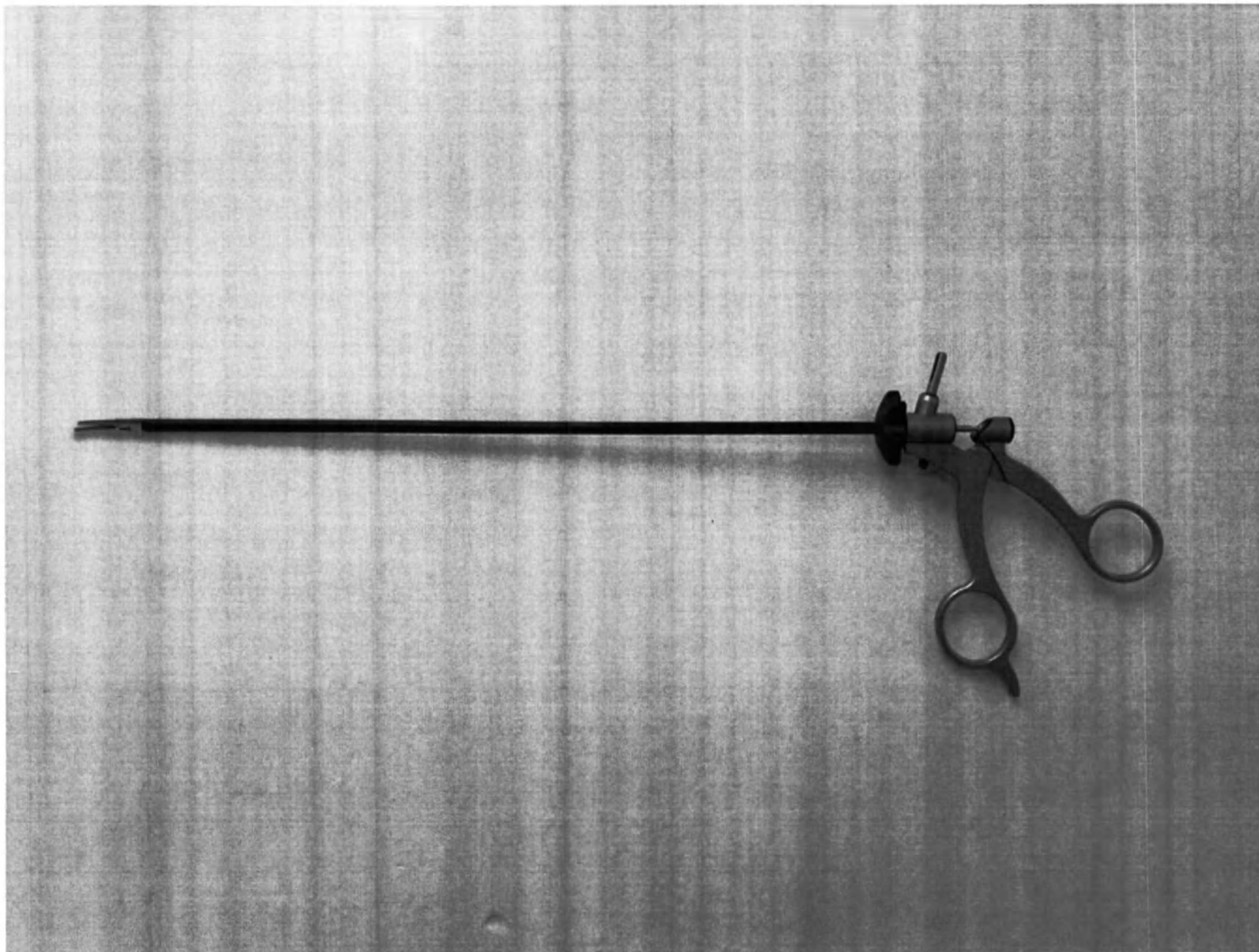
Фотографическое изображение 191. Инструмент электрохирургический с подвижными браншами Исп. 77
