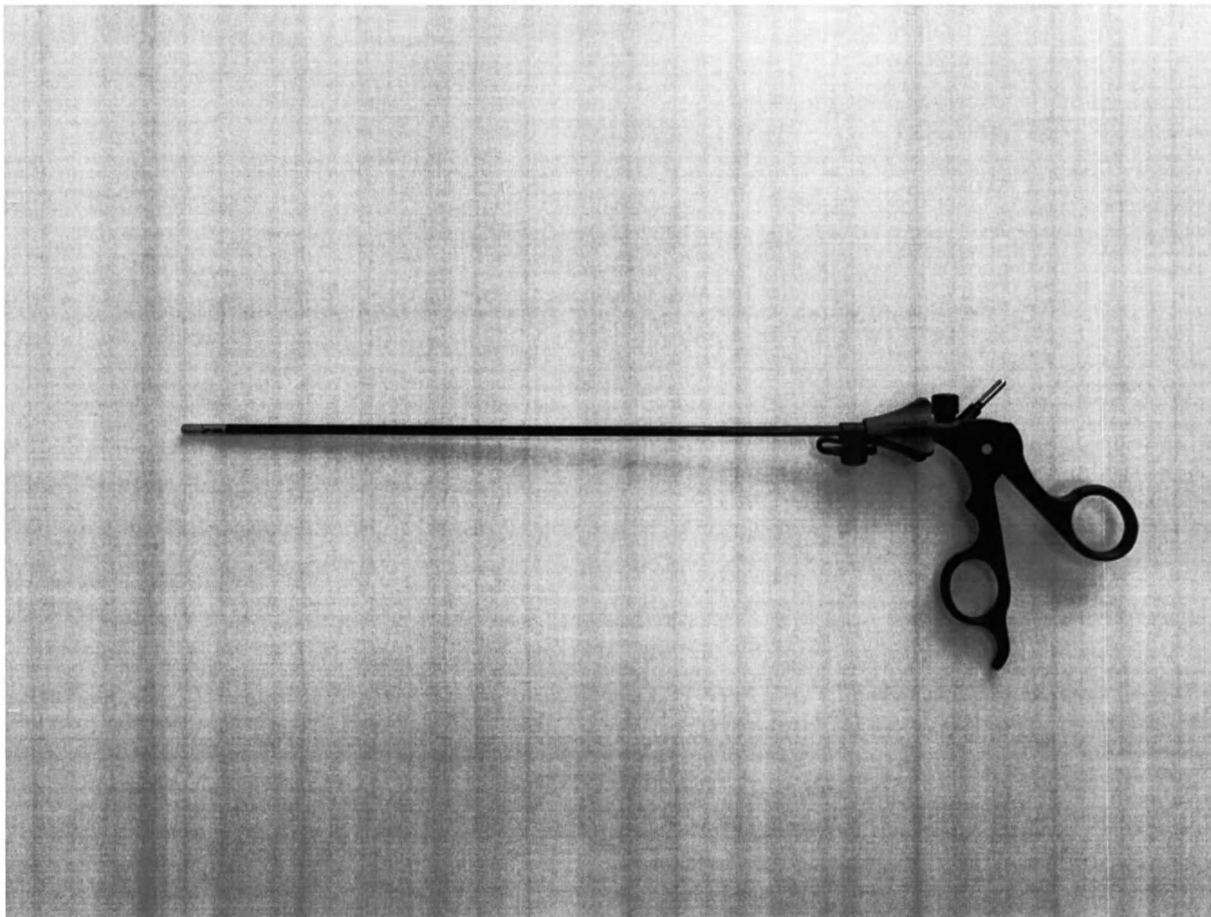
Фотографическое изображение 123. Инструмент электрохирургический с подвижными браншами Исп. 9
