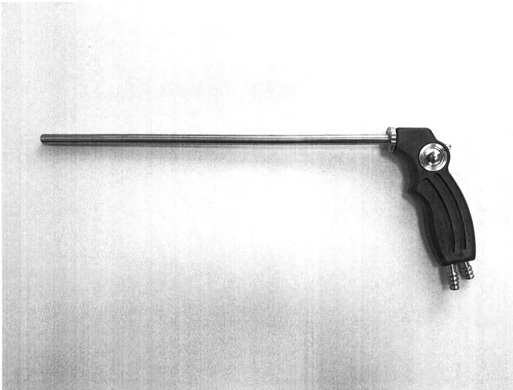
Фотографическое изображение 720. Трубка с клапаном для очистки и промывания операционного поля Исп. 2
