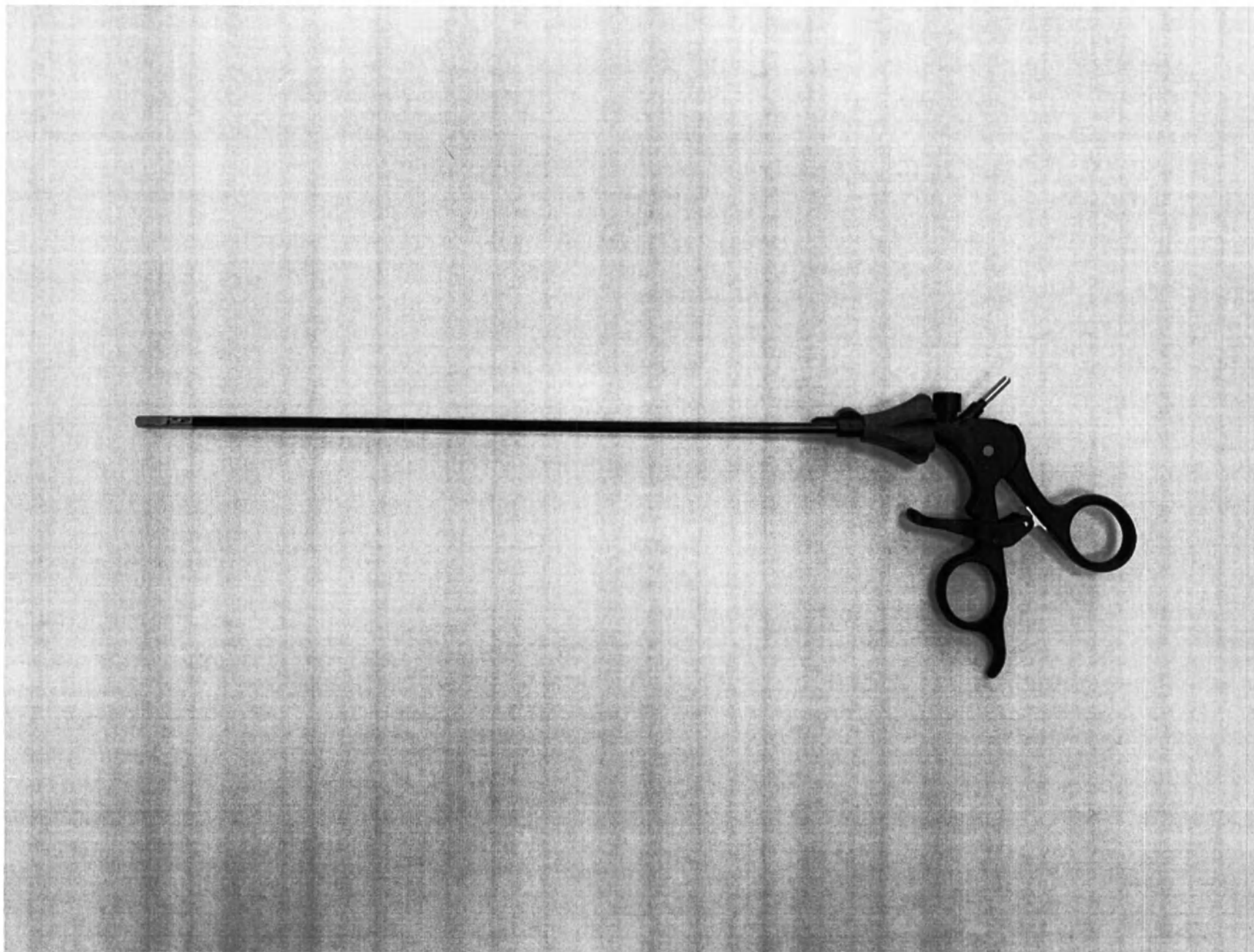
Фотографическое изображение 147. Инструмент электрохирургический с подвижными браншами Исп. 33
