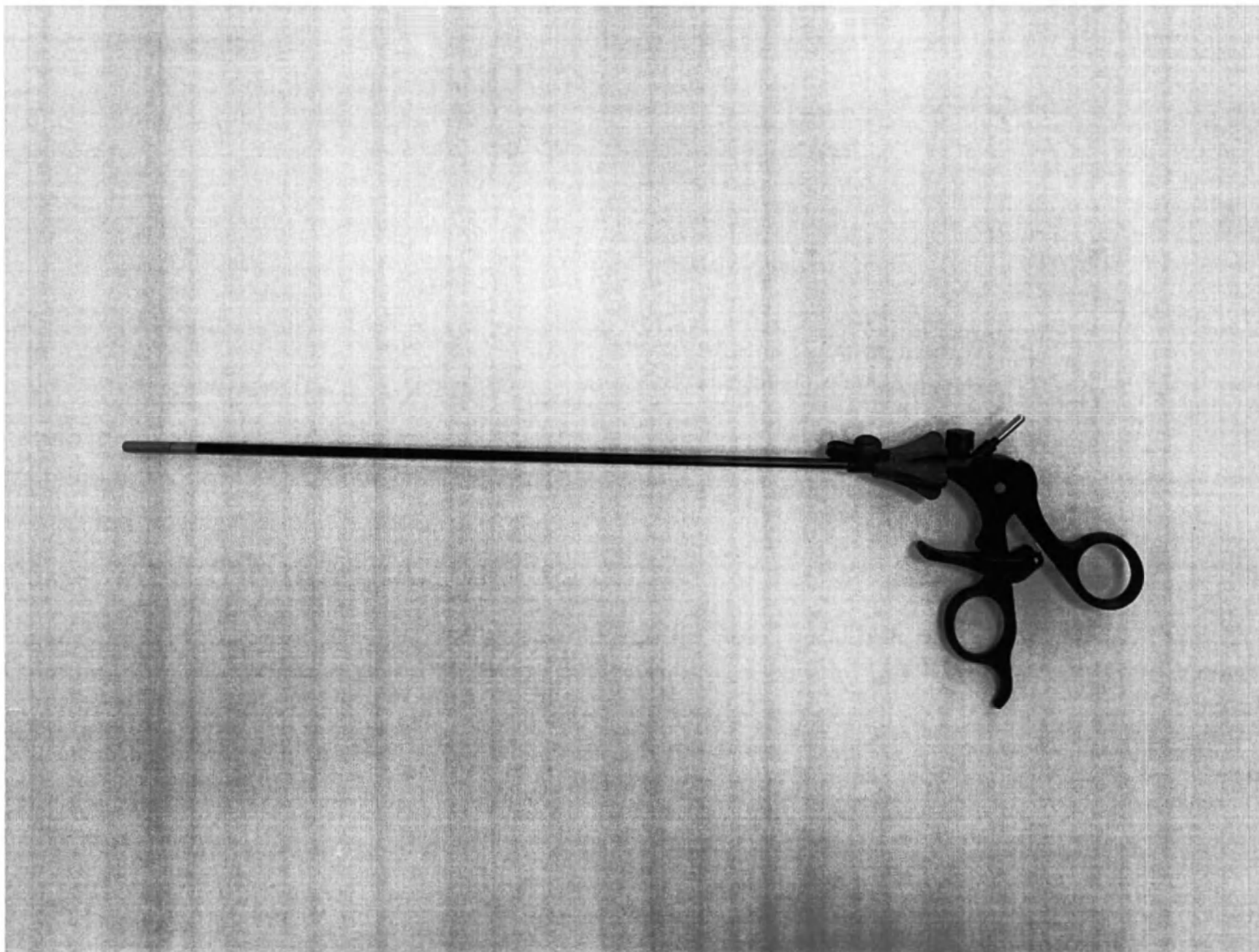
Фотографическое изображение 160. Инструмент электрохирургический с подвижными браншами Исп. 46
