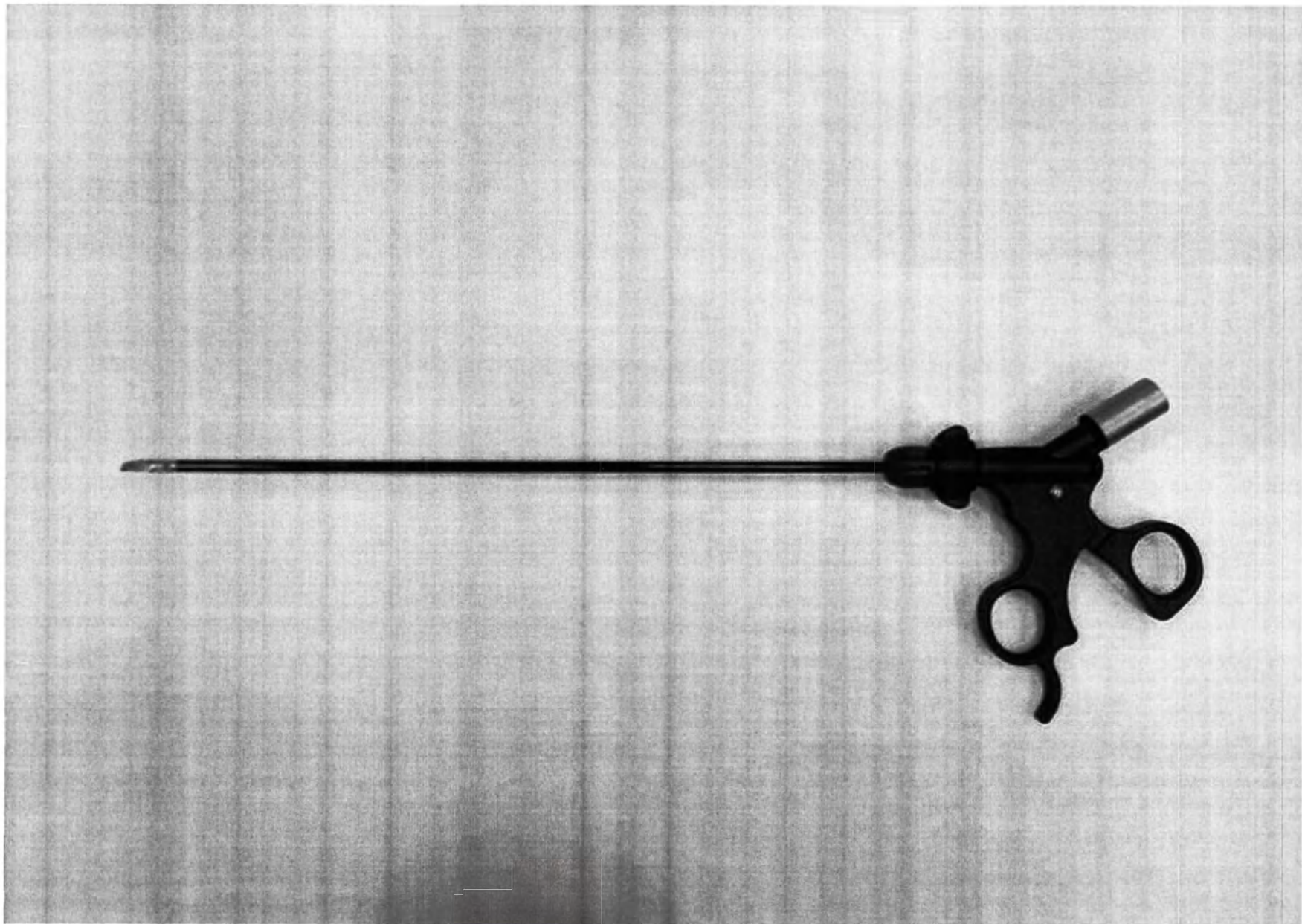
Фотографическое изображение 273. Инструмент электрохирургический с подвижными браншами Исп. 159
