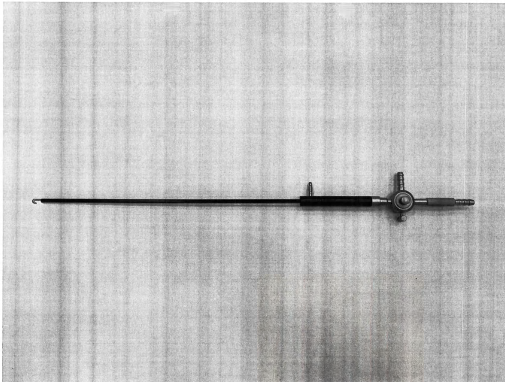
Фотографическое изображение 113. Инструмент электрод с рукояткой Исп. 51
