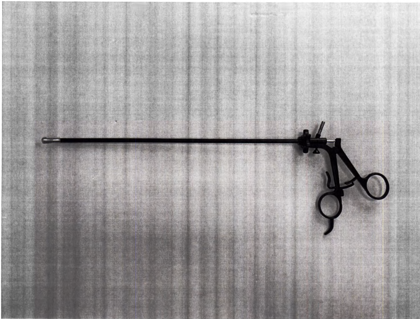
Фотографическое изображение 237. Инструмент электрохирургический с подвижными браншами Исп. 123
