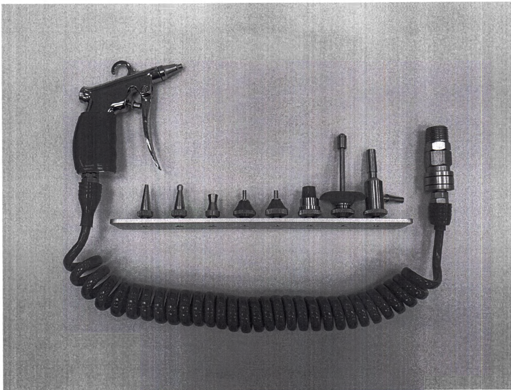
Фотографическое изображение 749. Устройство промывочное Исп. 1
