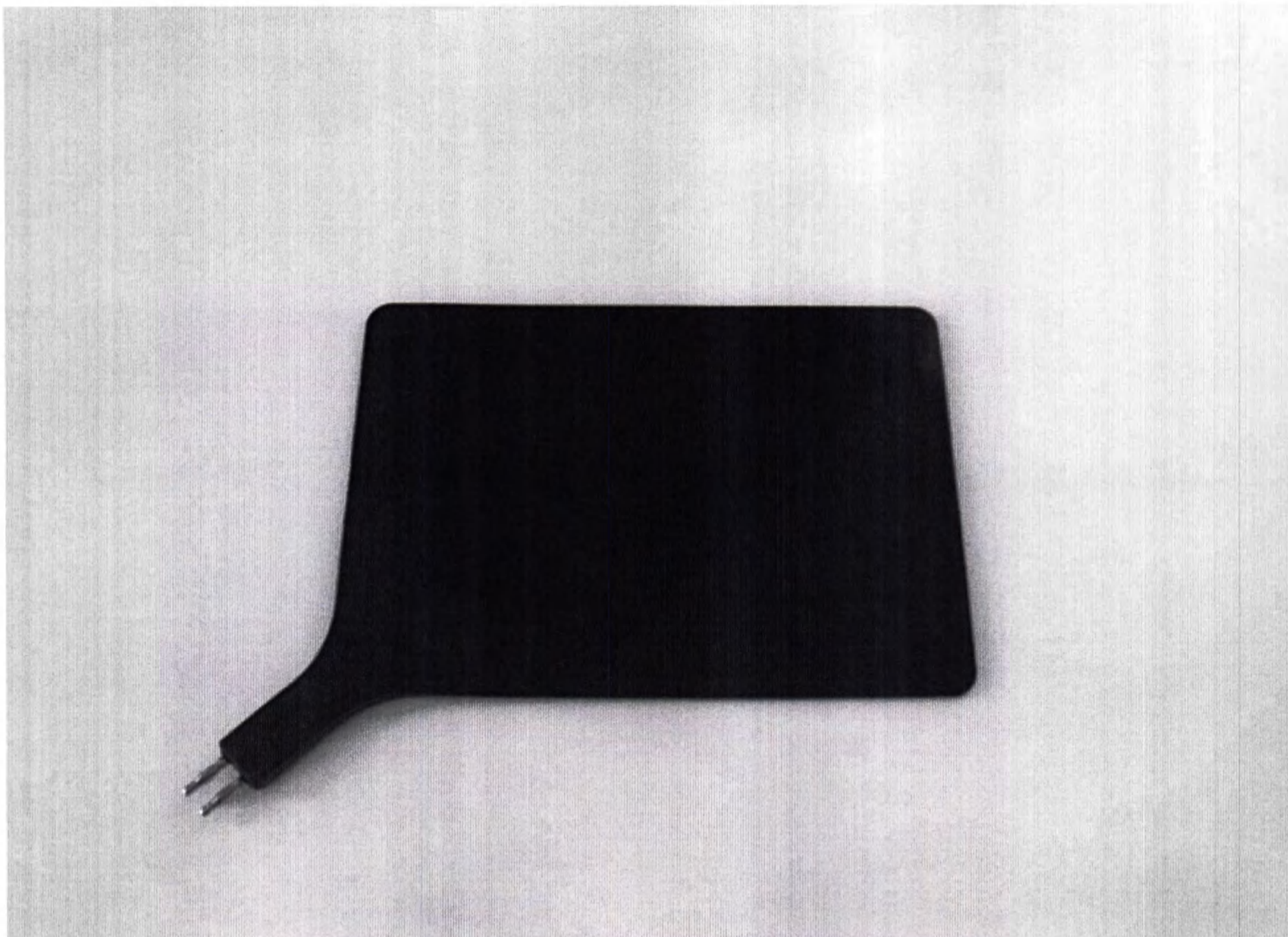
Фотографическое изображение 729. Электрод нейтральный
