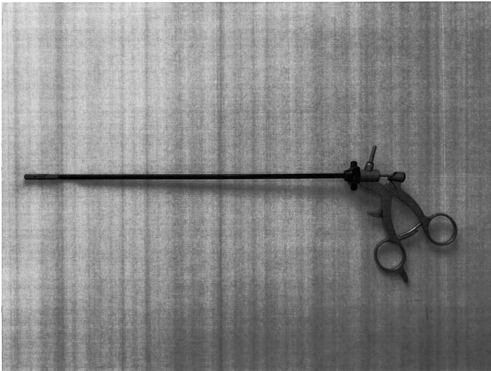
Фотографическое изображение 204. Инструмент электрохирургический с подвижными браншами Исп. 90
