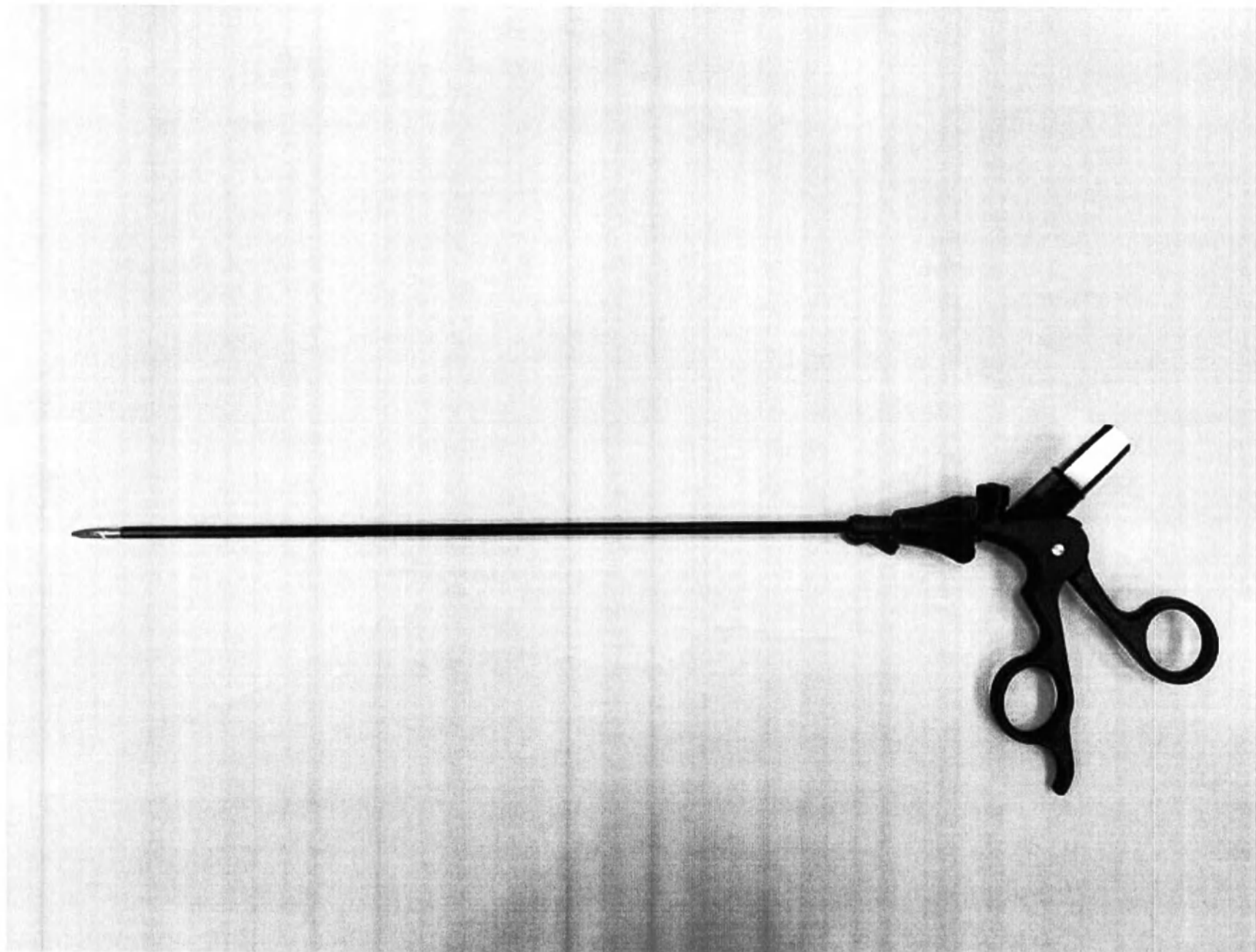
Фотографическое изображение 261. Инструмент электрохирургический с подвижными браншами Исп. 147
