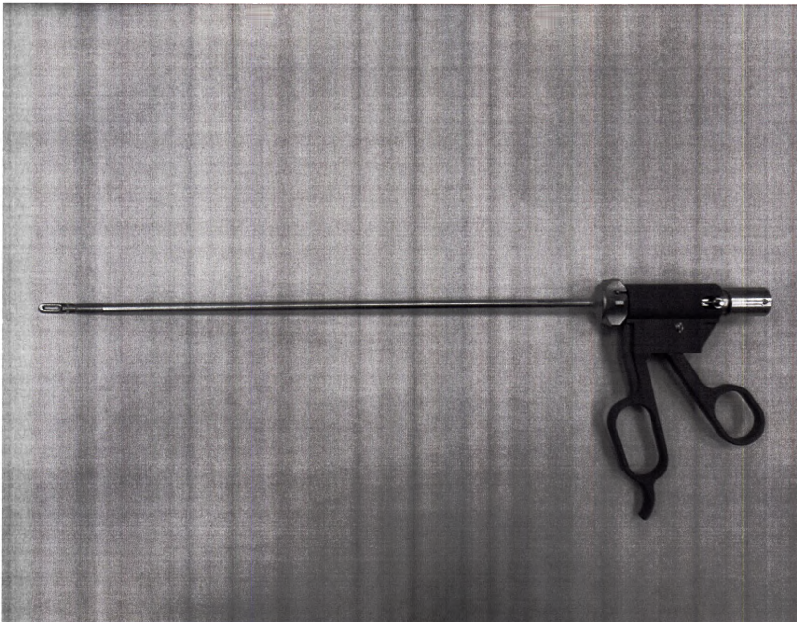
Фотографическое изображение 294. Инструмент электрохирургический с подвижными браншами Исп. 180
