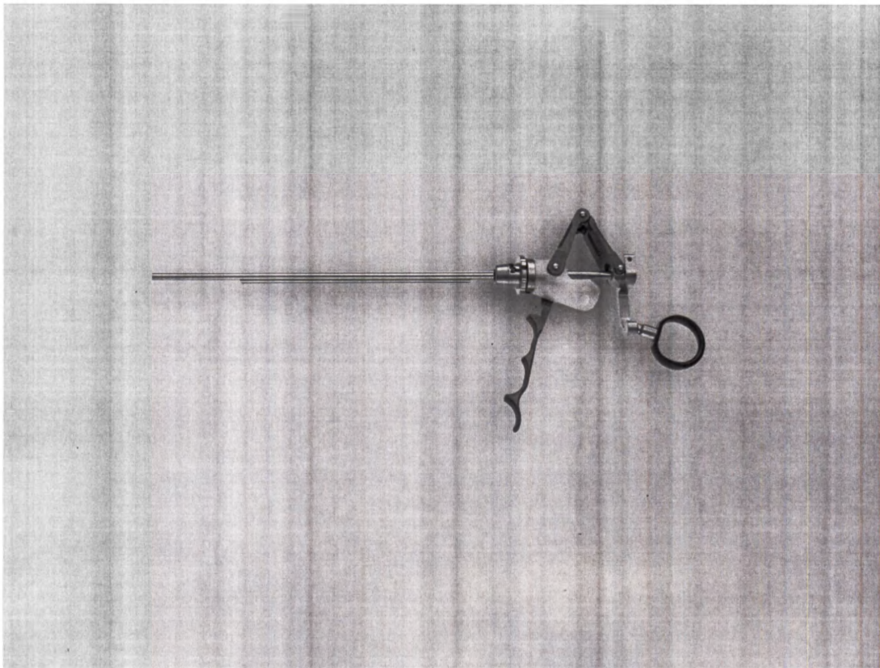
Фотографическое изображение 642. Держатель инструмента электрода с направителем Исп. 8
