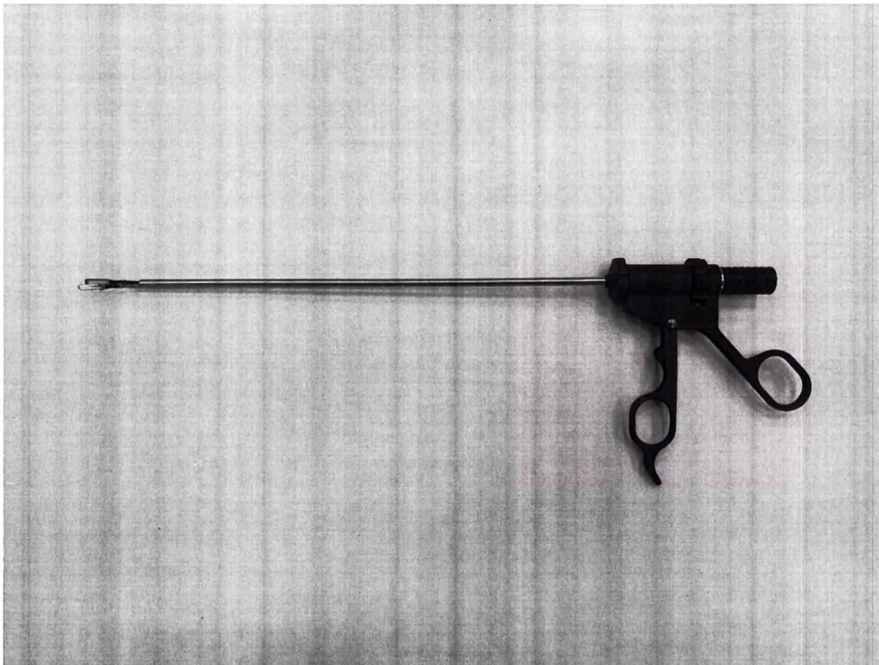
Фотографическое изображение 297. Инструмент электрохирургический с подвижными браншами Исп. 183
