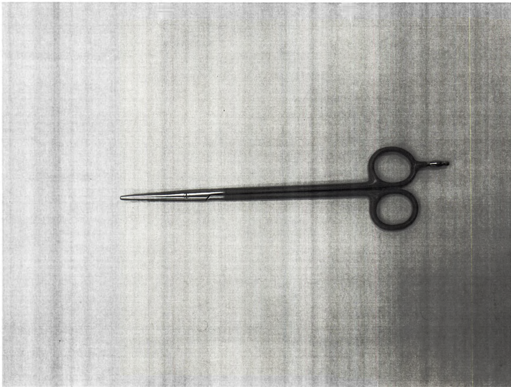
Фотографическое изображение 58. Инструмент электрод ножницы Исп. 1
