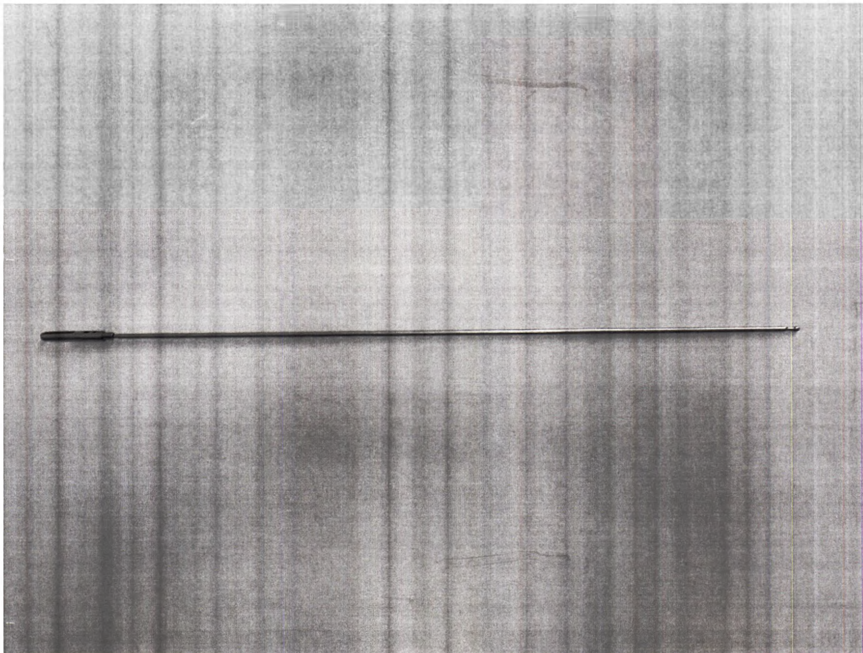
Фотографическое изображение 352. Инструмент электрод-вставка с подвижными браншами Исп. 41
