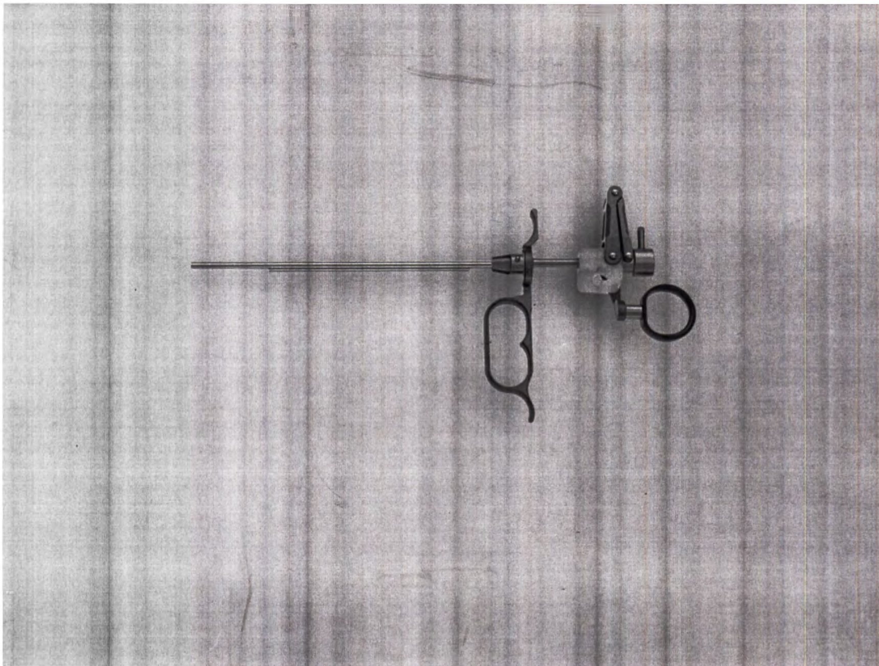
Фотографическое изображение 639. Держатель инструмента электрода с направителем Исп. 5
