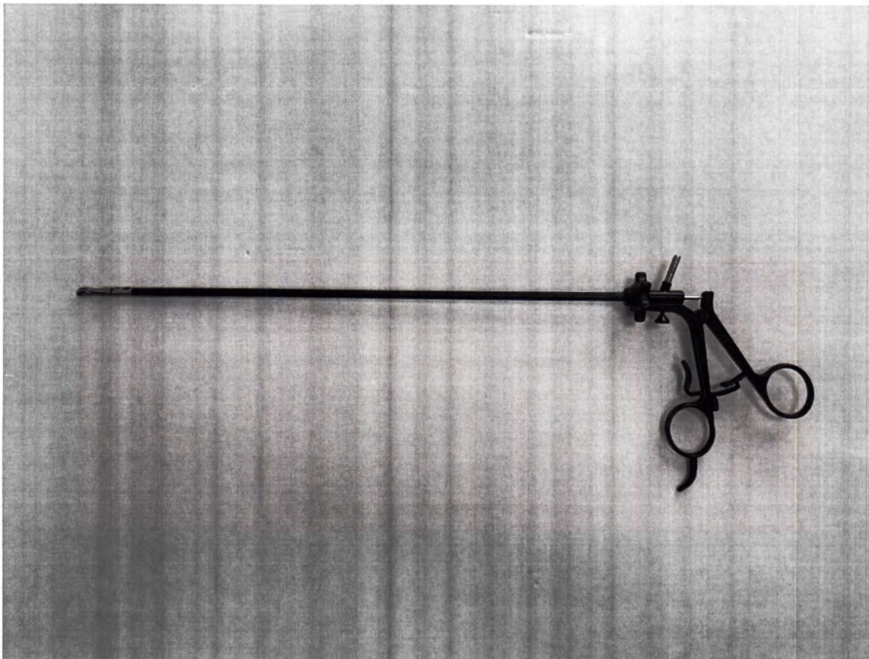
Фотографическое изображение 244. Инструмент электрохирургический с подвижными браншами Исп. 130
