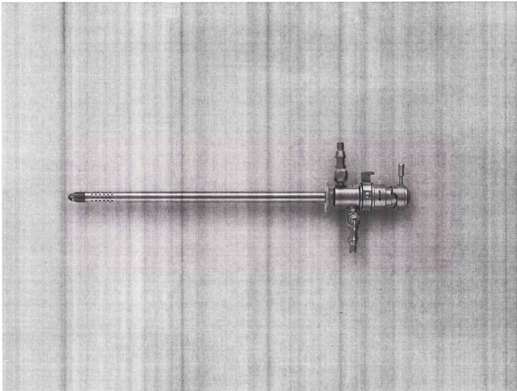
Фотографическое изображение 657. Изолятор-трубка инструмента электрода с направителем Исп. 3
