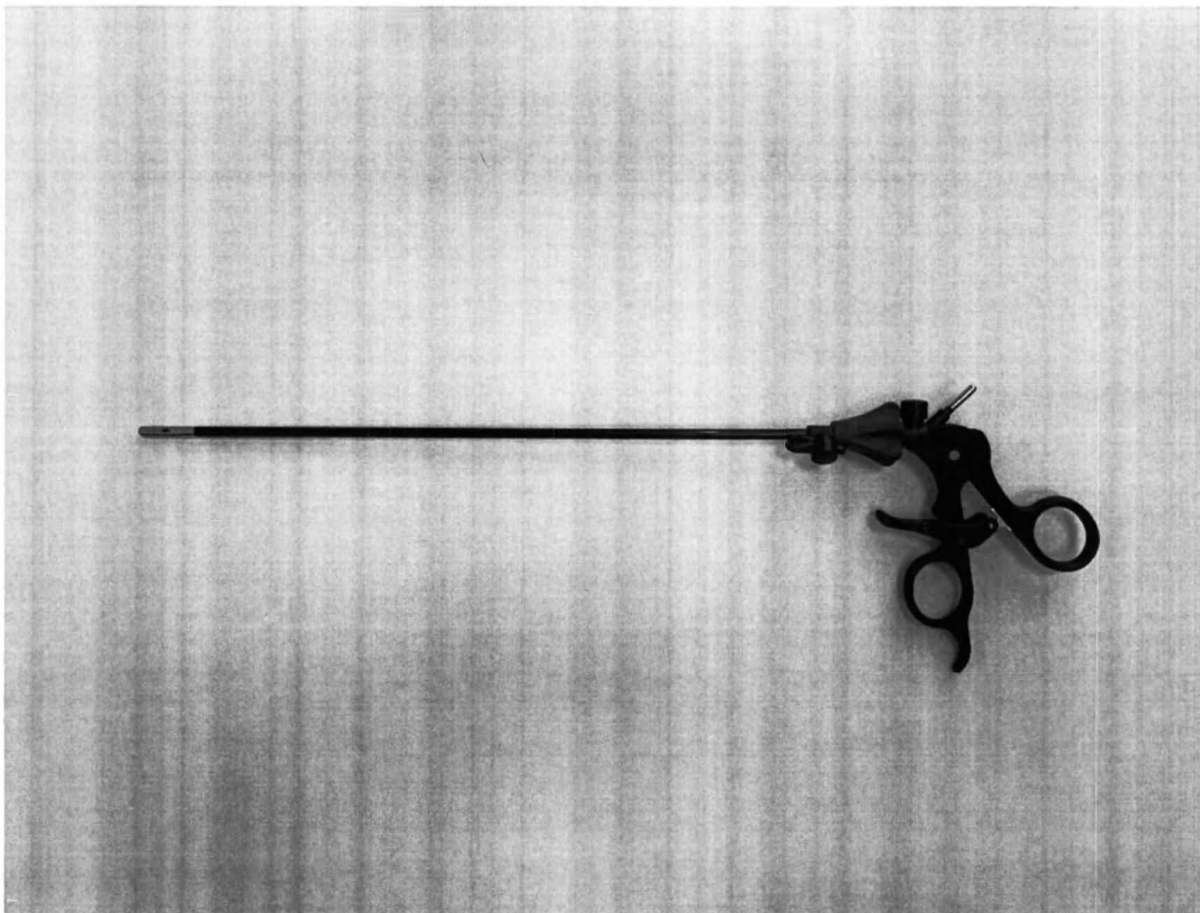
Фотографическое изображение 139. Инструмент электрохирургический с подвижными браншами Исп. 25
