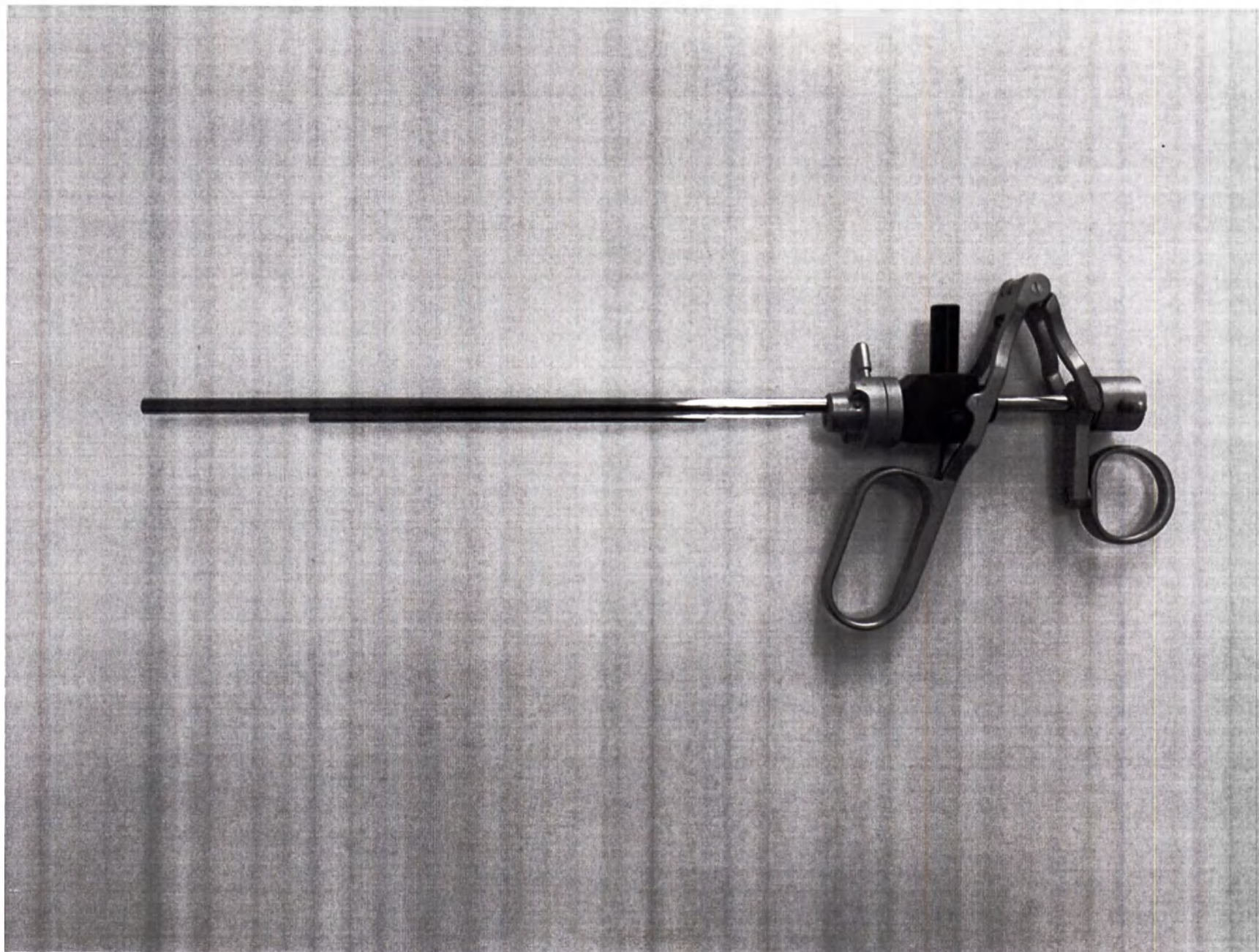
Фотографическое изображение 636. Держатель инструмента электрода с направителем Исп. 2
