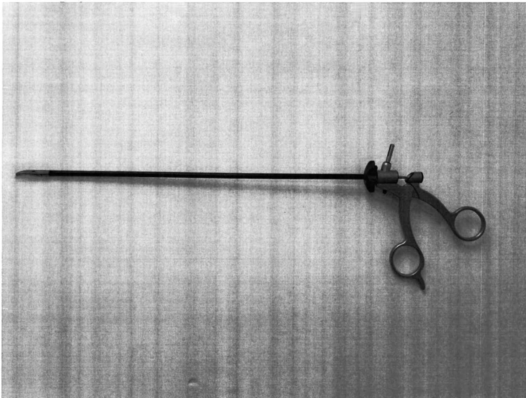
Фотографическое изображение 178. Инструмент электрохирургический с подвижными браншами Исп. 64
