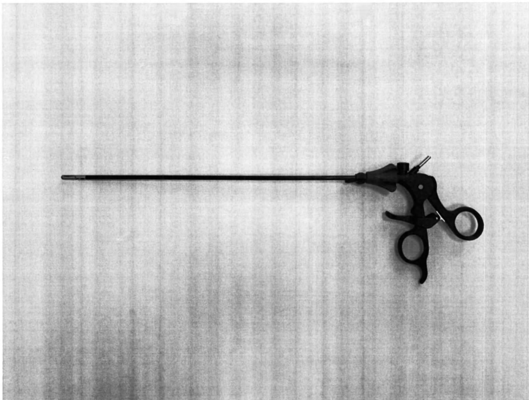
Фотографическое изображение 170. Инструмент электрохирургический с подвижными браншами Исп. 56
