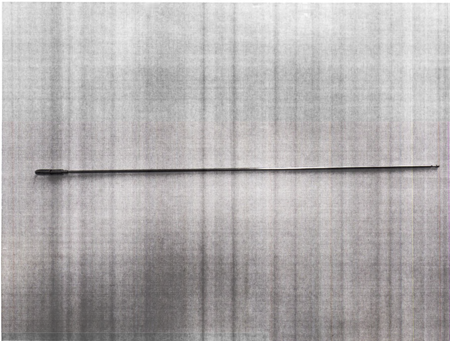
Фотографическое изображение 385. Инструмент электрод-вставка с подвижными браншами Исп. 74
