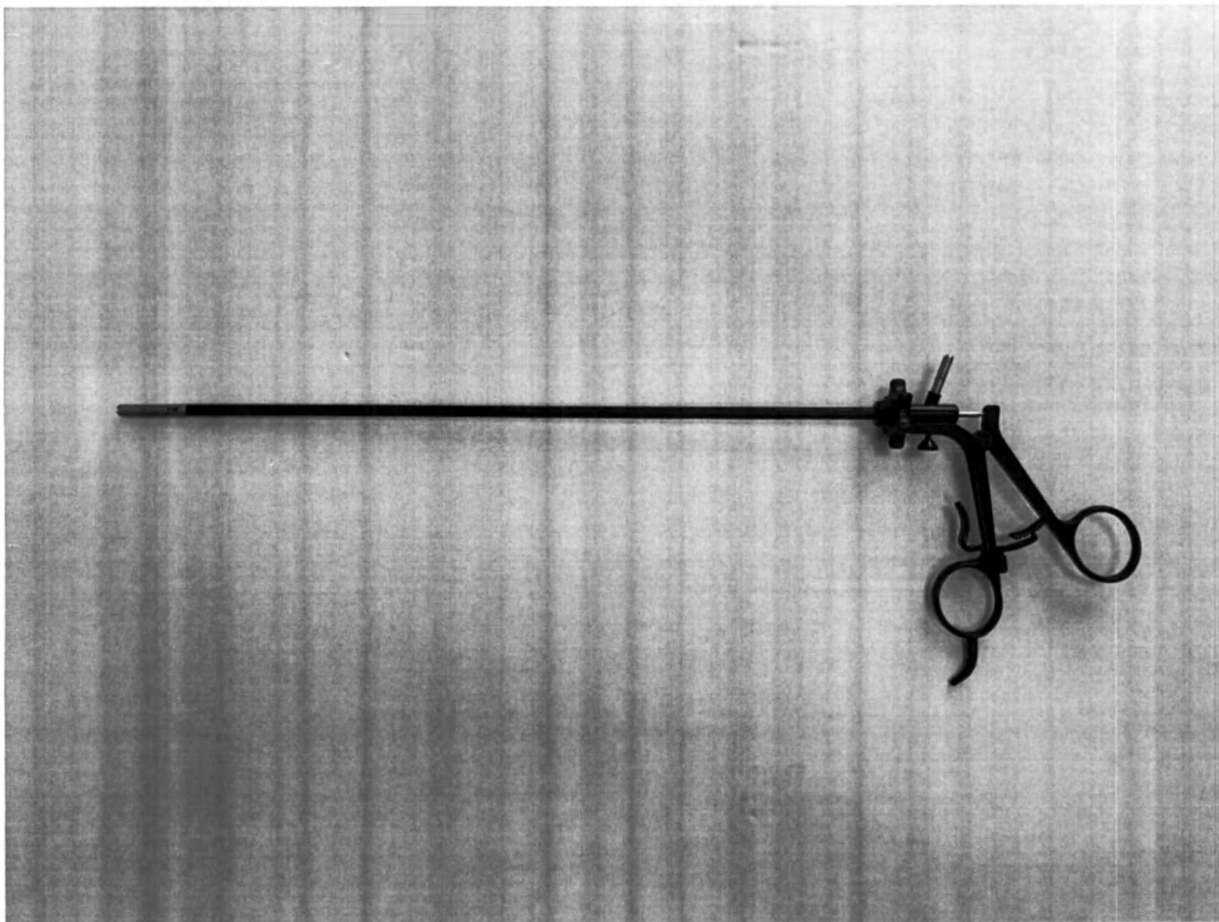
Фотографическое изображение 238. Инструмент электрохирургический с подвижными браншами Исп. 124
