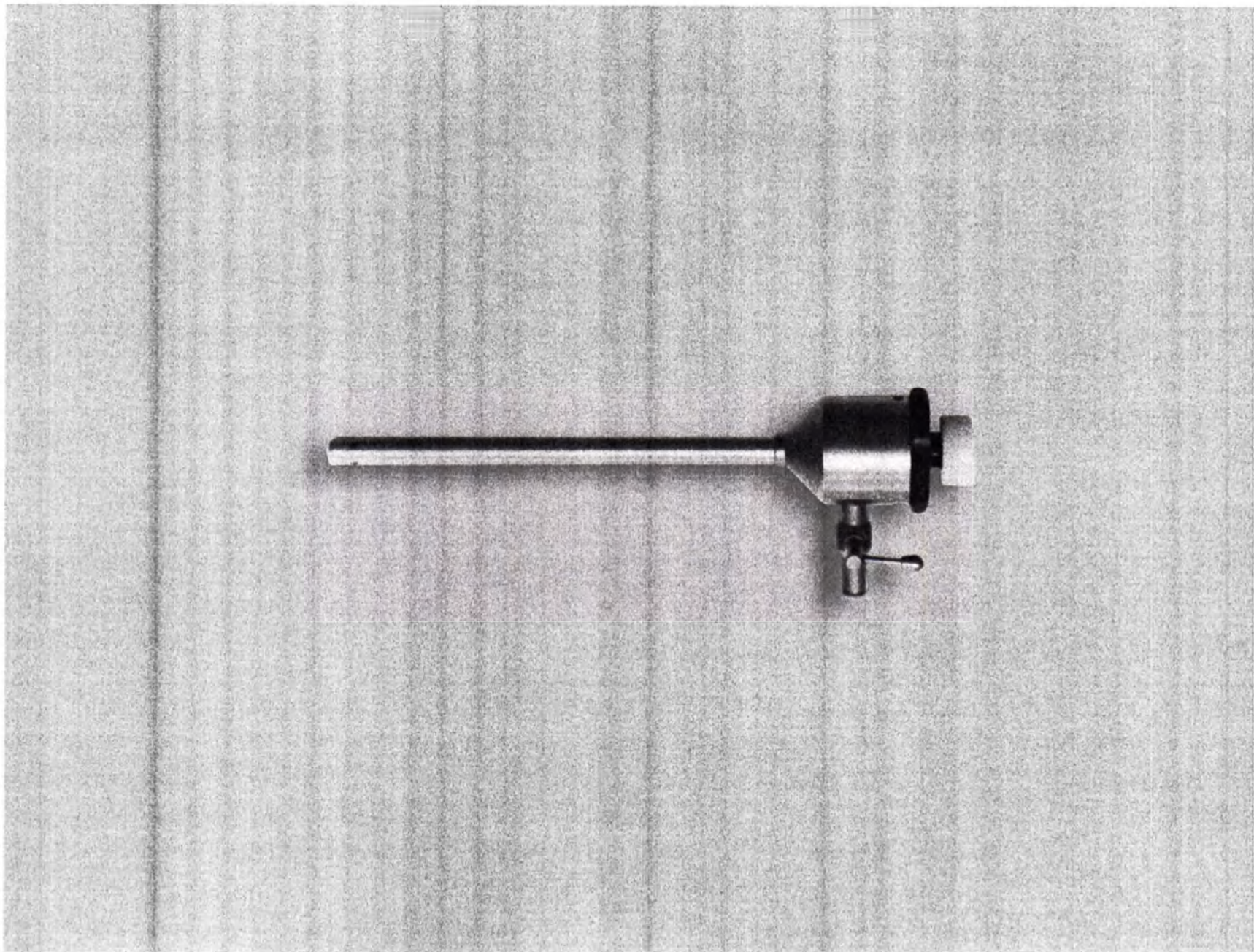
Фотографическое изображение 673. Трубка для введения инструментов Исп. 15
