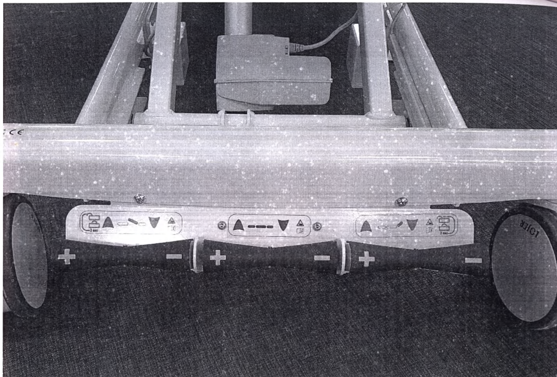
Комплект педалей для регулировки высоты, средней секции и сиденья
