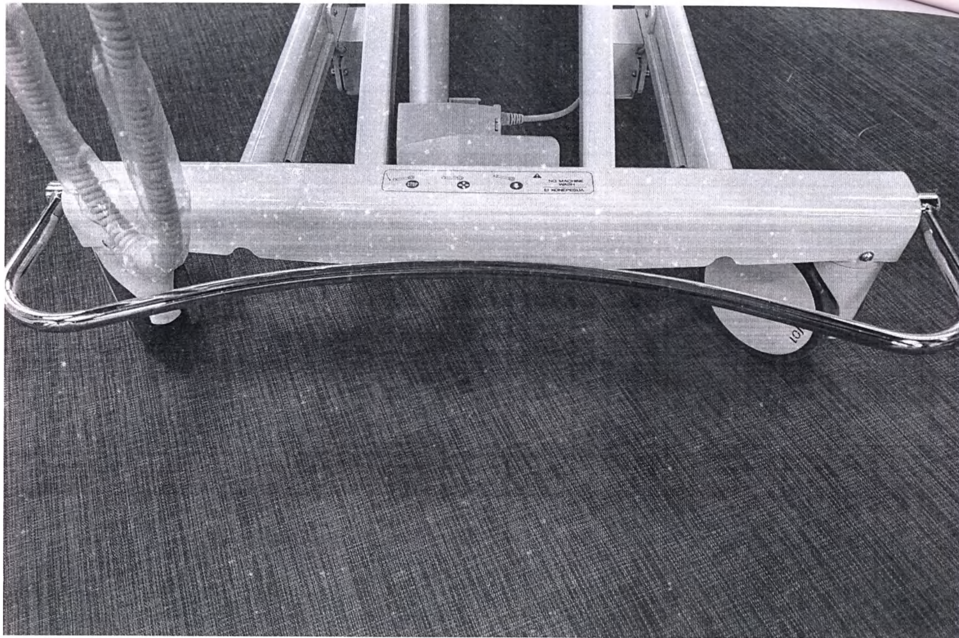
Педаль центральной блокировки колес
