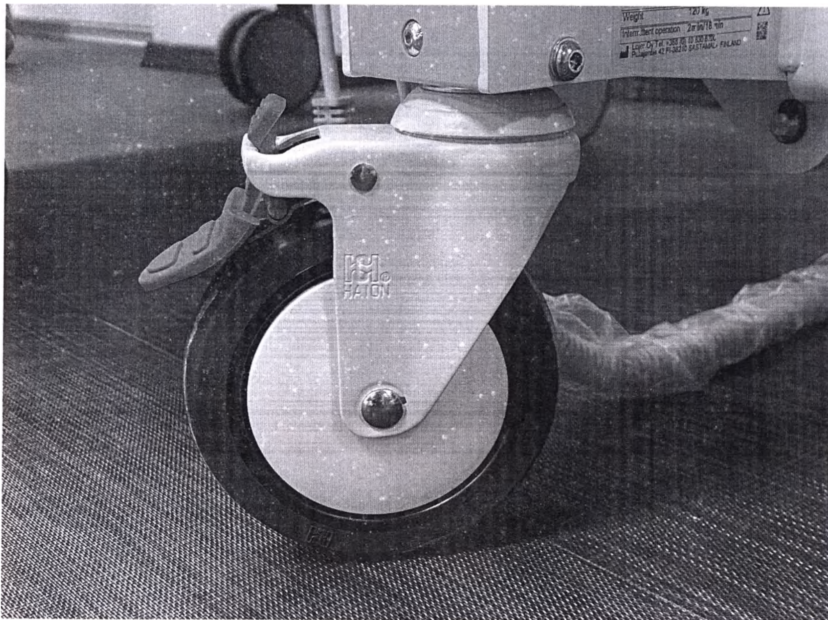
Колесо с индивидуальной блокировкой, диаметром 125 мм
