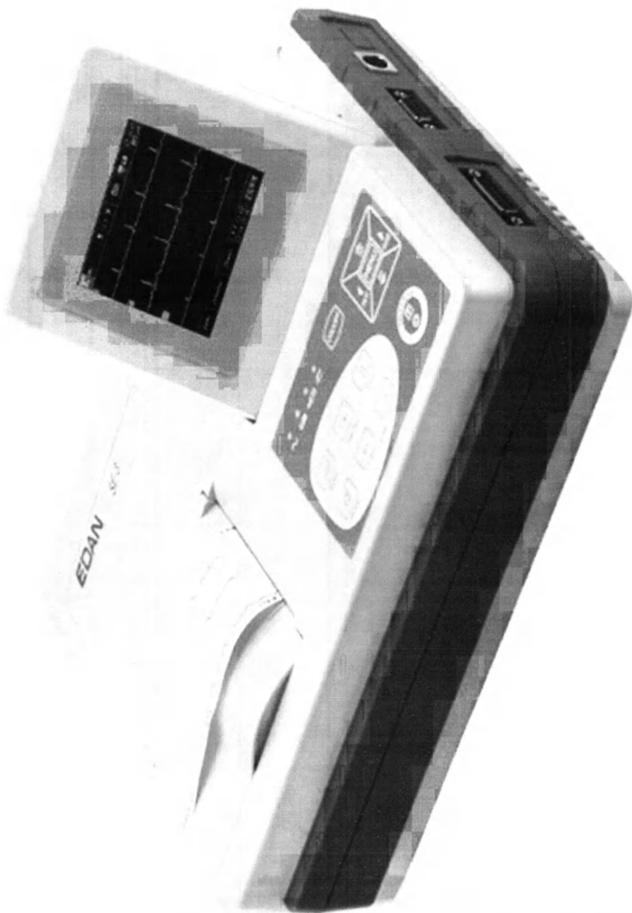
Рис. 5 Блок основной SE-3 (вид спереди; вид сзади аналогичен виду сзади блока основного SE-300B)
