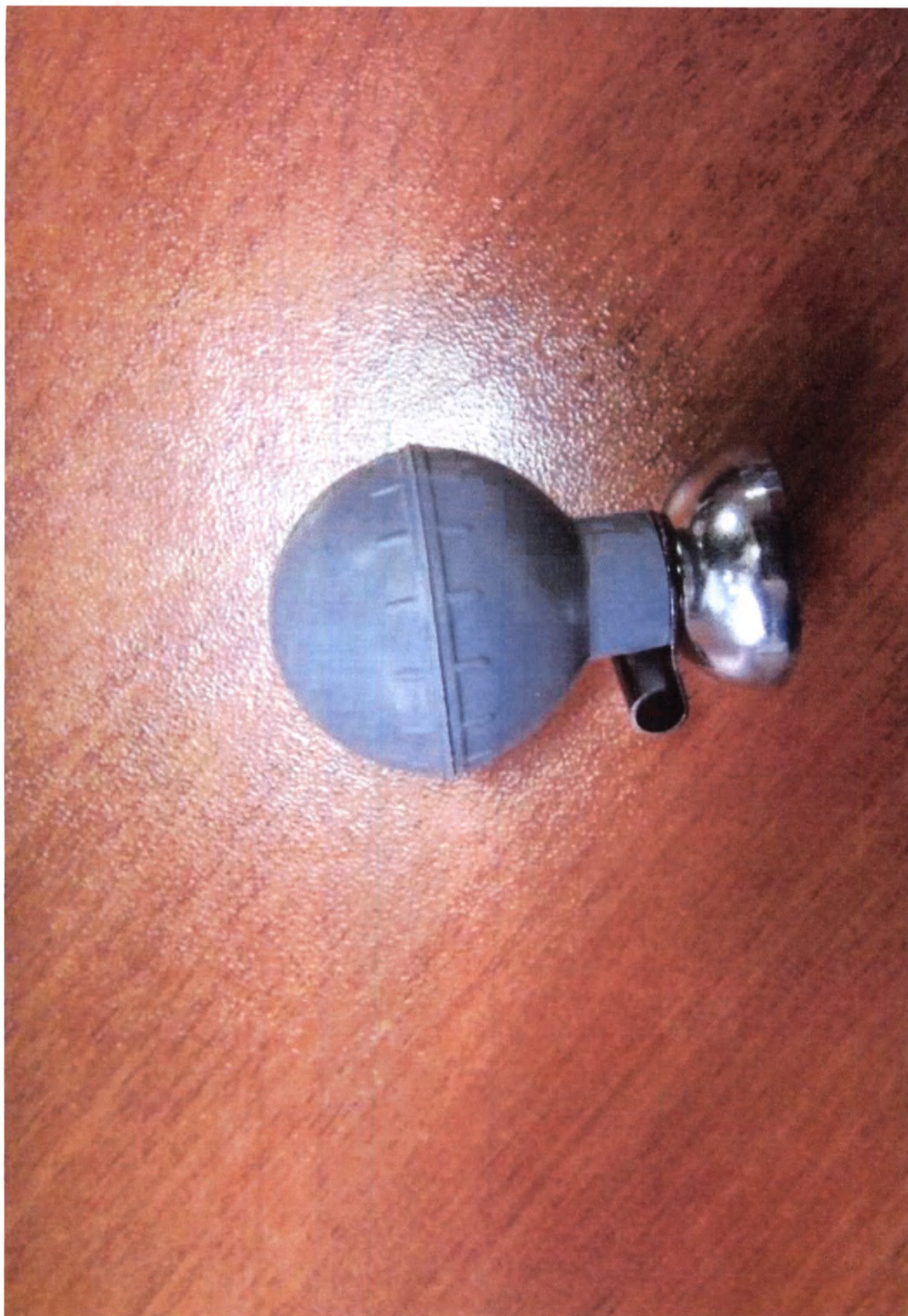
Рис. 14 Электрод-присоска грудной для взрослых (6 шт./уп.)
