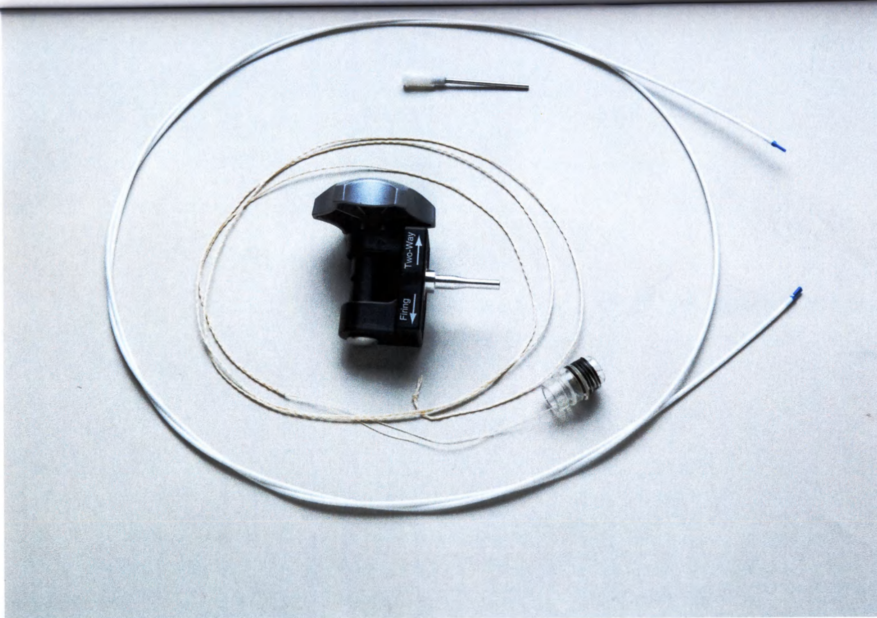
Лигатор шестизарядный Сاعد - MBL-U-6-F
