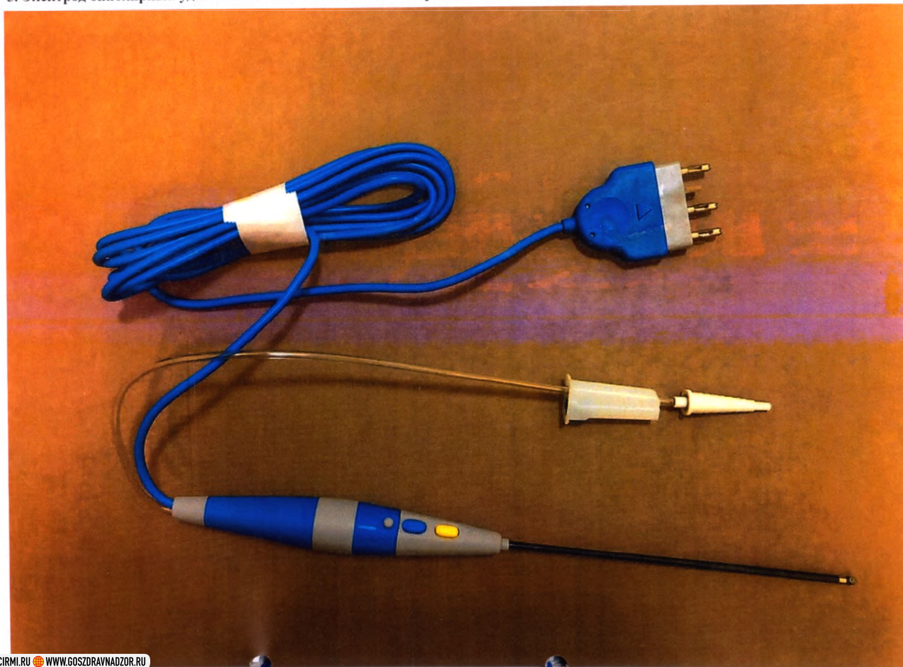
5. Электрод биполярный удлиненный 90° с каналом для аспирации. Изделие вне упаковки.
