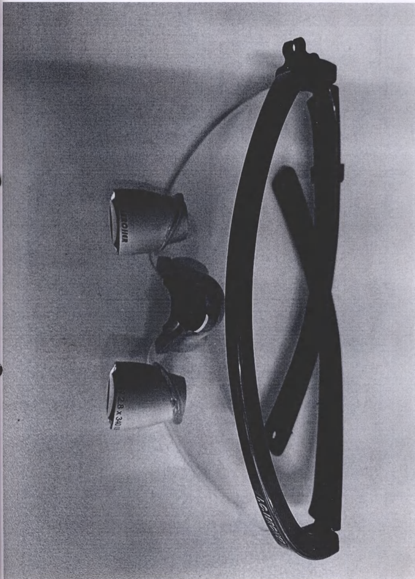
Рисунок 3. Лупа бинокулярная, вариант исполнения: S-View (общий вид)
