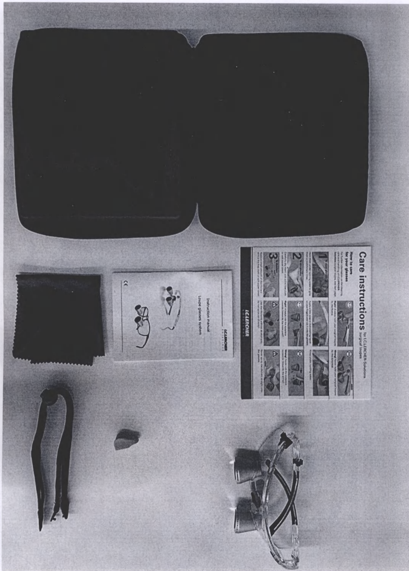
Рисунок 1. Лупа бинокулярная, вариант исполнения: X-View (комплект поставки)
