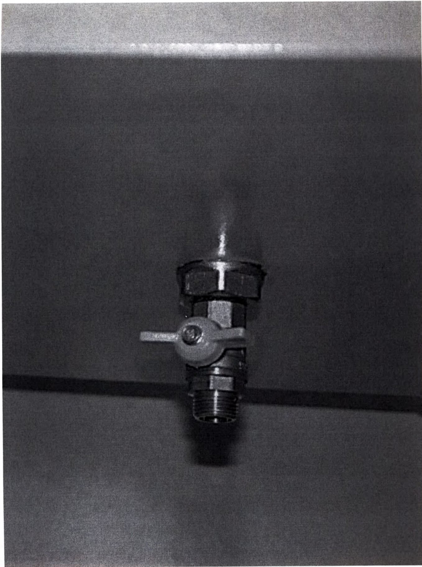
Фотография 4. Дренажный кран для удаления отработанного моющего раствора. («Комплекс моющее - дезинфицирующий медицинский КМД-24-«Я-ФП», ТУ 9451-024-55307168-2013)
