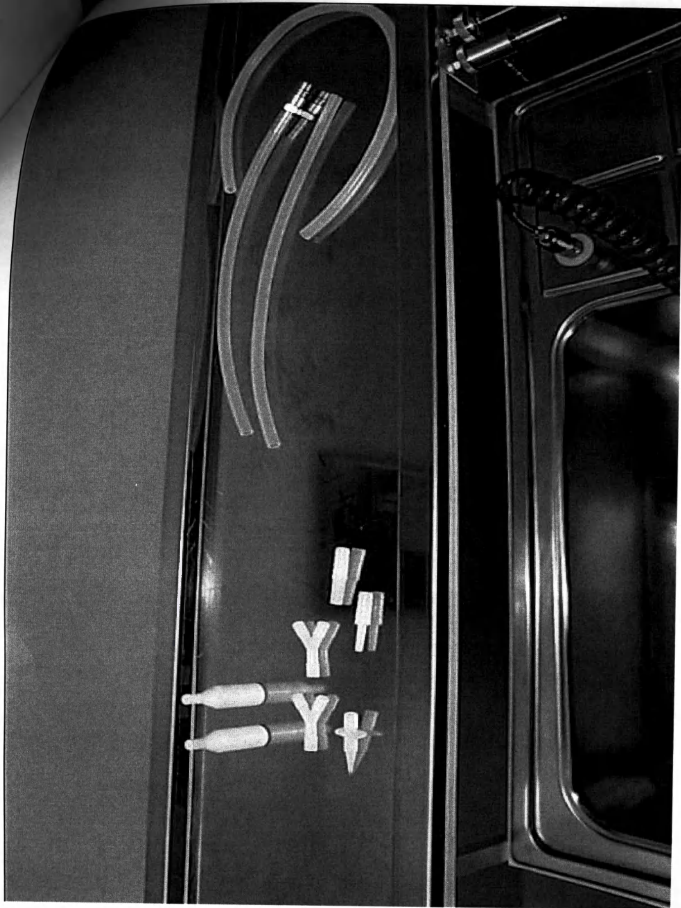
Фотография 6. Комплект приспособлений для очистки эндоскопов (состоит из полимерных переходников, наконечников различного диаметра и шлангов силиконовых) («Комплекс моюще - дезинфицирующий медицинский КМД-24-«Я-ФП», ТУ 9451-024-55307168-2013)
