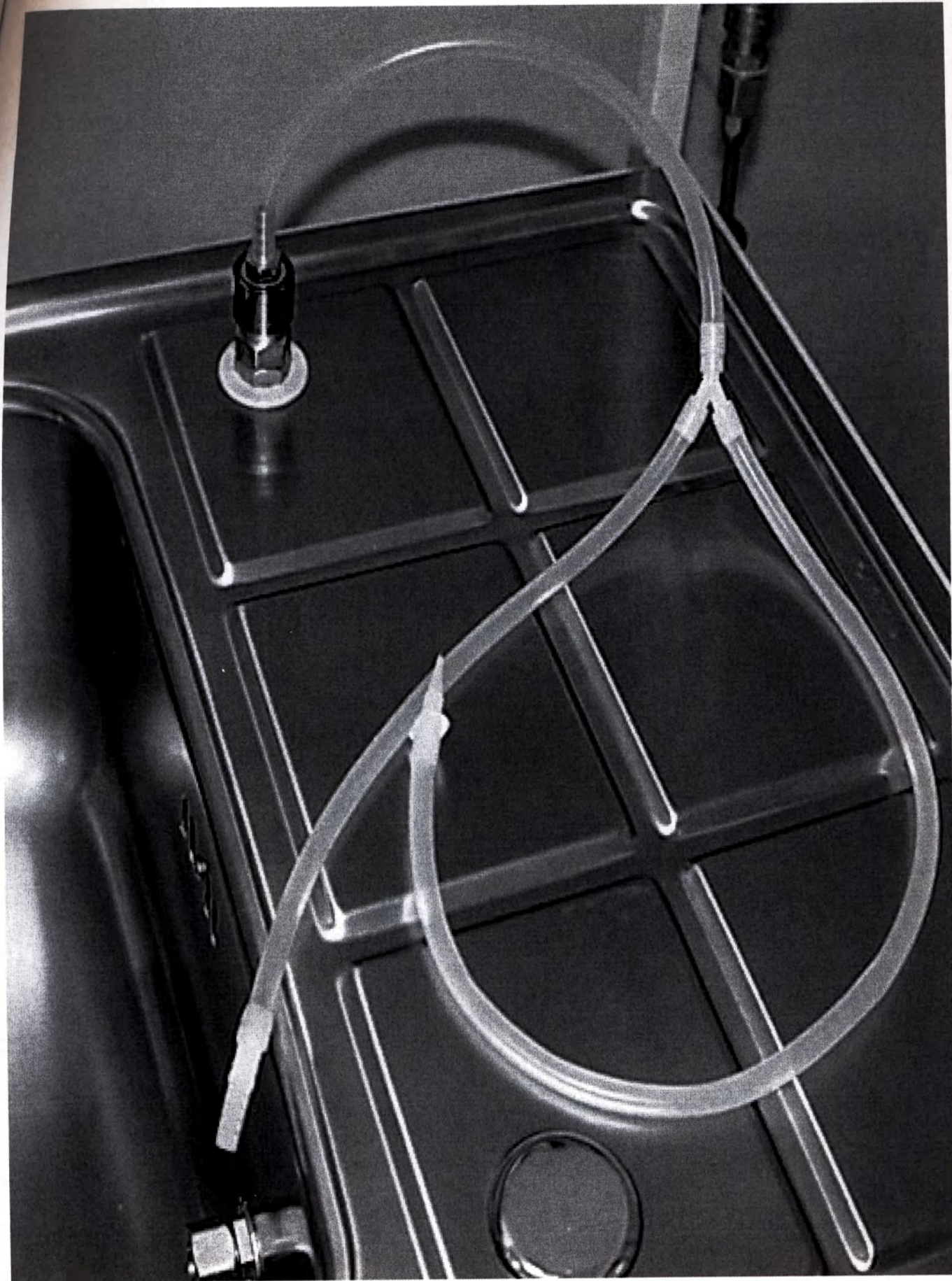
Фотография 5. Быстросъемное соединение для подключения комплектов по очистке с Y – образным соединительным переходником. («Комплекс моюще-дезинфицирующий медицинский КМД-24-«Я-ФП», ТУ 9451-024-55307168-2013)
