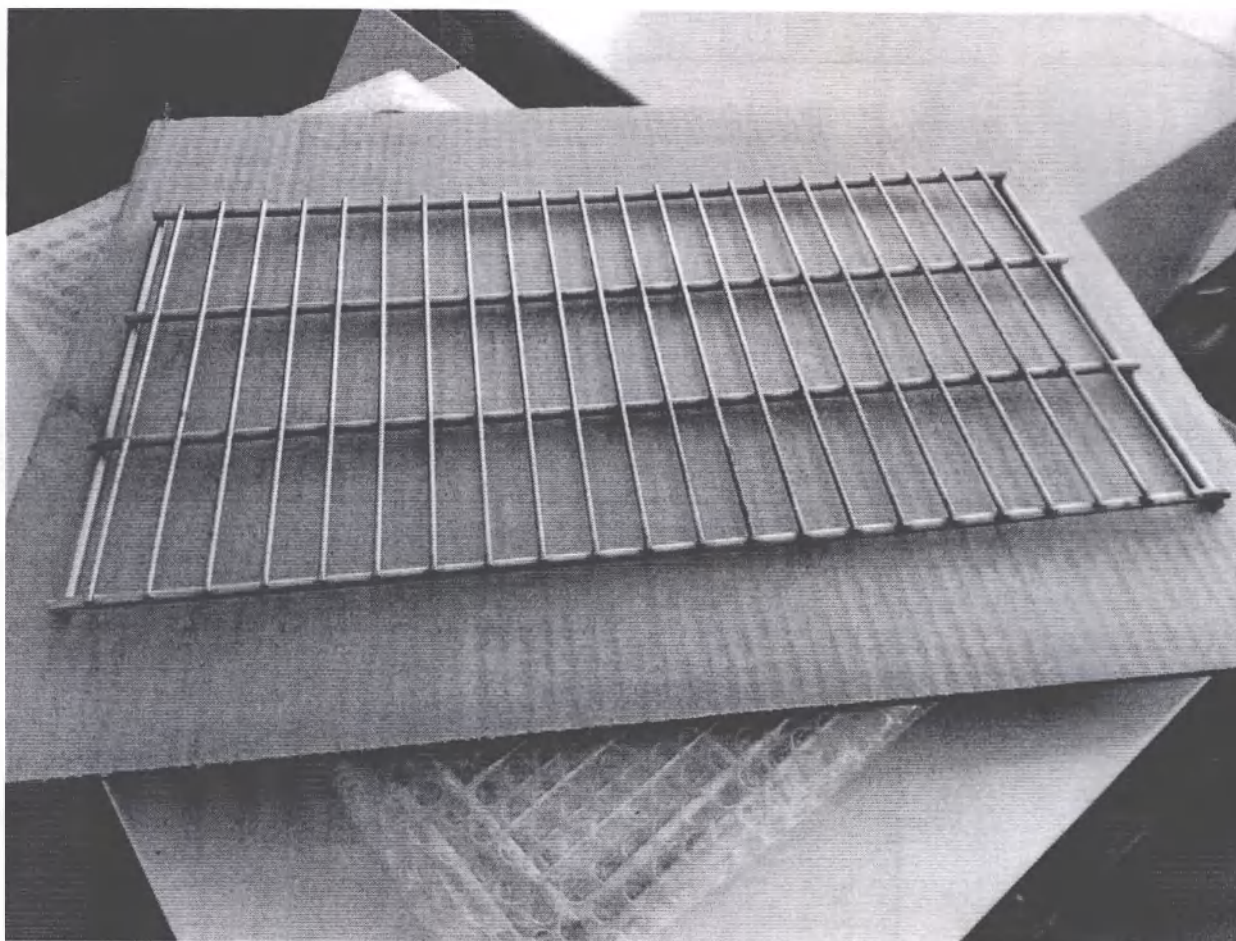
Фотографическое изображение 16. Кассета КИУС.321546.036.
