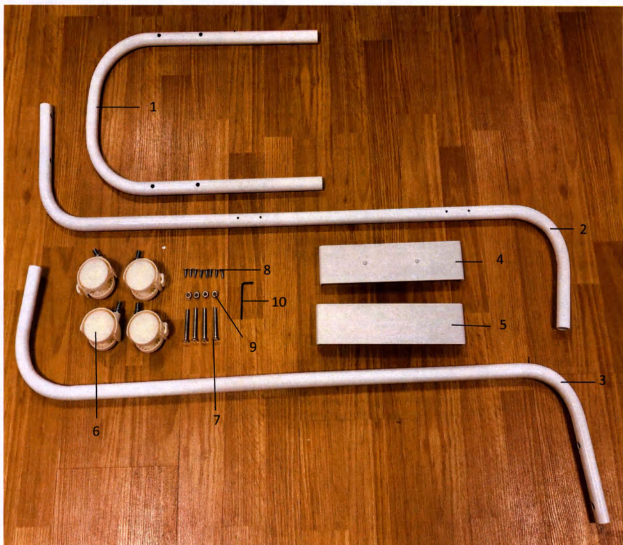
Стойка передвижная СП 2 (комплект поставки)
