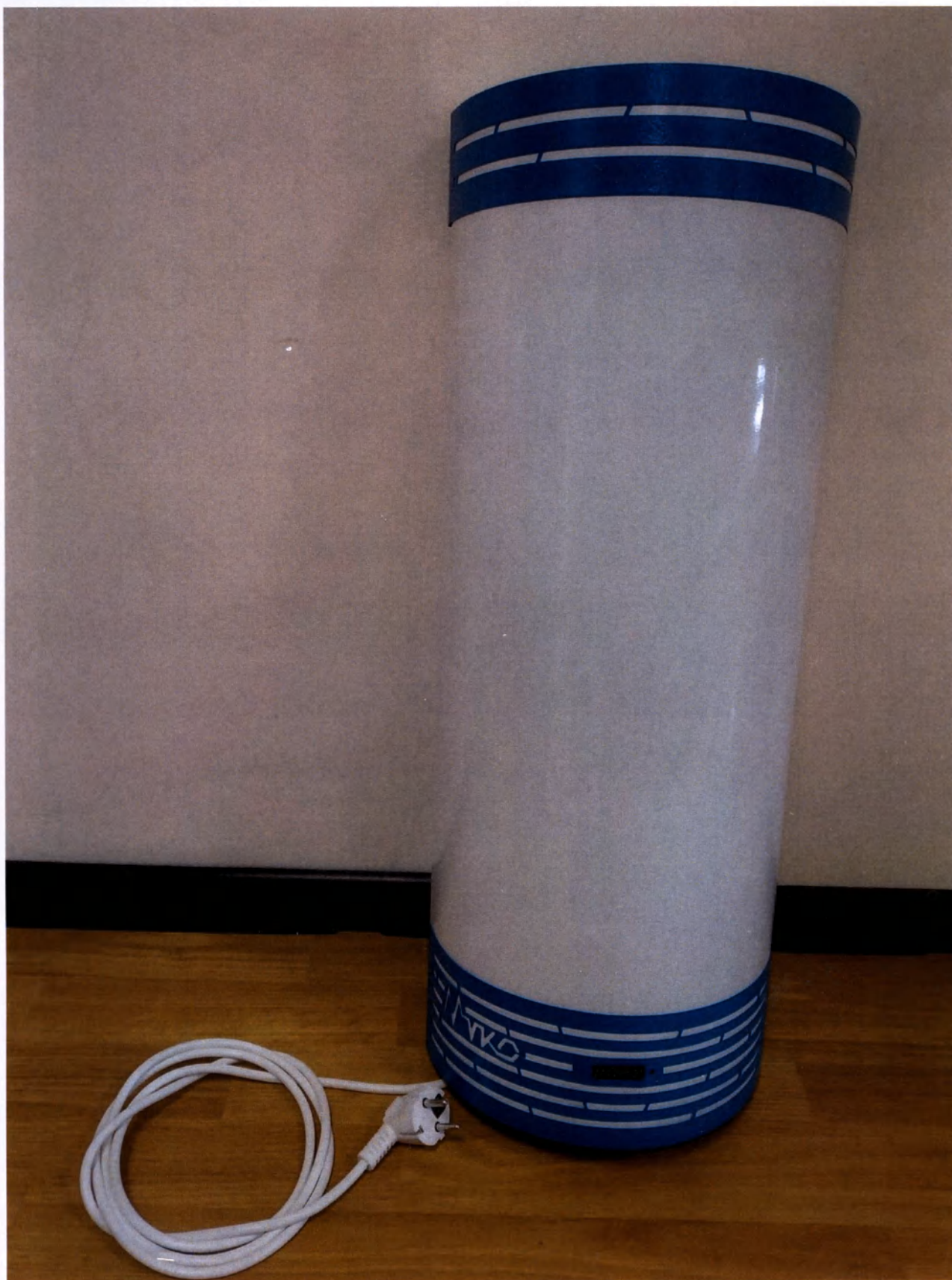
Общий вид Облучатель-рециркулятор бактерицидный для обеззараживания воздуха помещений ОБР 15/2- «Мед ТеКо»
