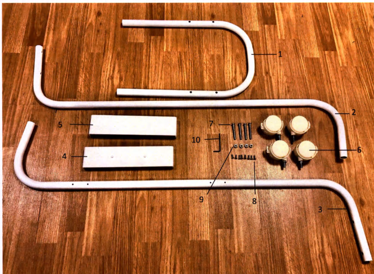
Стойка передвижная СП 1 (комплект поставки)
