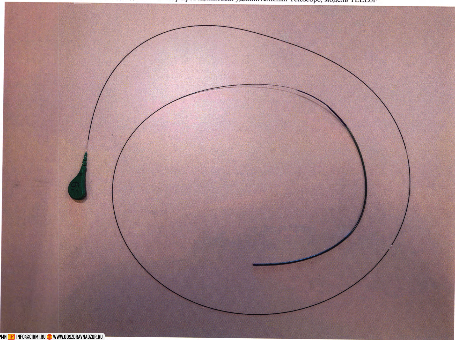
Внешний вид изделия: Катетер проводниковый удлинительный Telescope, модель TELE6F
