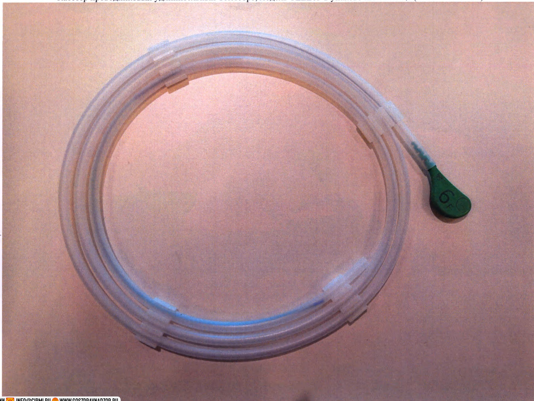
Катетер проводниковый удлинительный Telescope, модель TELE6F в упаковочном кольце (включая клипсы)
