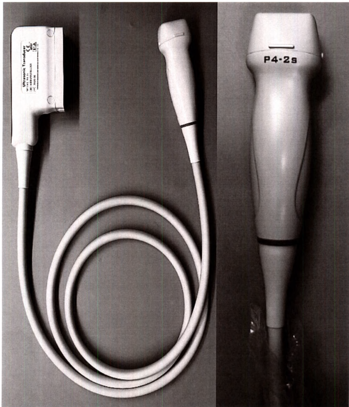
Датчик ультразвуковой секторный фазированный P4-2s
