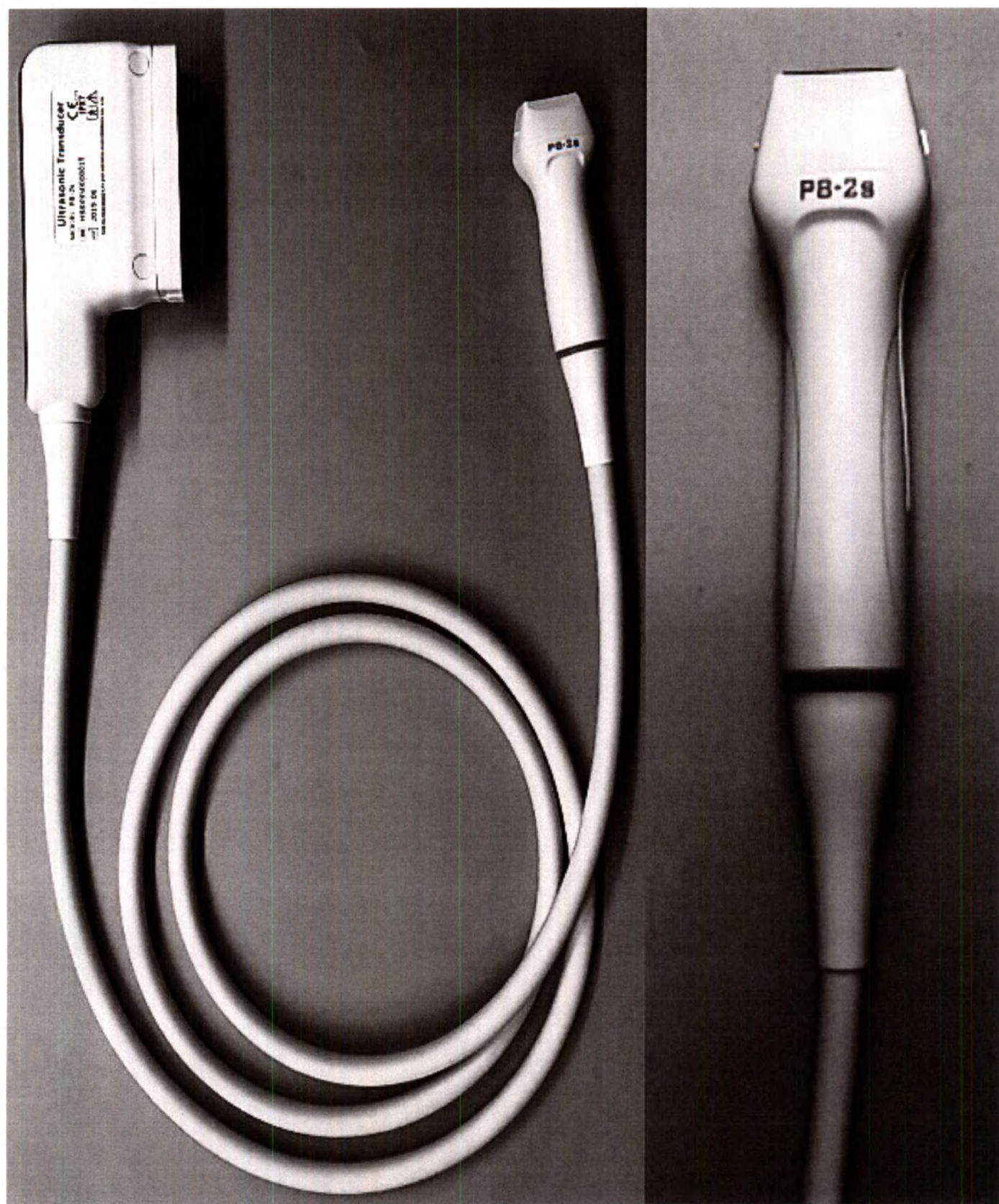
Датчик ультразвуковой секторный фазированный P8-2s
