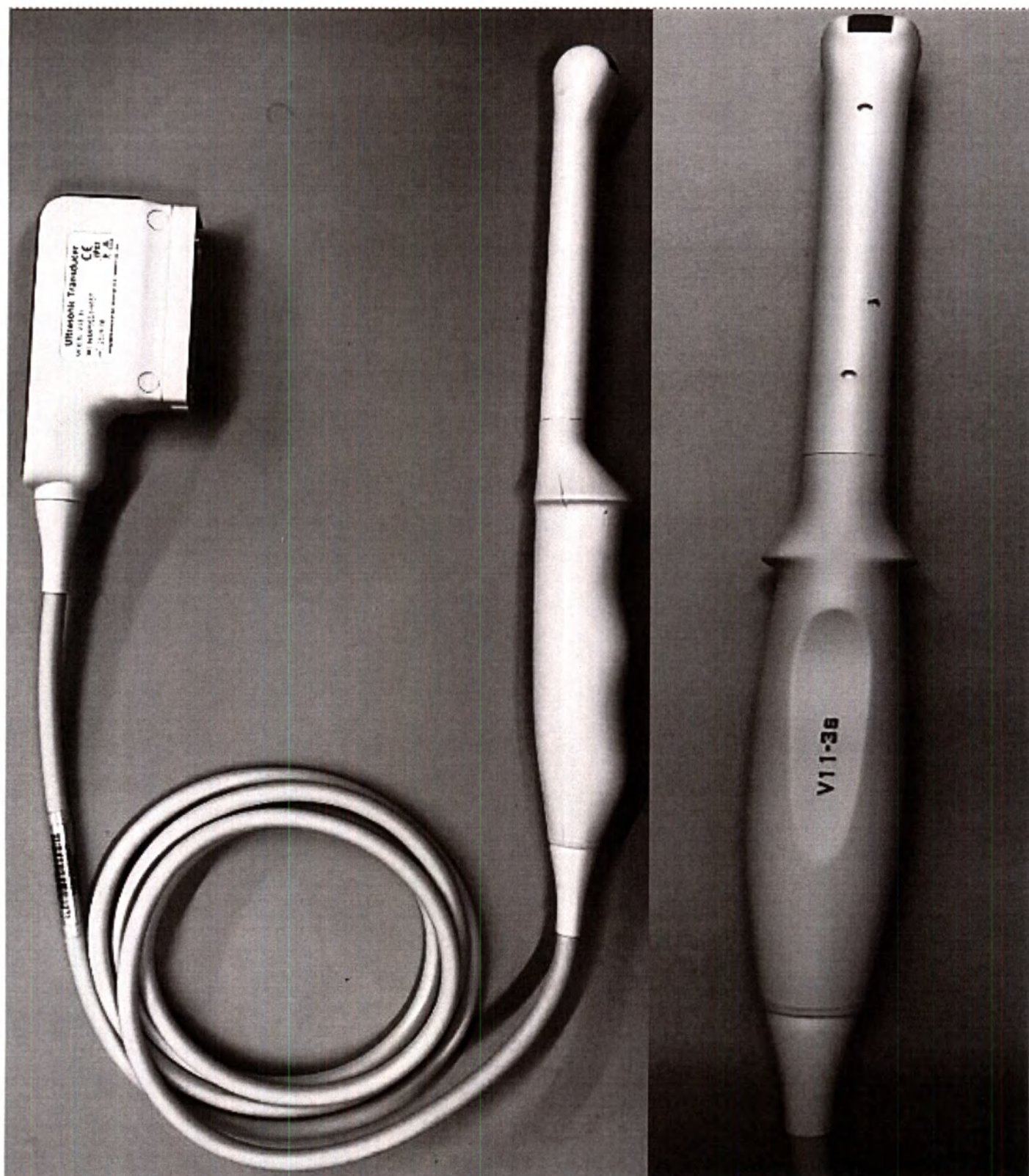
Датчик ультразвуковой внутриполостной V11-3s
