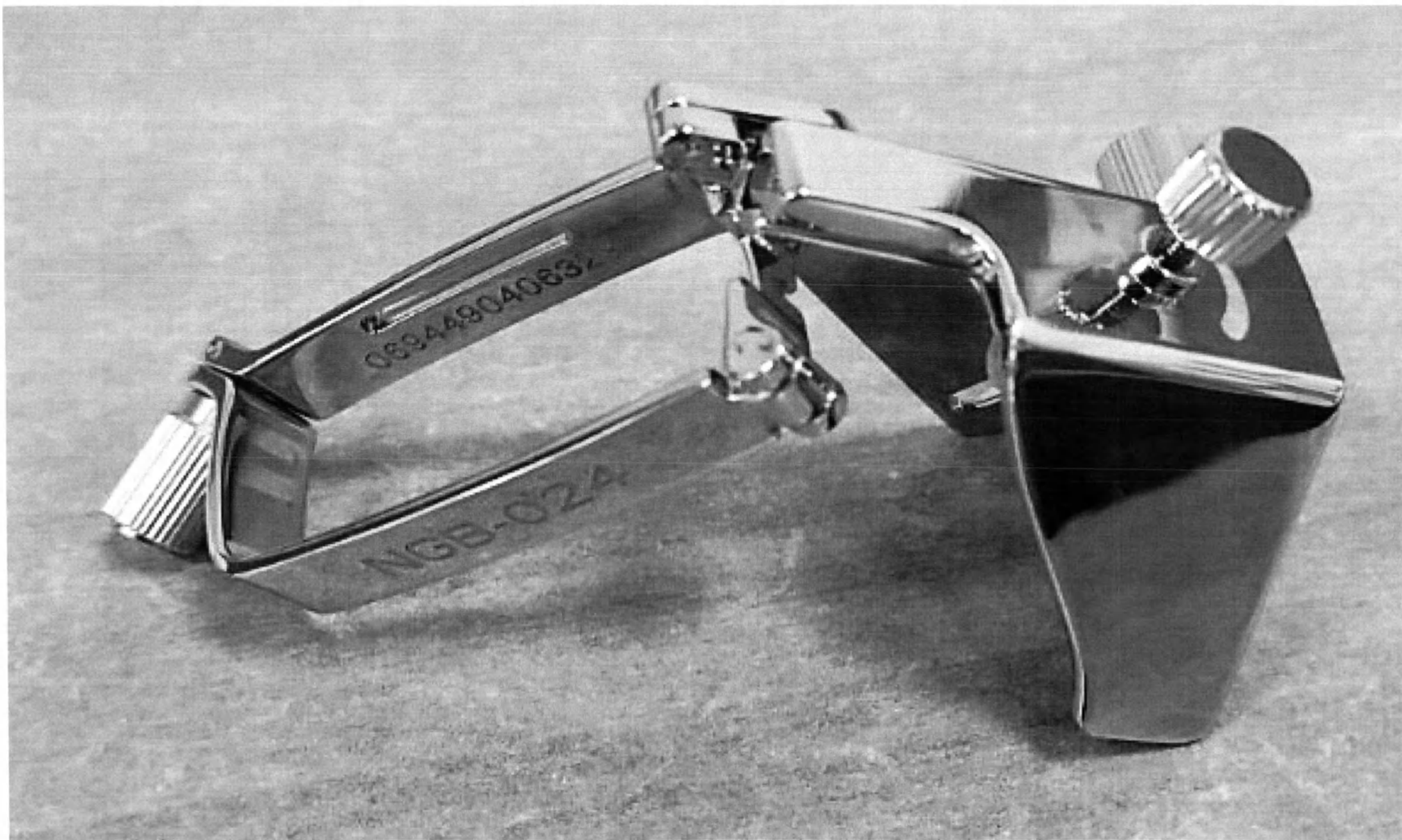
Насадка биопсийная металлическая, со съемной направляющей для игл NGB-024
