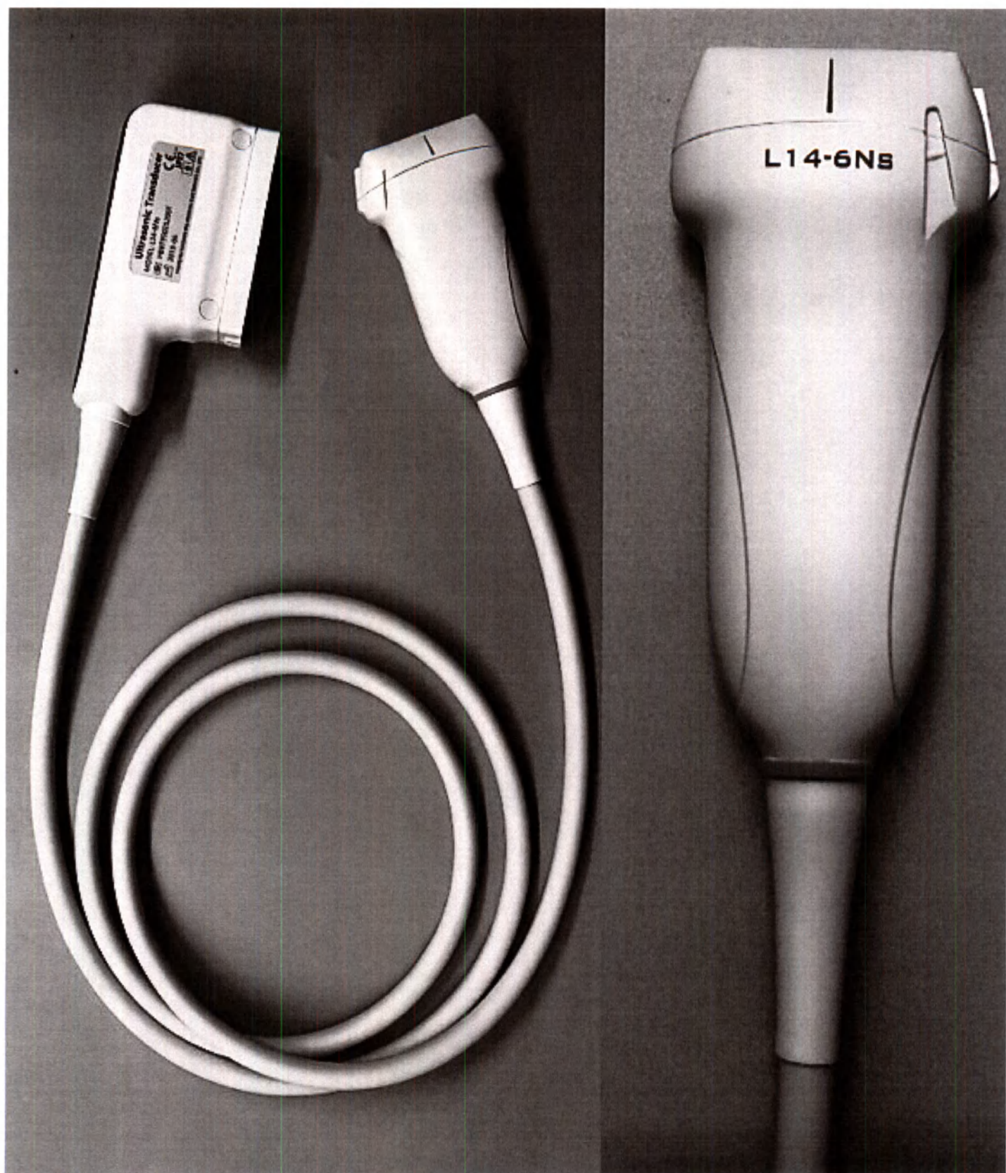
Датчик ультразвуковой линейный L14-6Ns
