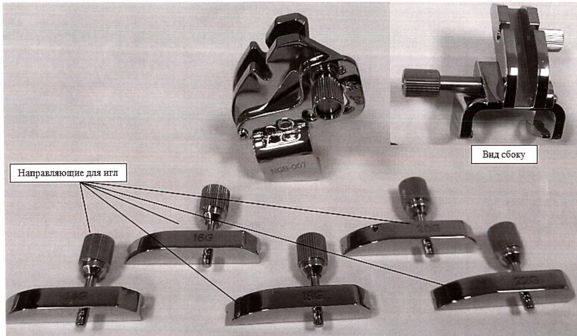
Насадка биопсийная металлическая, со съемной направляющей для игл NGB-007
