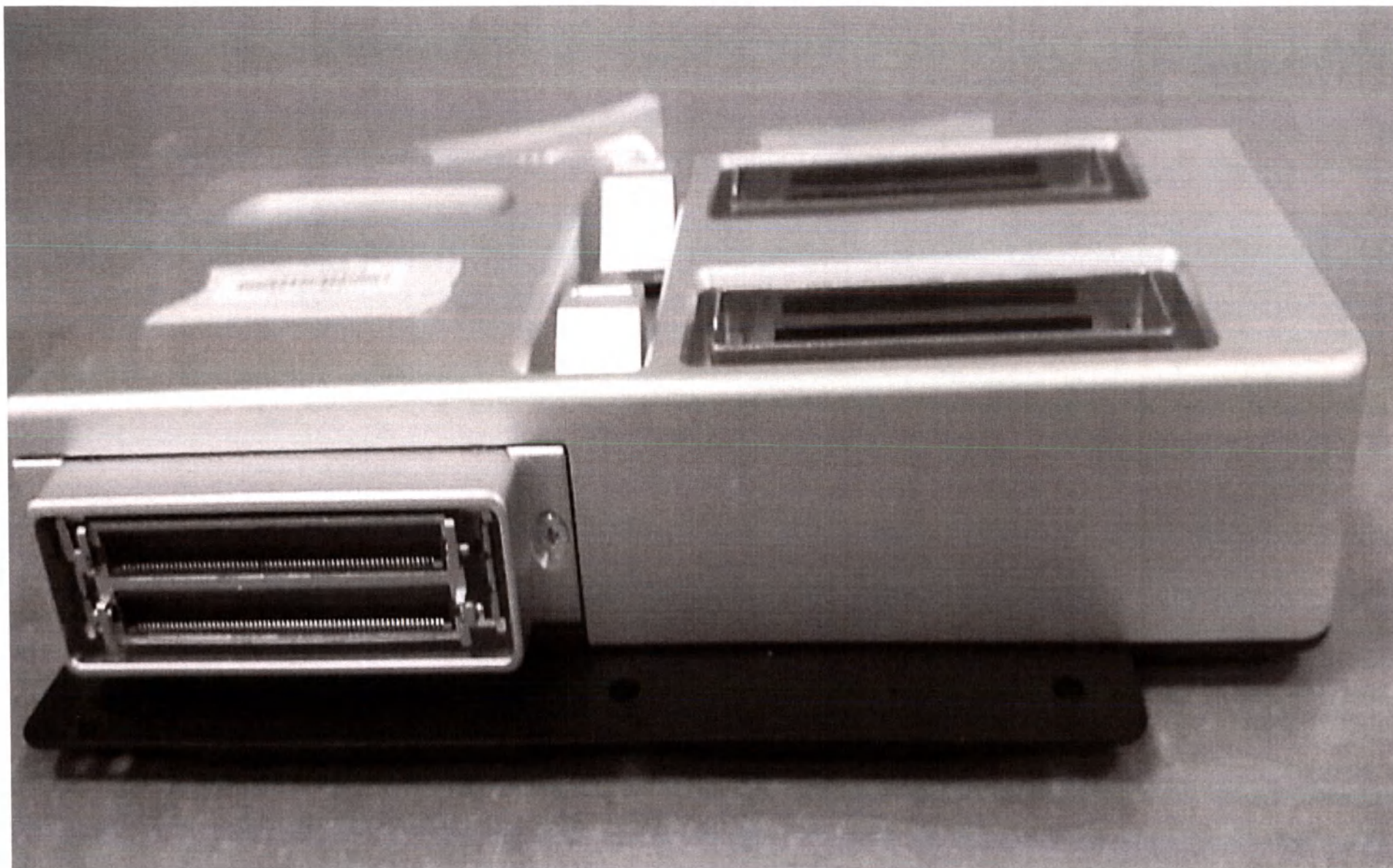
Модуль-разветвитель на два порта для подключения датчиков. Вид сбоку
