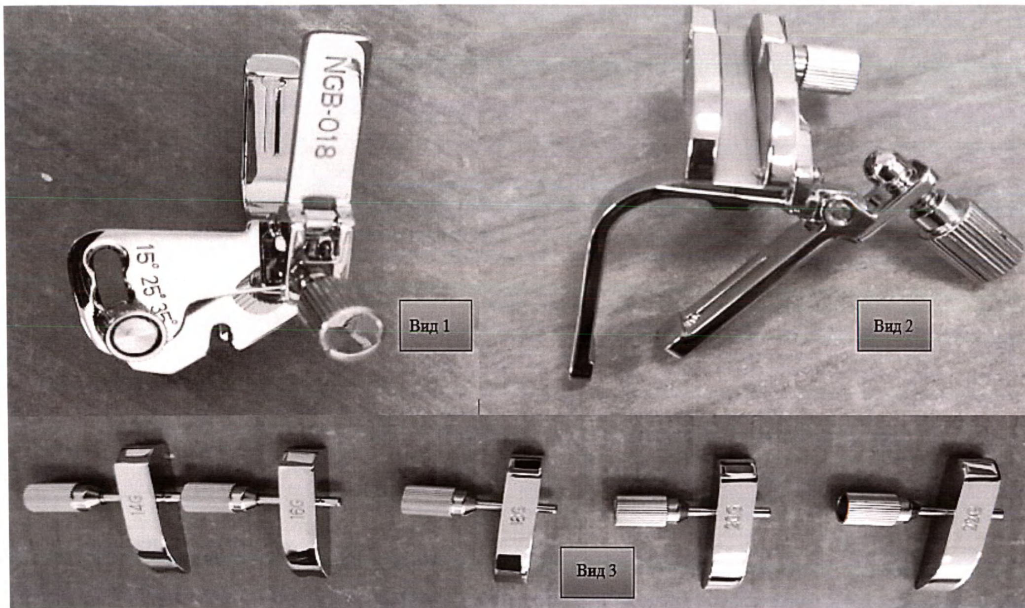
Насадка биопсийная металлическая, со съемной направляющей для игл NGB-018
