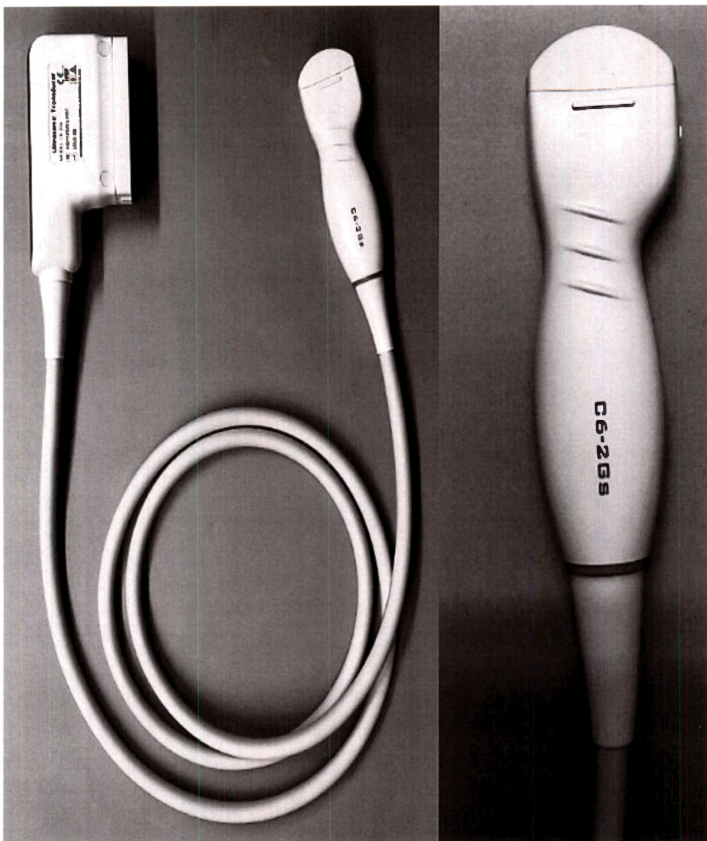
Датчик ультразвуковой конвексный C6-2Gs
