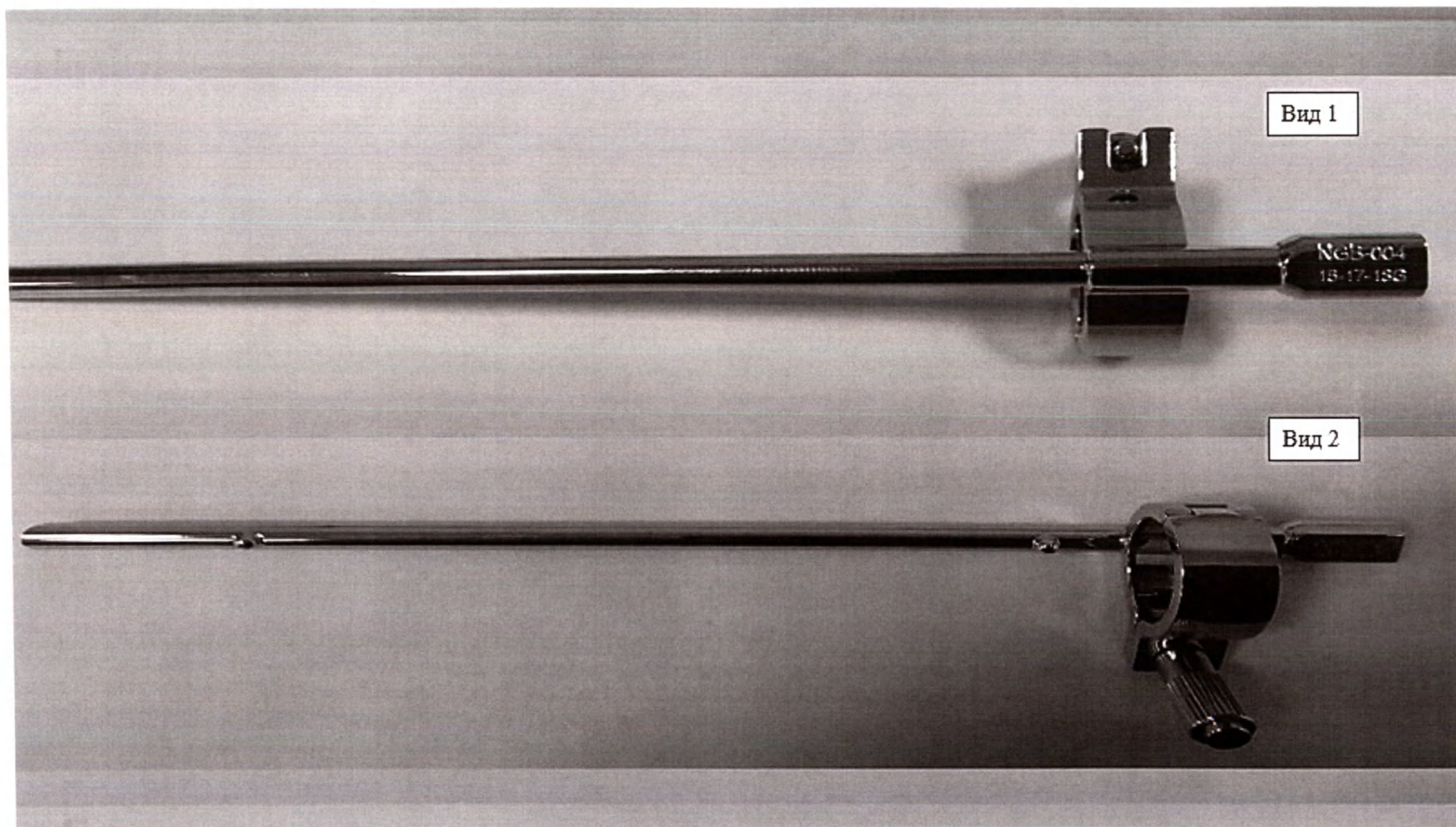
Насадка биопсийная металлическая, с несъемной направляющей для игл NGB-004
