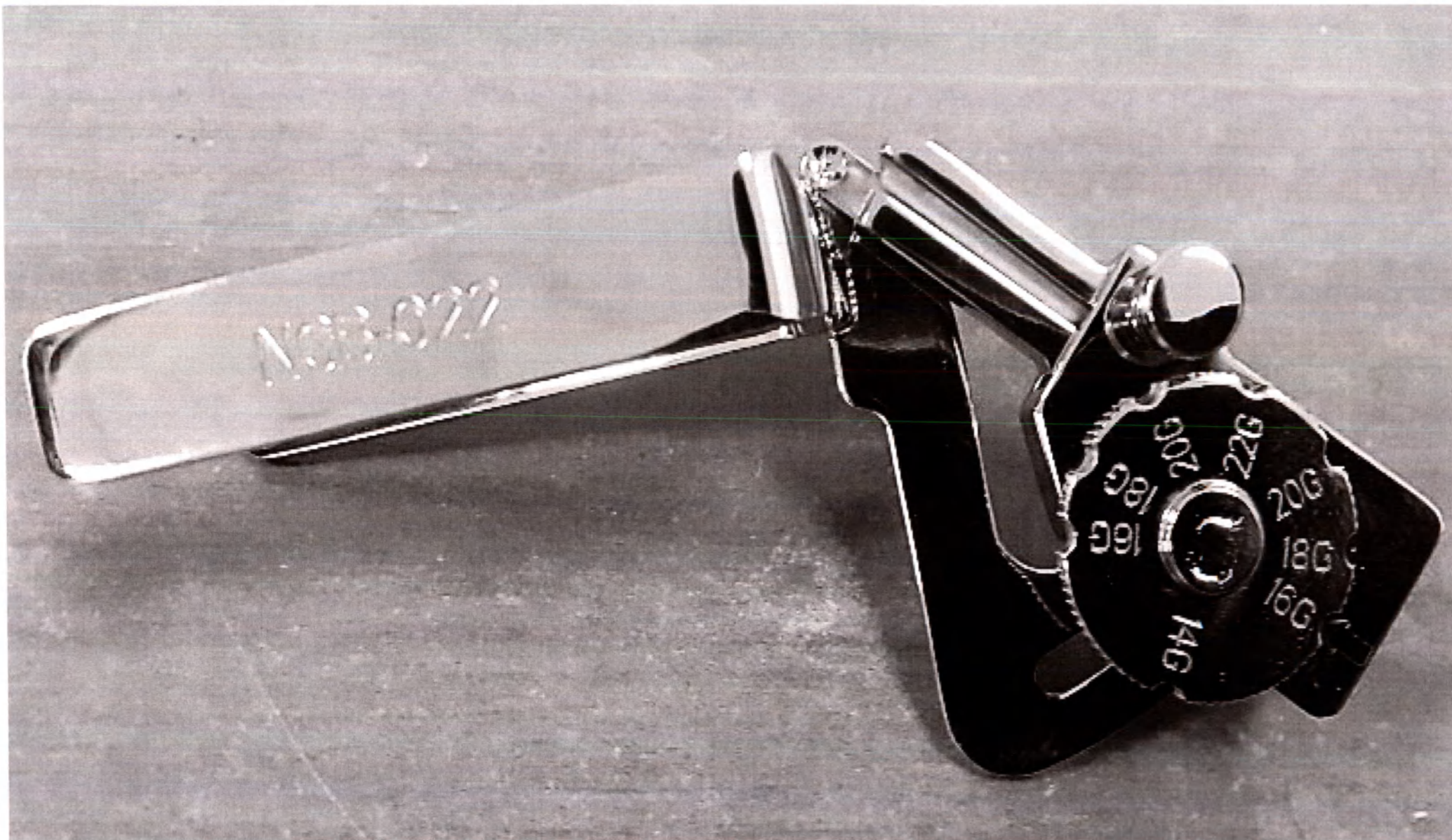
Насадка биопсийная металлическая, со съемной направляющей для игл NGB-022
