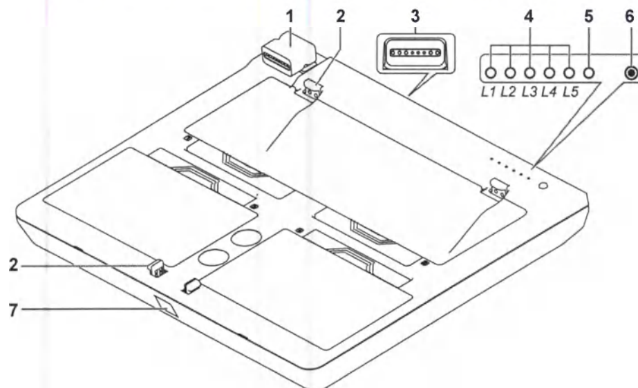
Рис. 2-3 Комплект аккумуляторов встраиваемых (U-Bank)
