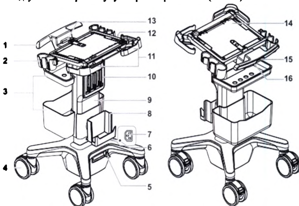
Рис. 13 Тележка мобильная МТЗ
