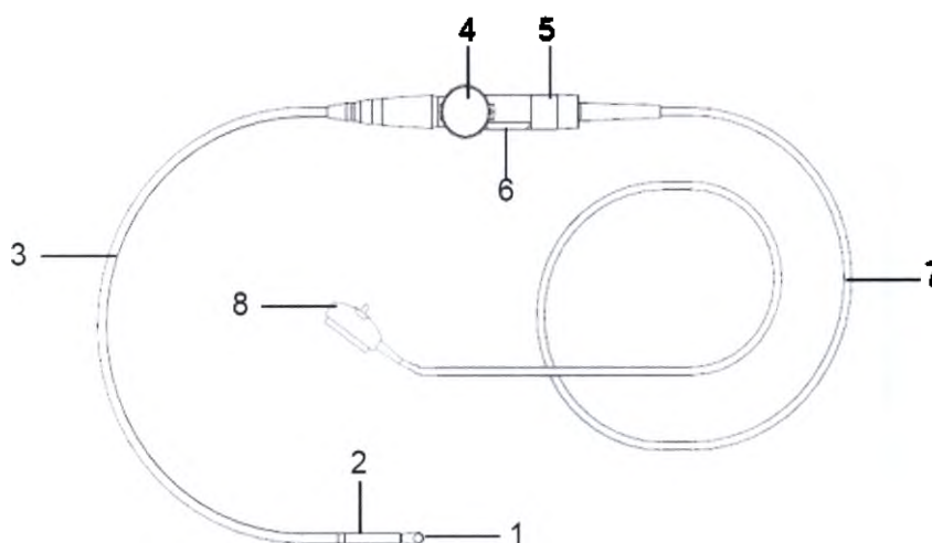
Устройство датчика ультразвукового секторного фазированного чреспищеводного P7-3Ts
