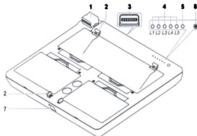
Рис.8 Комплект аккумуляторов встраиваемых (U-Bank)
