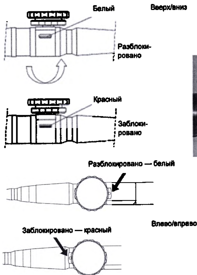
Рис. J-5 Кнопки для фиксации, датчик P8-3Ts
