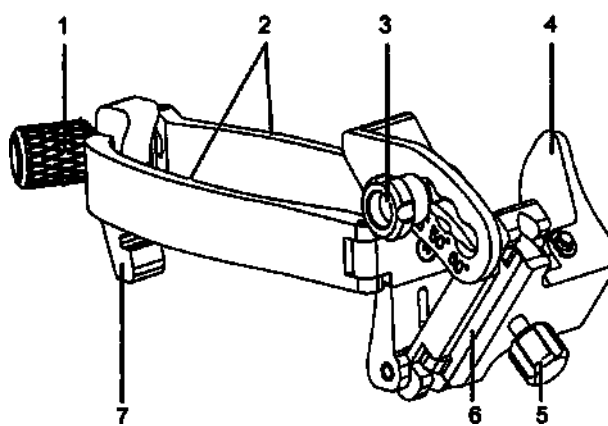
Насадка биопсийная металлическая, со съемной направляющей для игл NGB-053
