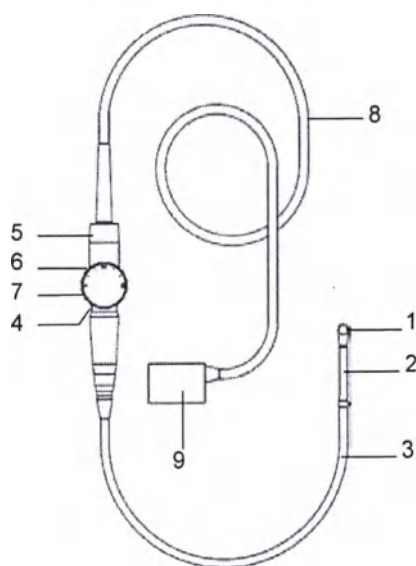
Рис. J-2 Функции каждого компонента педиатрического датчика ультразвукового секторного фазированного чрепшесоводного
