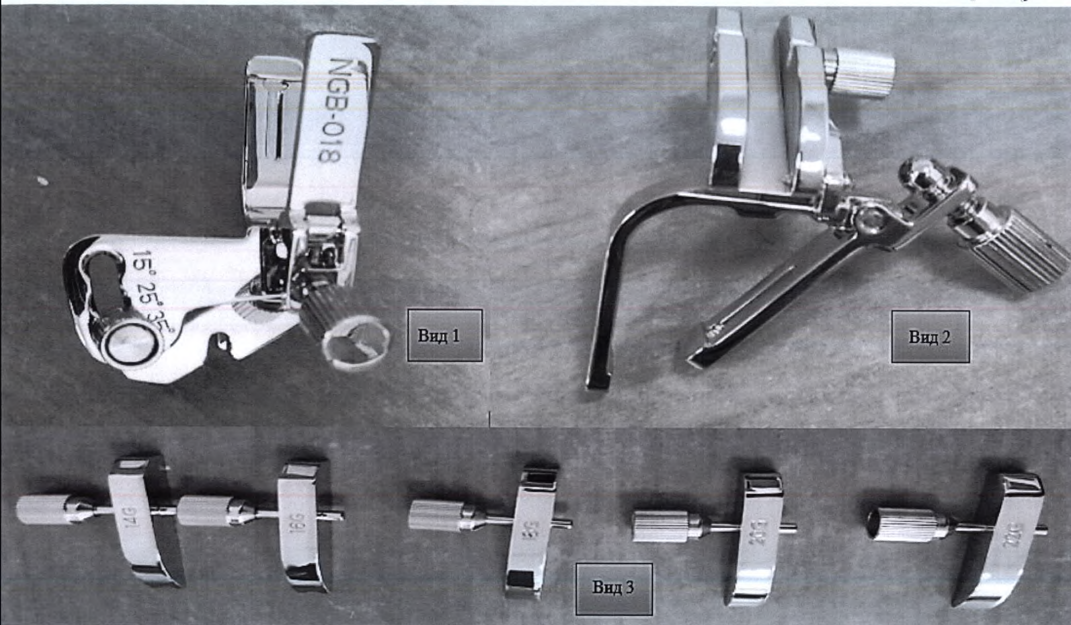
Насадка биопсийная металлическая, со съемной направляющей для игл NGB-018
