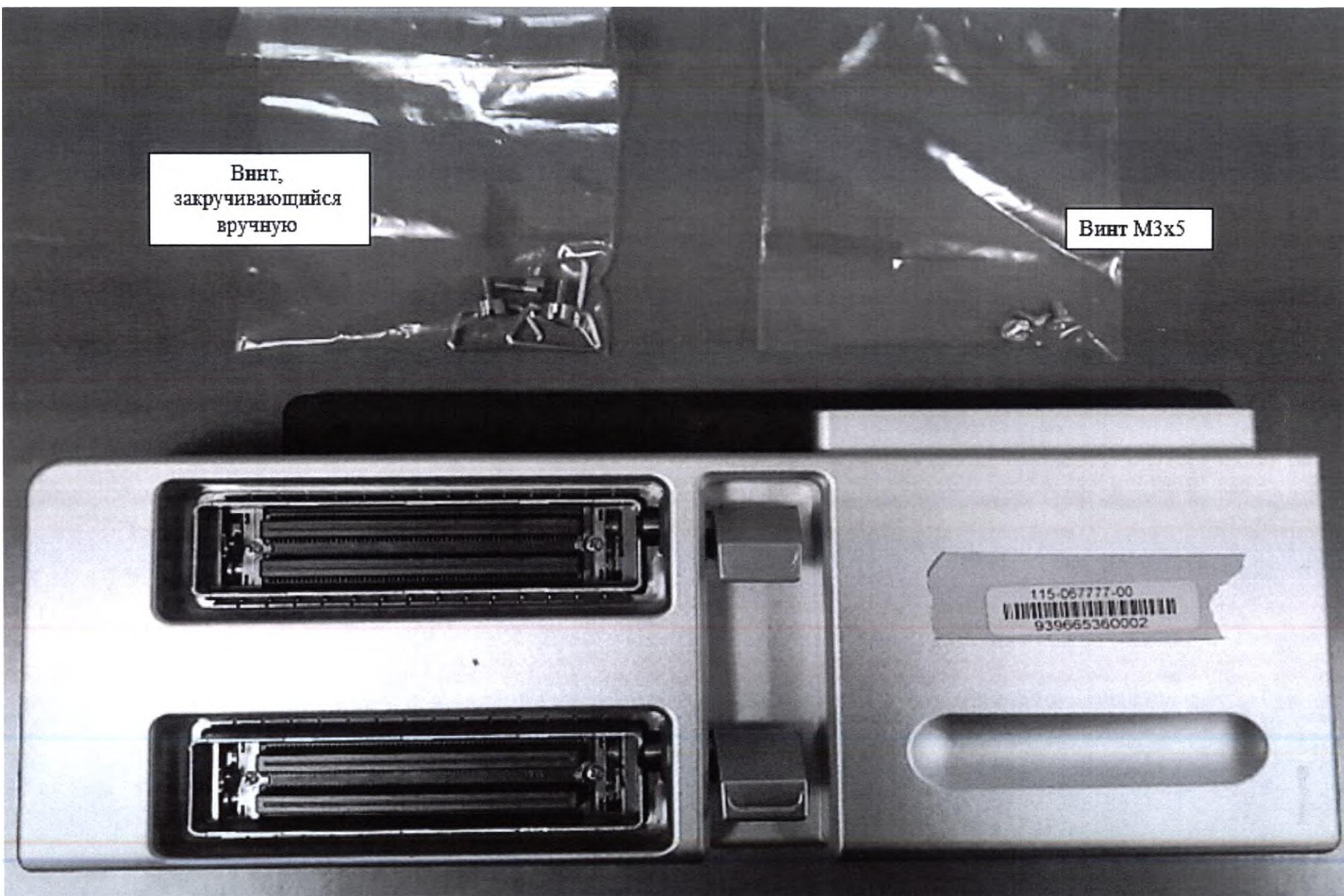
Модуль-разветвитель на два порта для подключения датчиков
