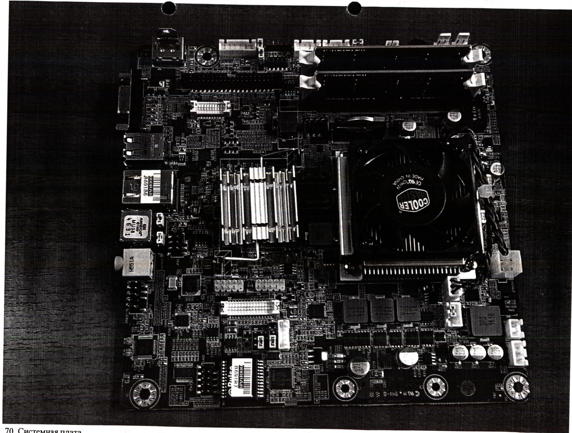
70. Системная плата.
