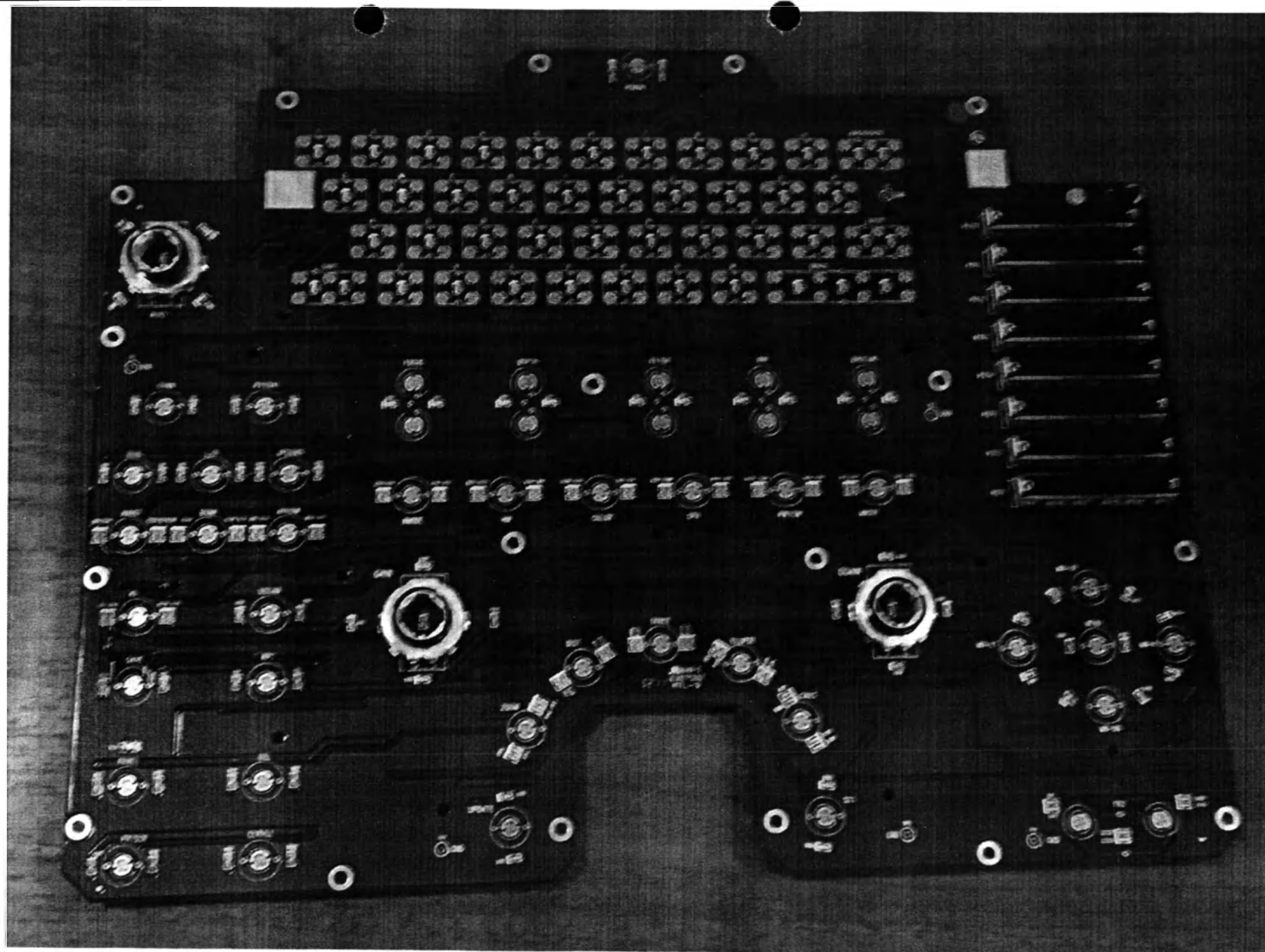
72. Панель управления.
