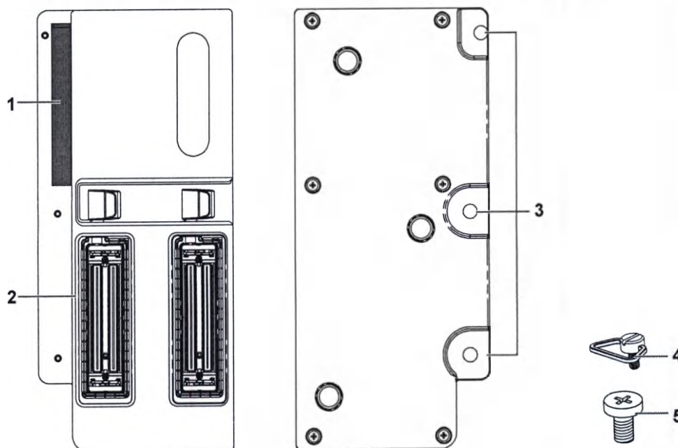
Рис. 2-2 Модуль-разветвитель на два порта для подключения датчиков
