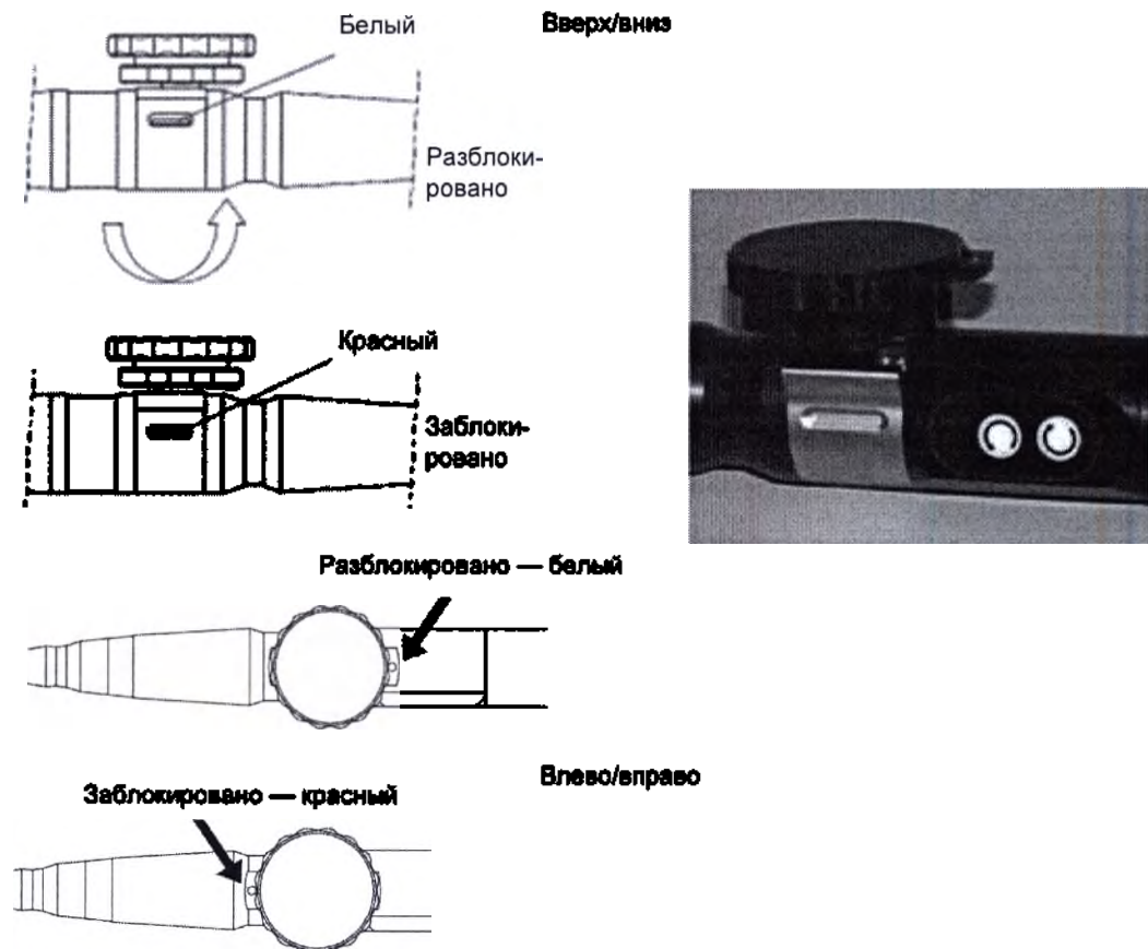
Рис. J-5 Кнопки для фиксации, датчик Р8-3Ts
