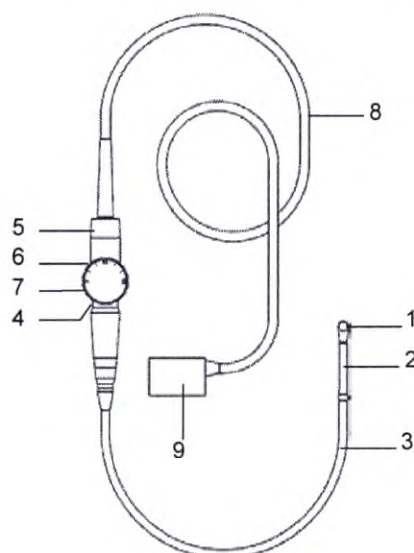
Рис. J-2 Функции каждого компонента педиатрического датчика ультразвукового секторного фазированного чреспищеводного
