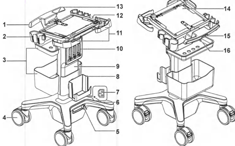
Рис. В-1 Обзор тележки
