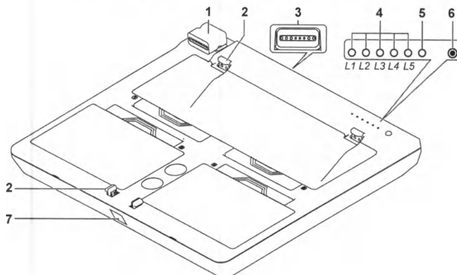
Рис. 2-3 Комплект аккумуляторов встраиваемых (U-Bank)
