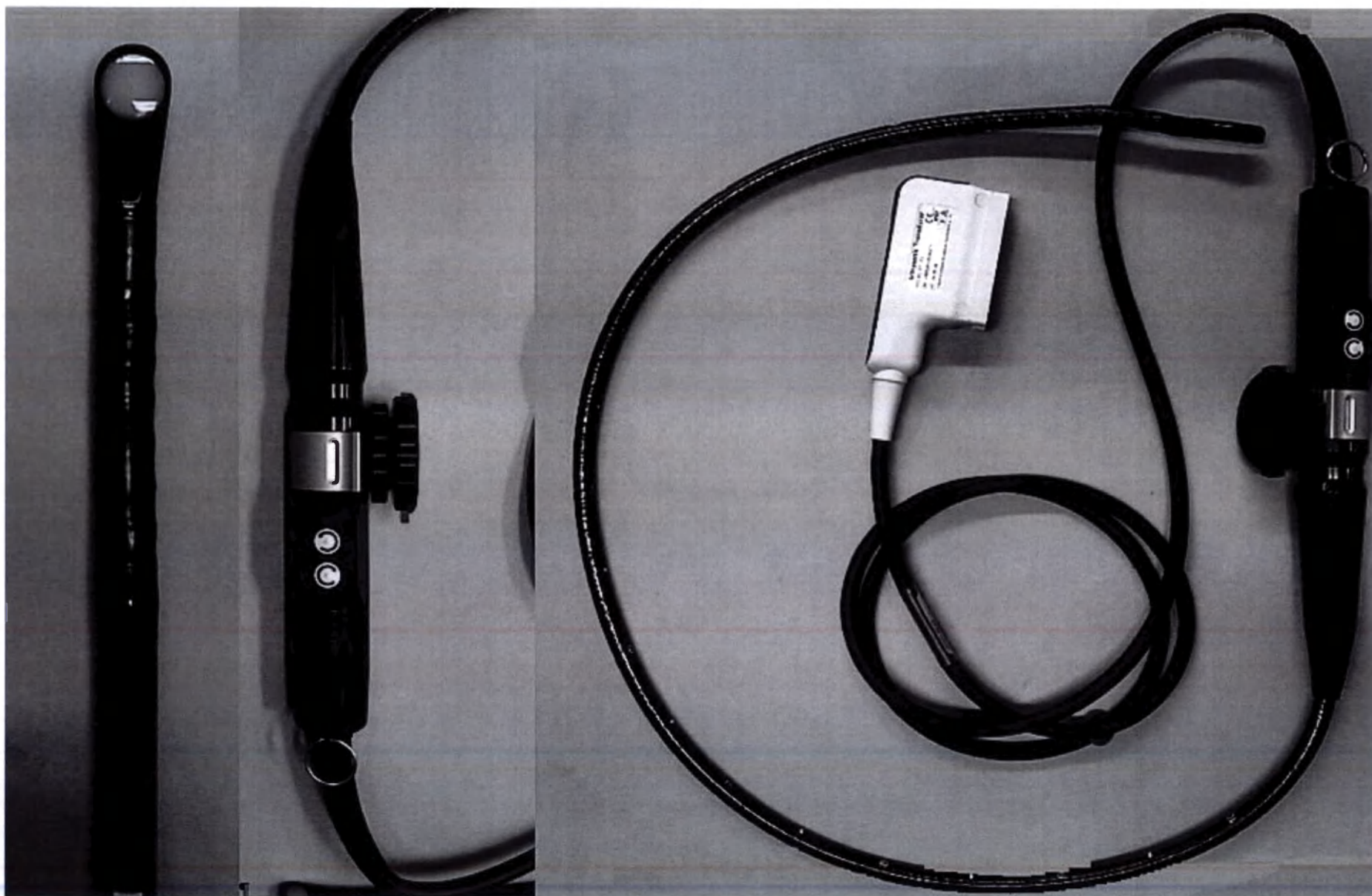
Датчик ультразвуковой секторный фазированный чреспищеводный Р7-3Тс
