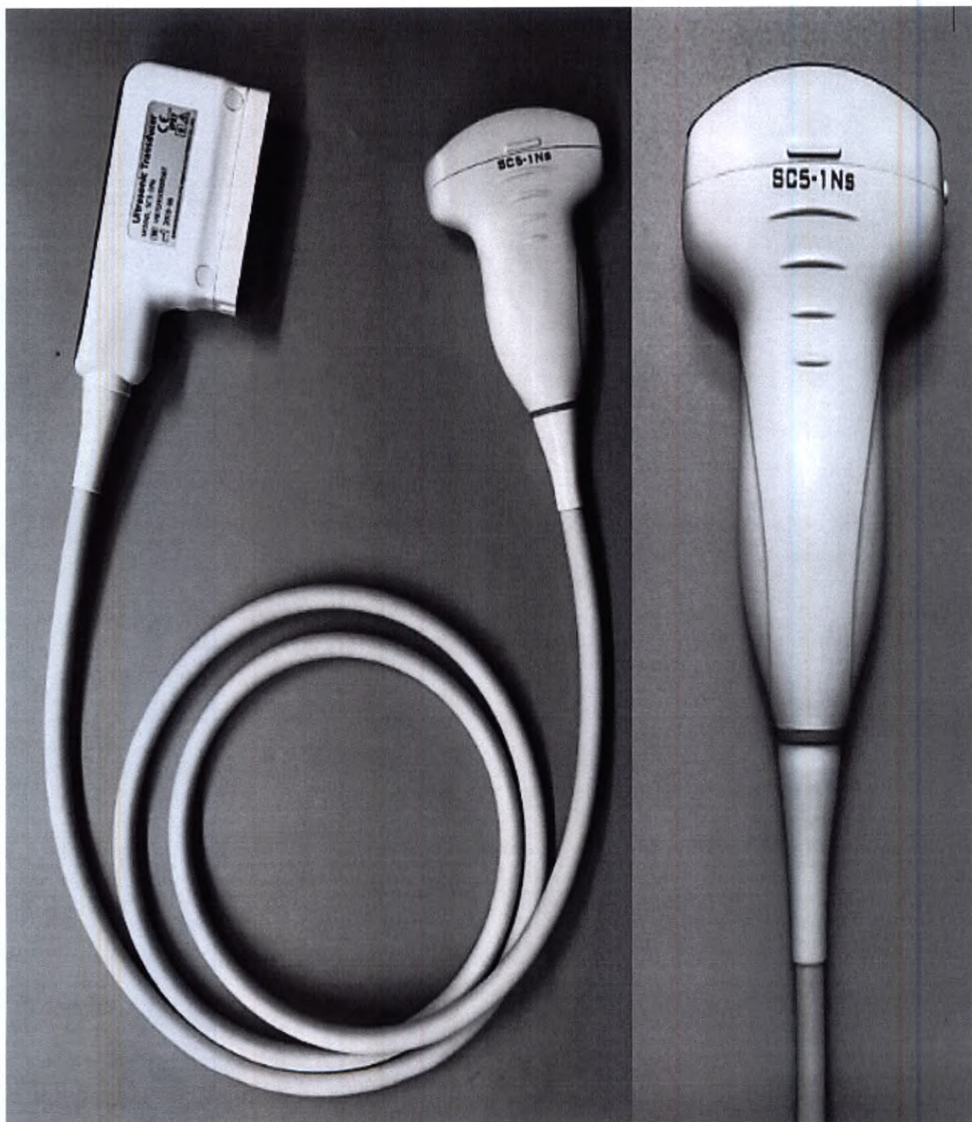
Датчик ультразвуковой секторный фазированный Р10-4s
