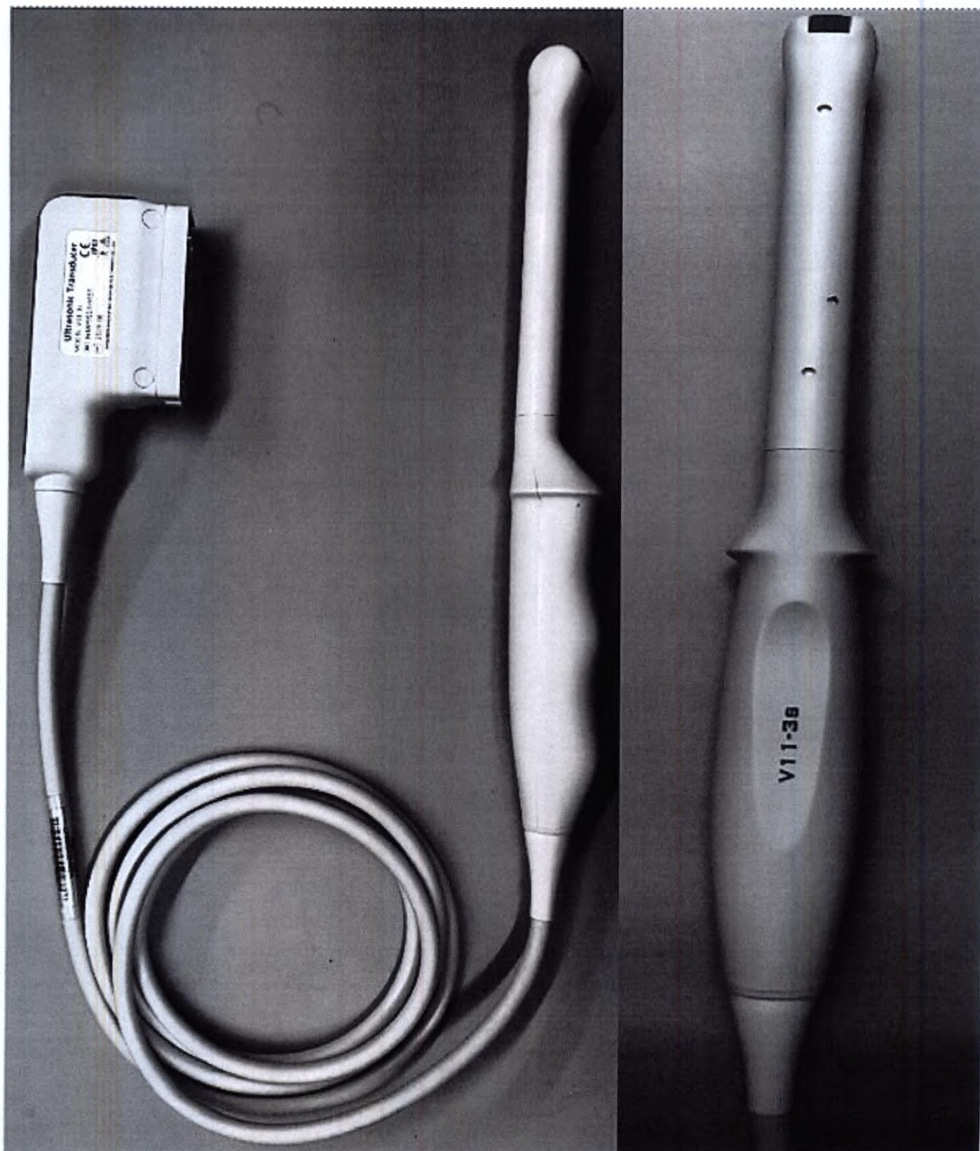
Датчик ультразвуковой внутриполостной V11-3s
