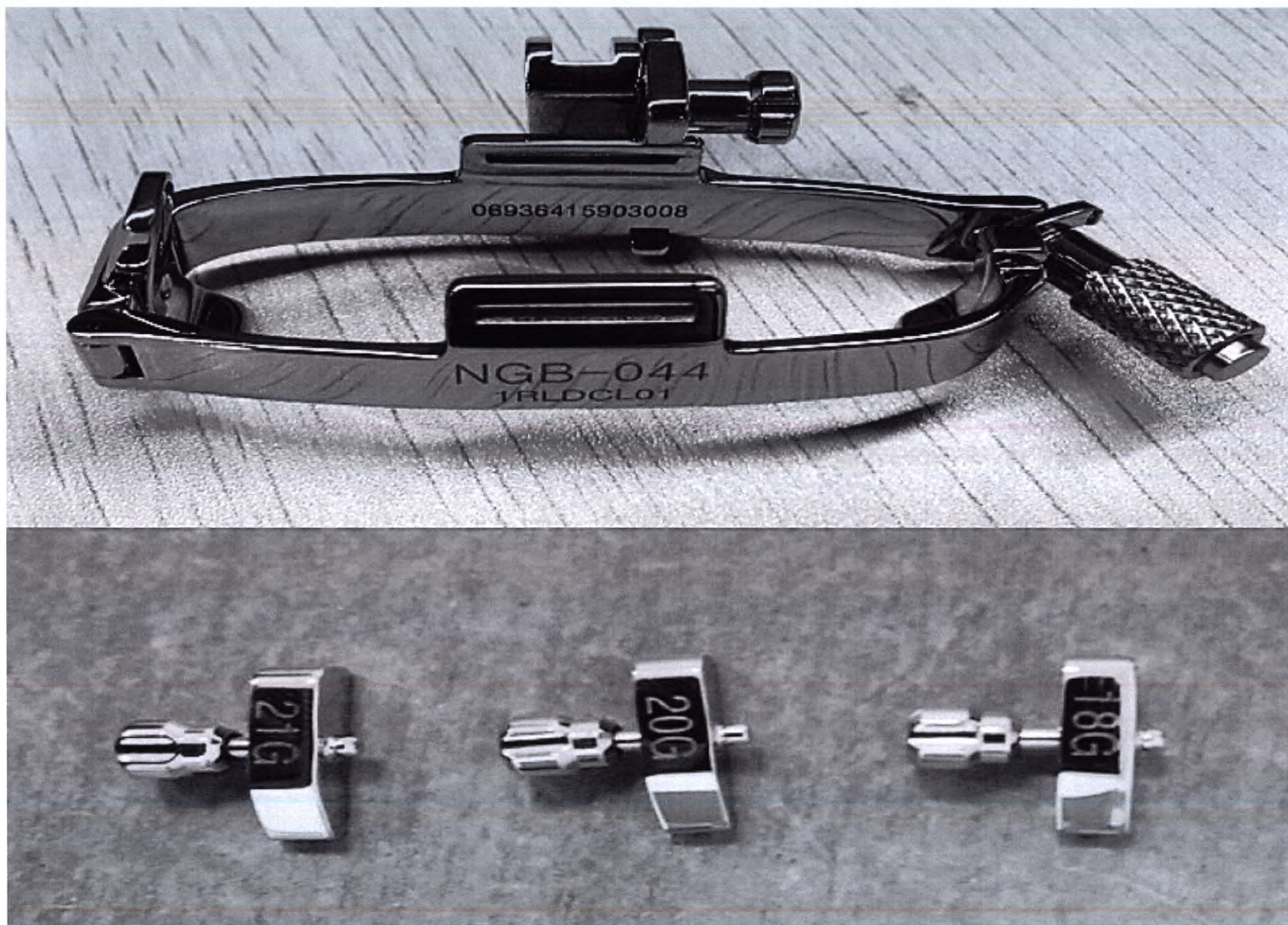
Насадка биопсийная металлическая, со съемной направляющей для игл NGB-044
