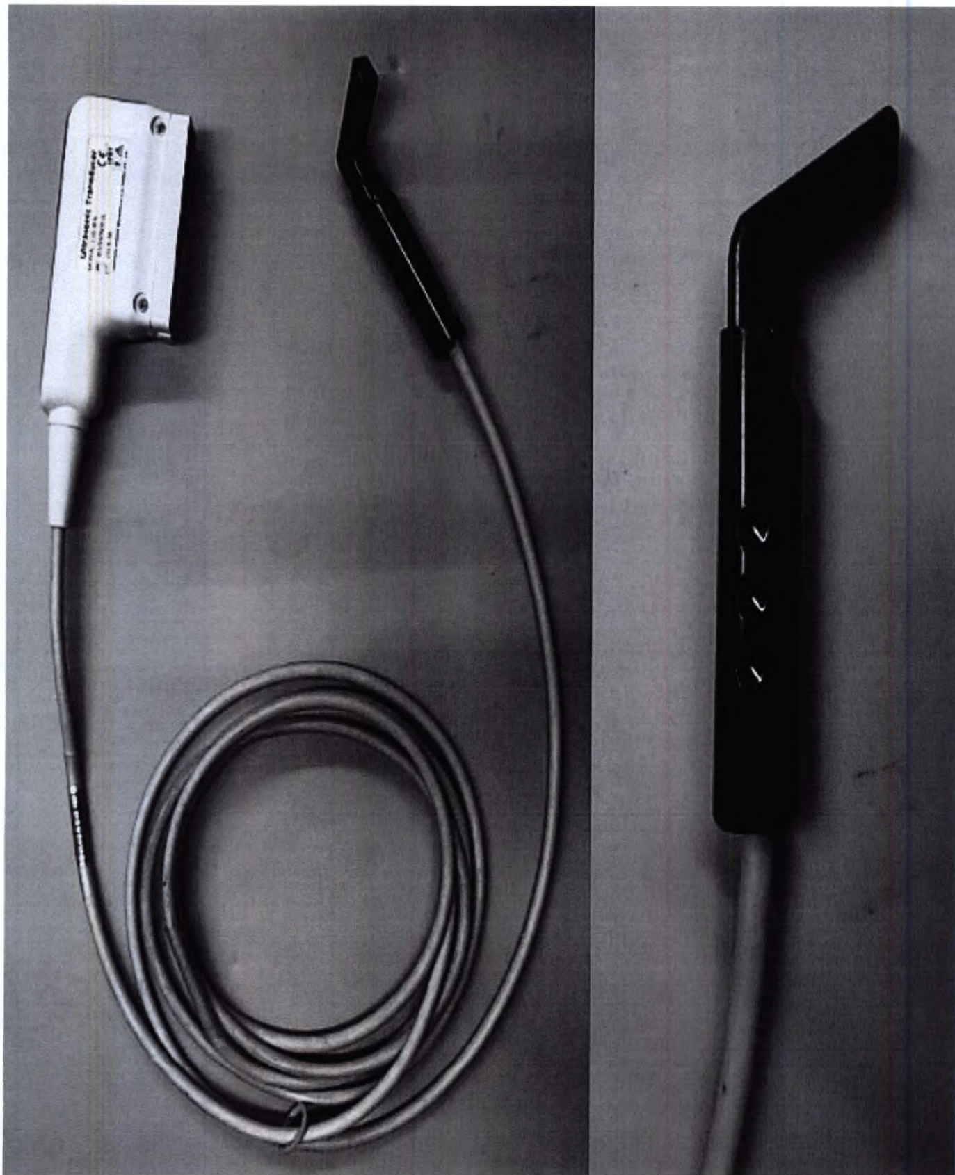
Датчик ультразвуковой интраоперационный L16-4Hs
