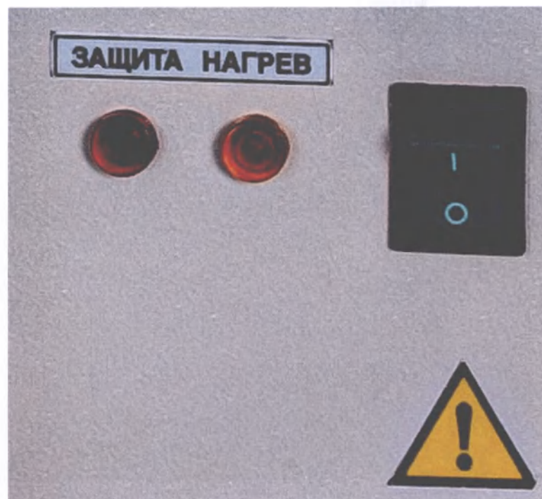
Рисунок 3 – Общий вид приборной панели и панели управления стерилизатора воздушного ГП-80 СПУ по ТУ 9451-012-00141798-2005
