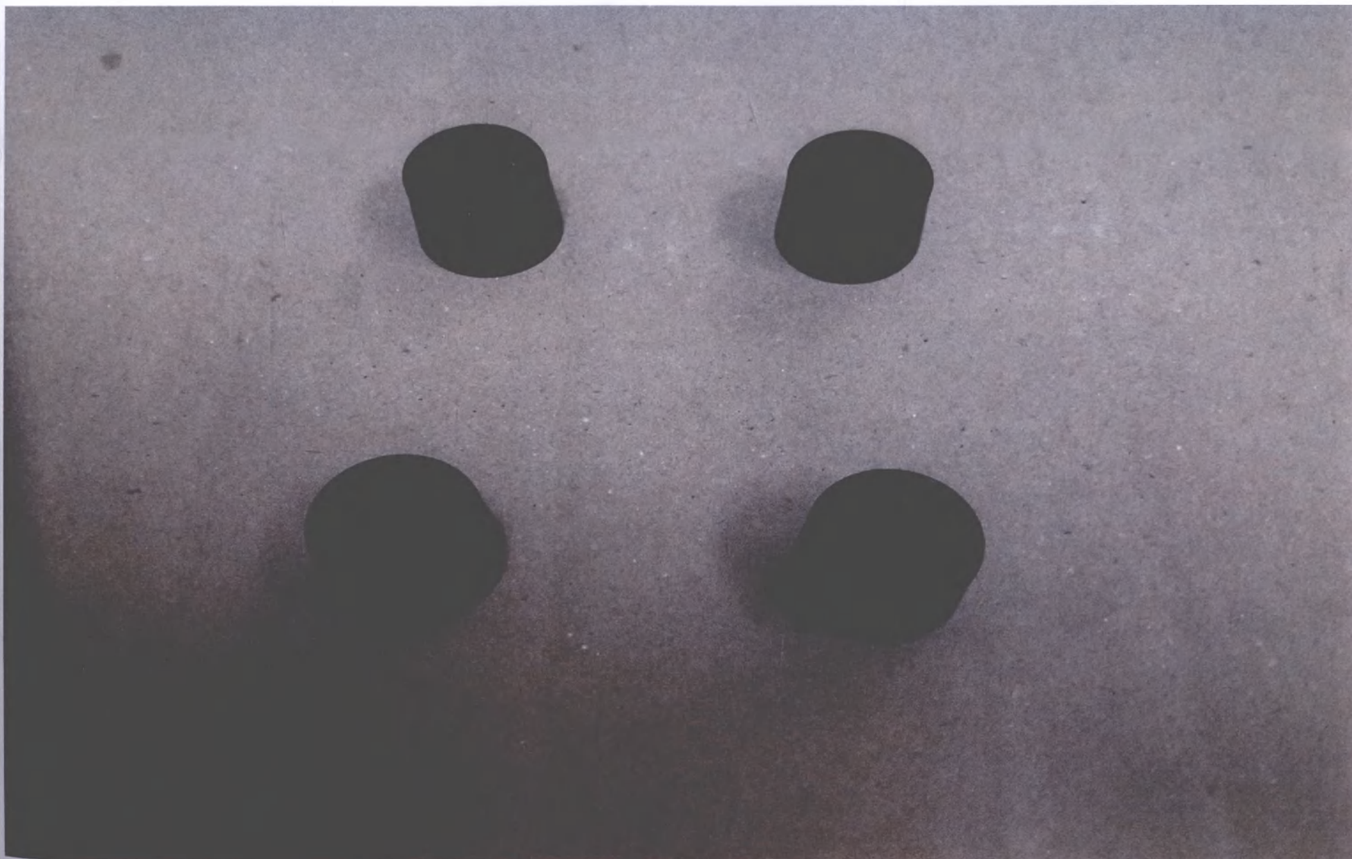
Рисунок 5 – Общий вид ножек стерилизатора воздушного ГП-80 СПУ по ТУ 9451-012-00141798-2005
