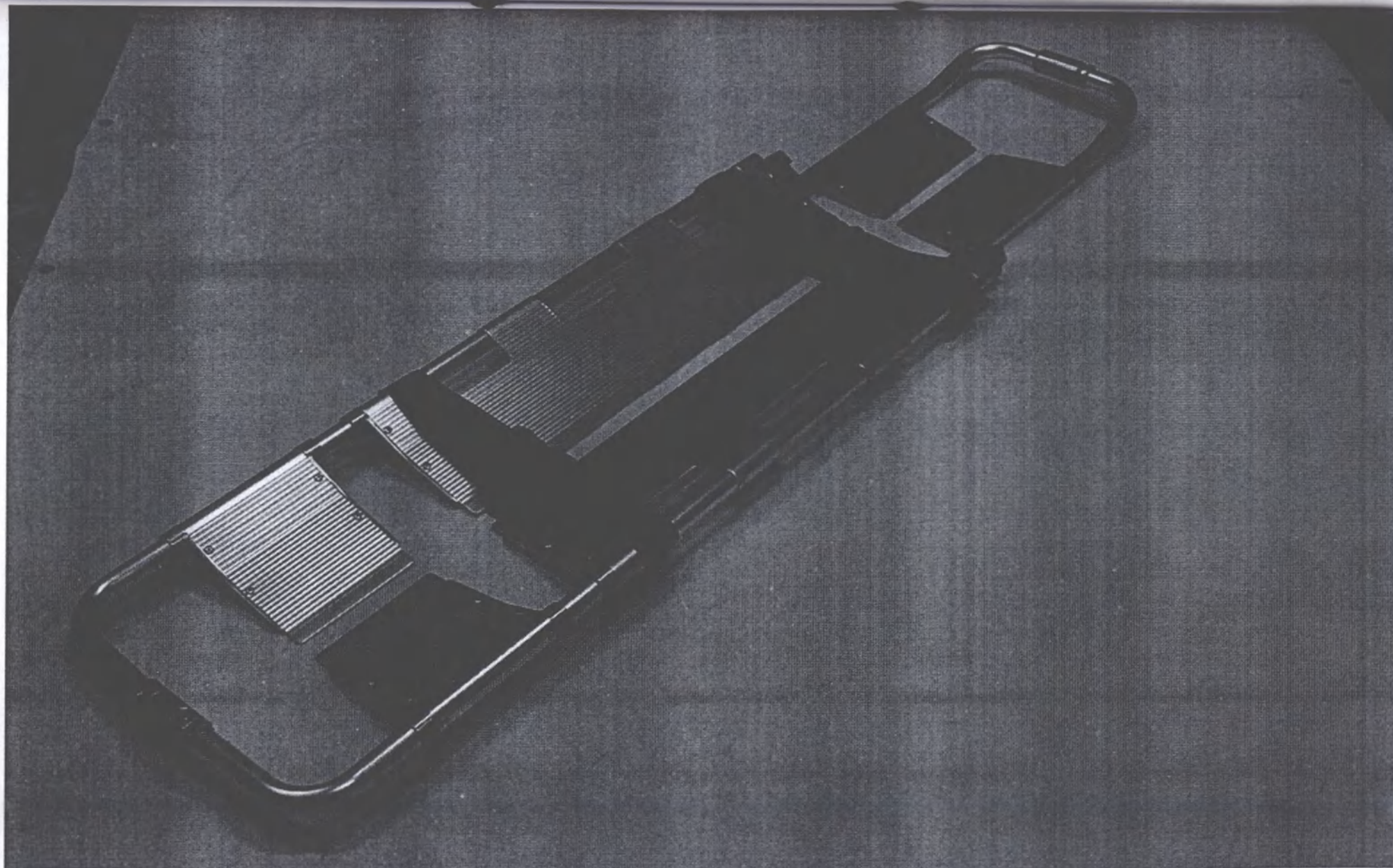
Носилки медицинские DDJ-3C с принадлежностями. Общий вид
