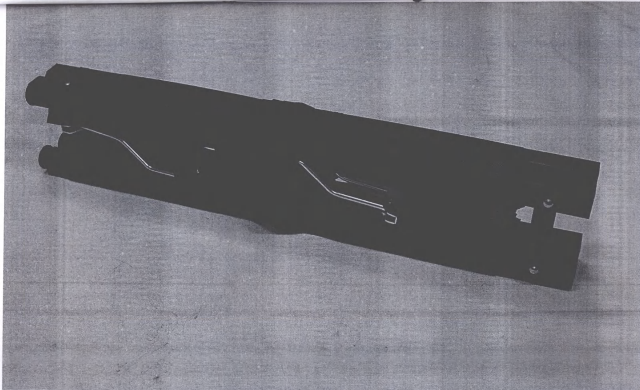
Носилки медицинские DDJ-2F с принадлежностями. Общий вид в сложенном состоянии
