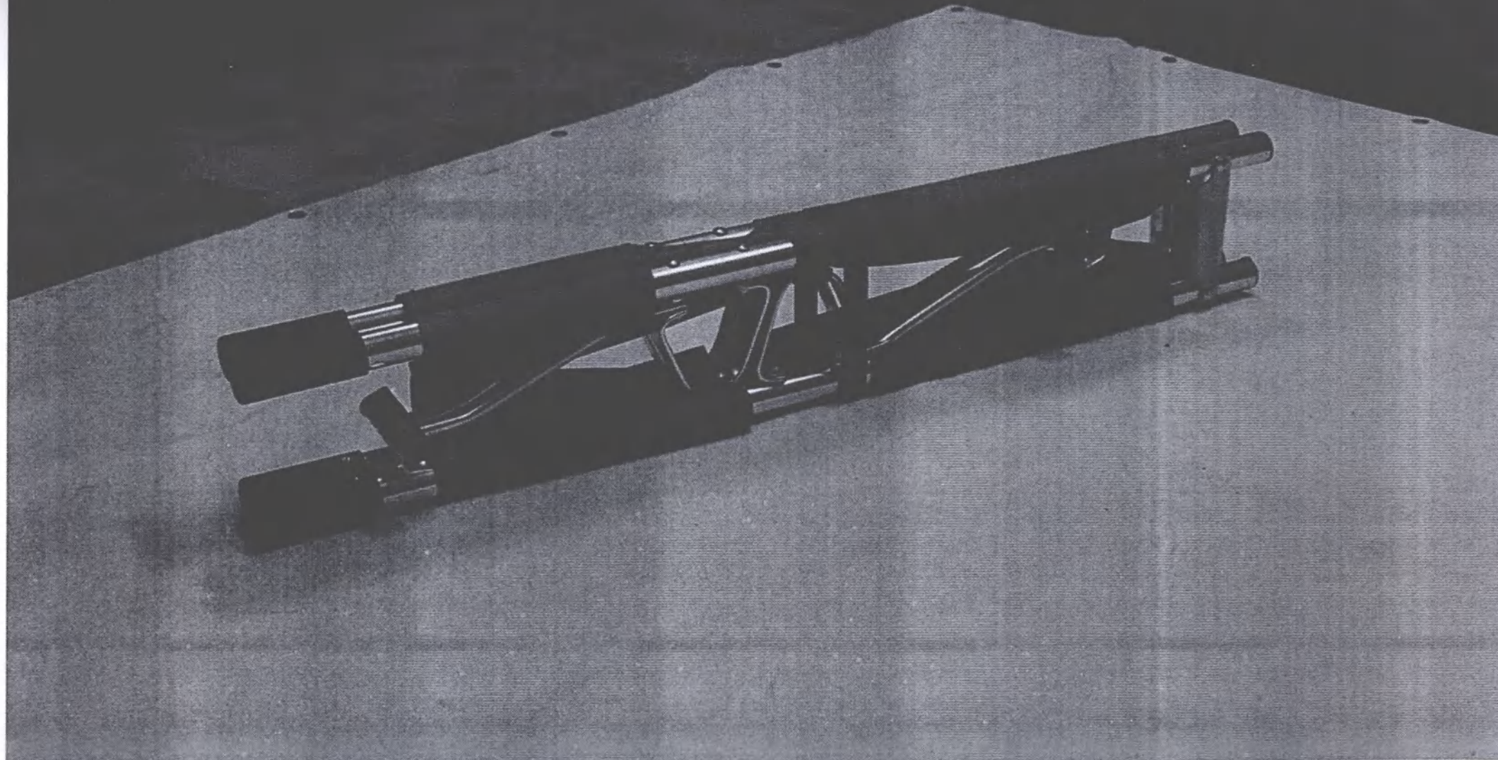
Носилки медицинские DDJ-2A с принадлежностями. Общий вид в сложенном состоянии
