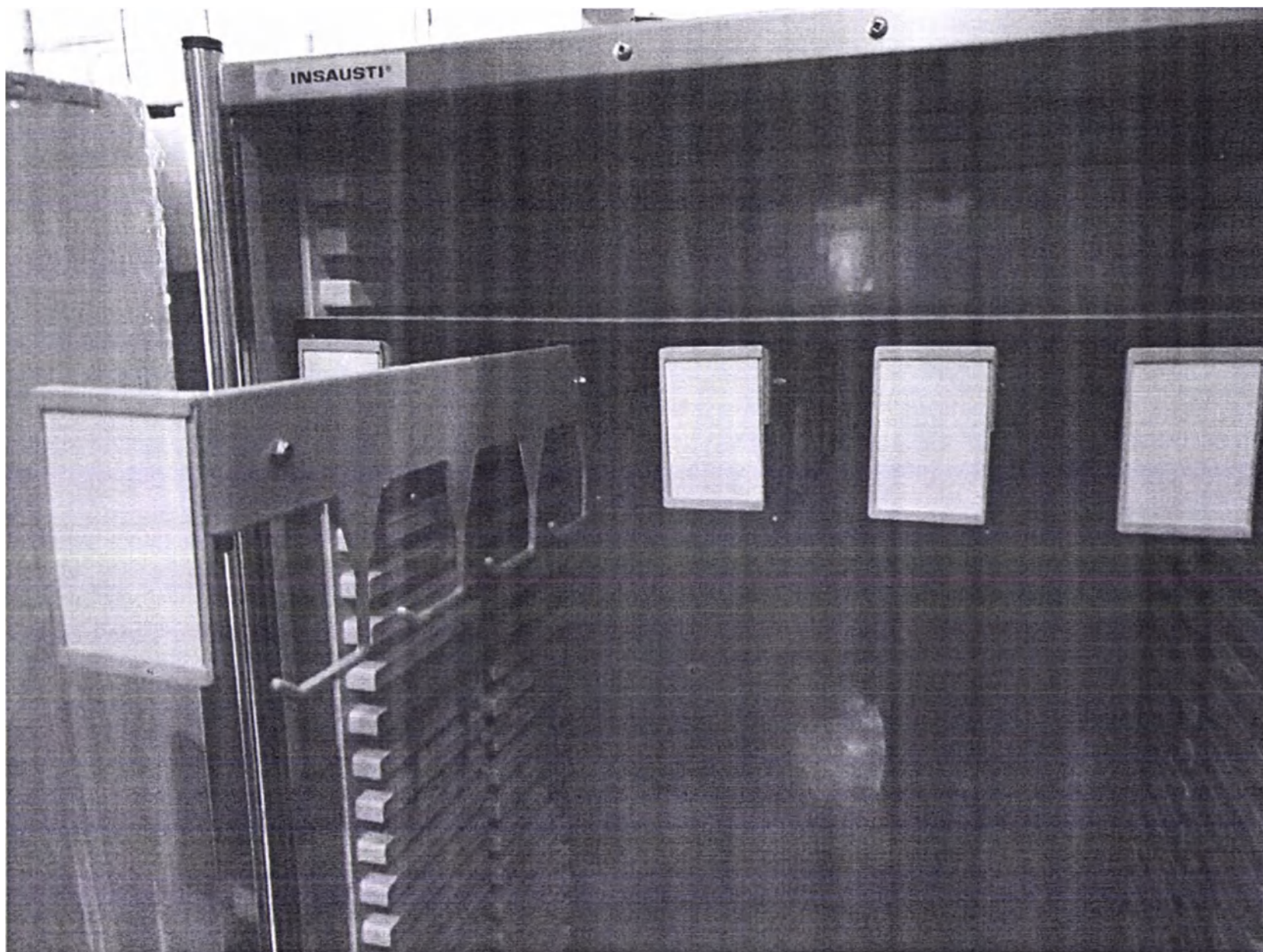
«Тележка универсальная внутрибольничная», в вариантах исполнения, с принадлежностями: «Тележка серии 600, с панелями», «Тележка серии 700, с панелями» -- Полка регулируемая, для катетеров
