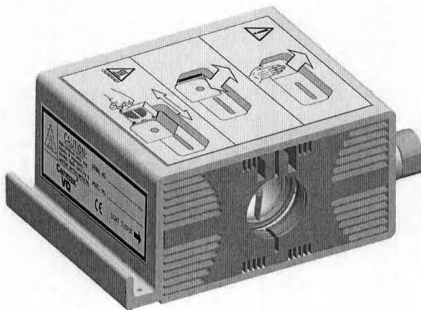
Рис. 12.1 Модуль ксеноновой лампы Cermax VQ
