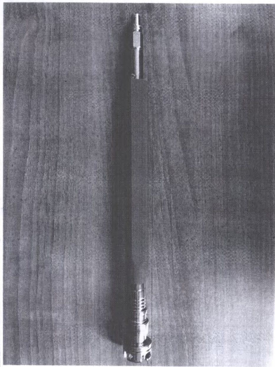
Фото 18. Рукоятка для захвата фрезы ацетабулярной
