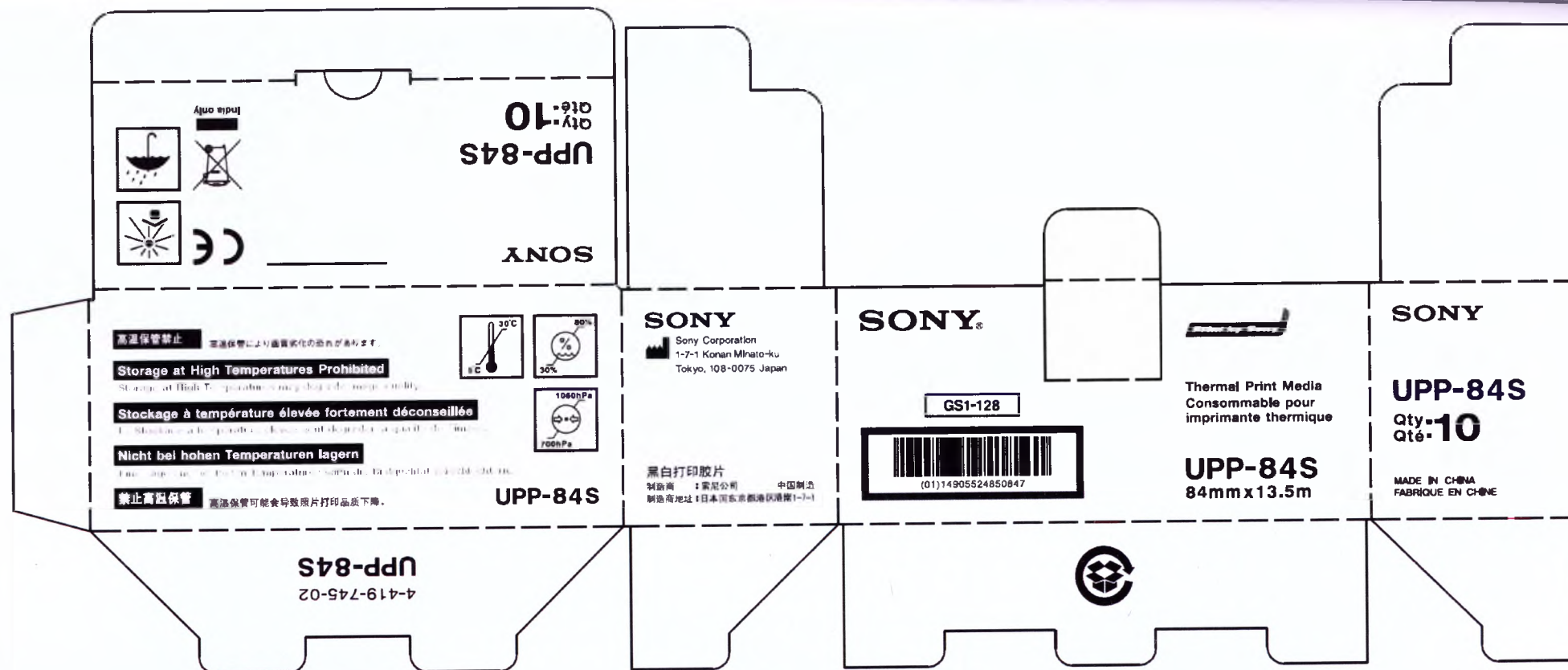
Макет упаковки 24. UPP-84S. Индивидуальная упаковка
