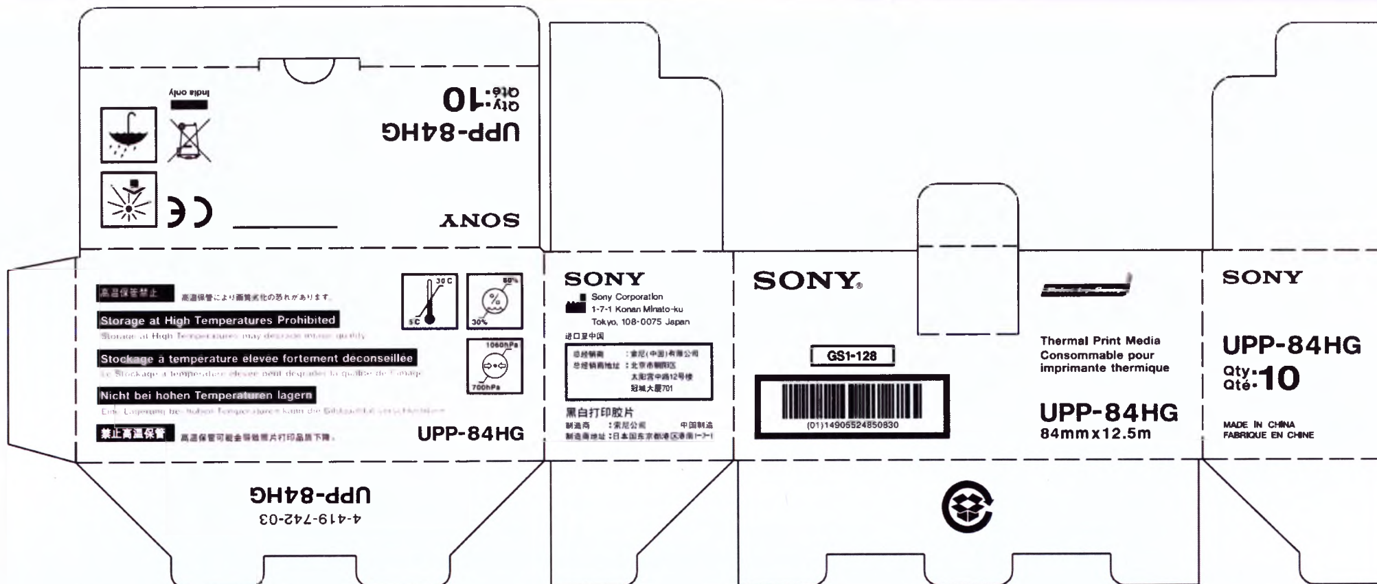
Макет упаковки 20. UPP-84HG. Индивидуальная упаковка
