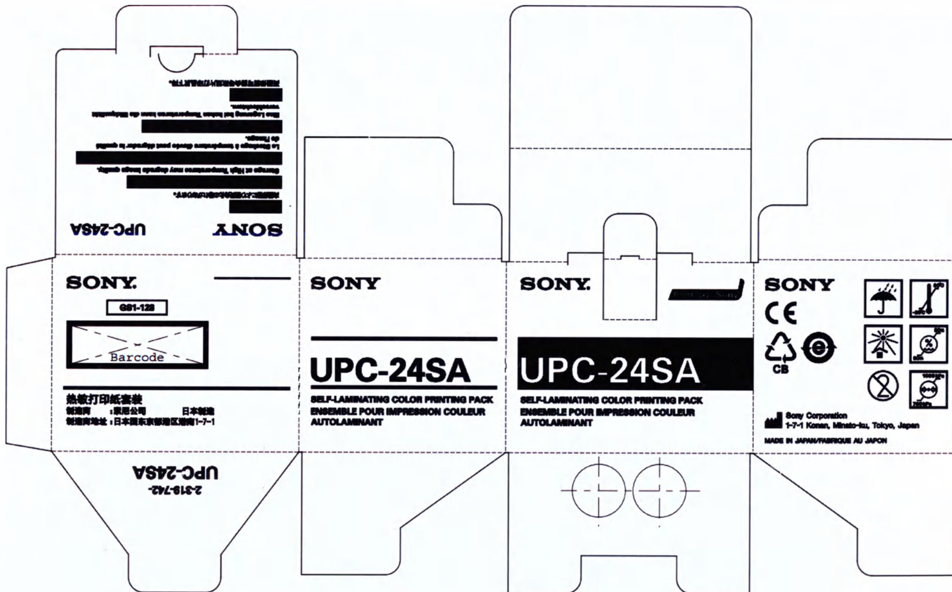
Макет упаковки 11. UPC-24SA. Индивидуальная упаковка
