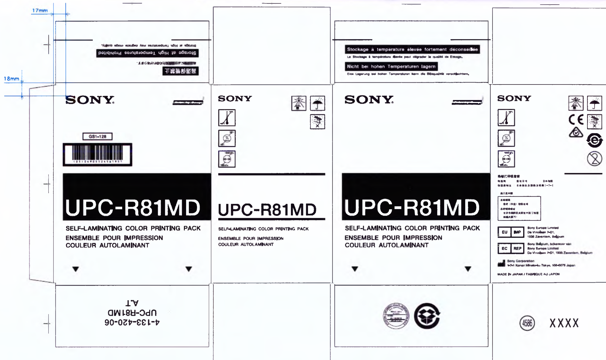
Макет упаковки 17. UPC-R81MD. Индивидуальная упаковка
