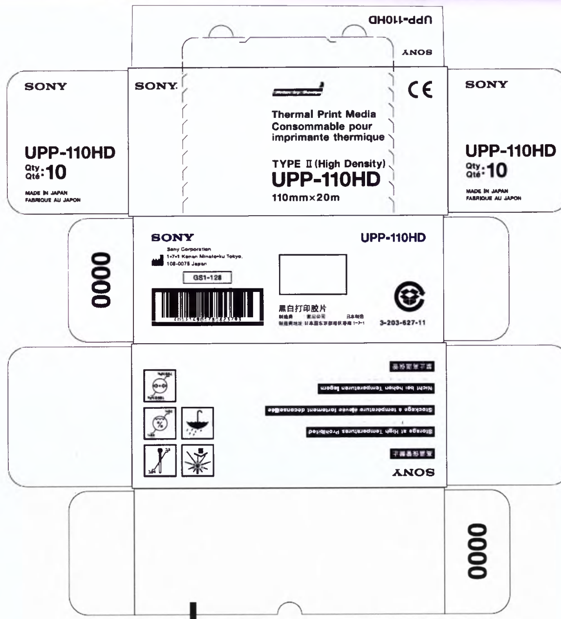
Макет упаковки 29. UPP-110HD. Индивидуальная упаковка
