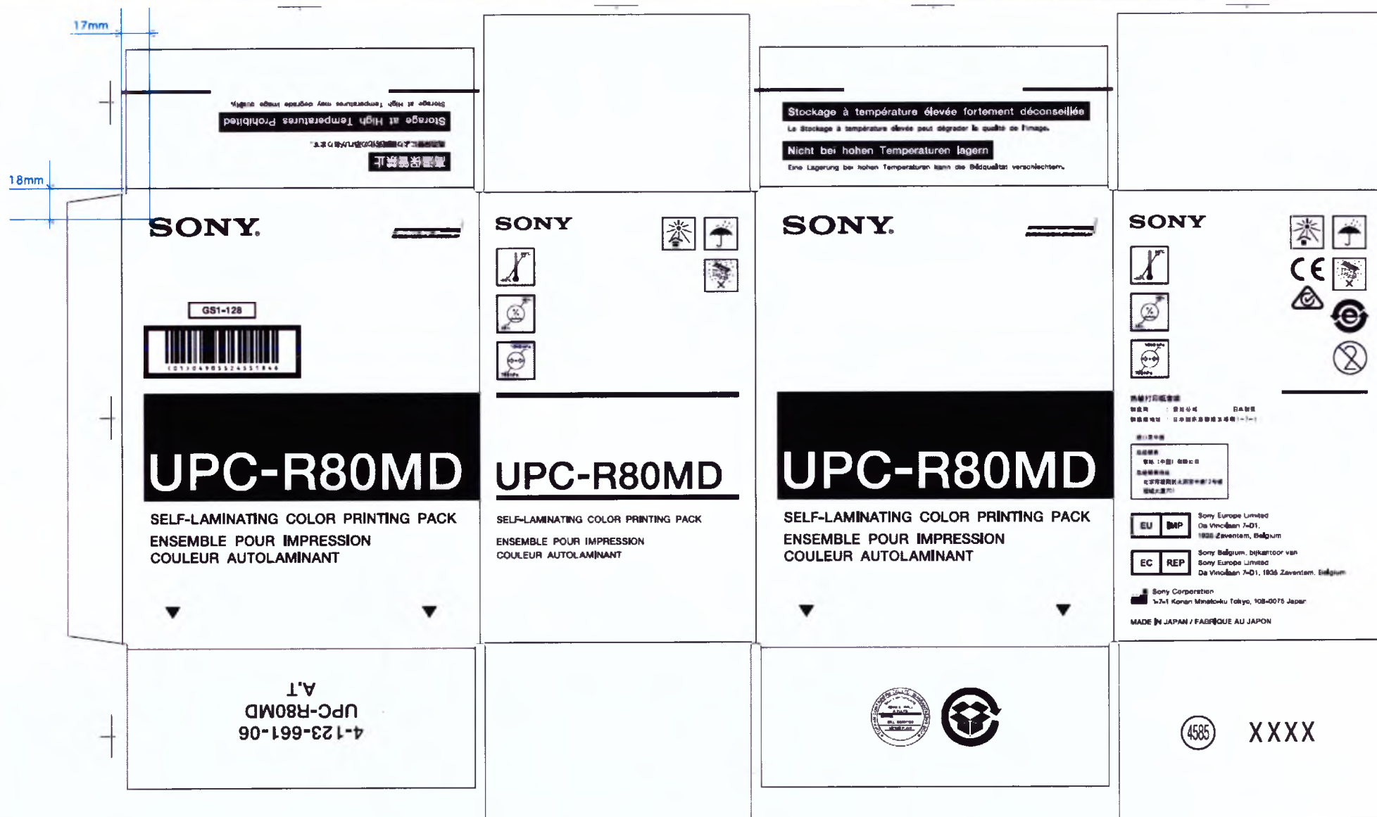
Макет упаковки 14. UPC-R80MD. Индивидуальная упаковка
