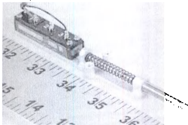
45. Приспособление для настройки лазерного указателя (от 1 до 4 шт.).
