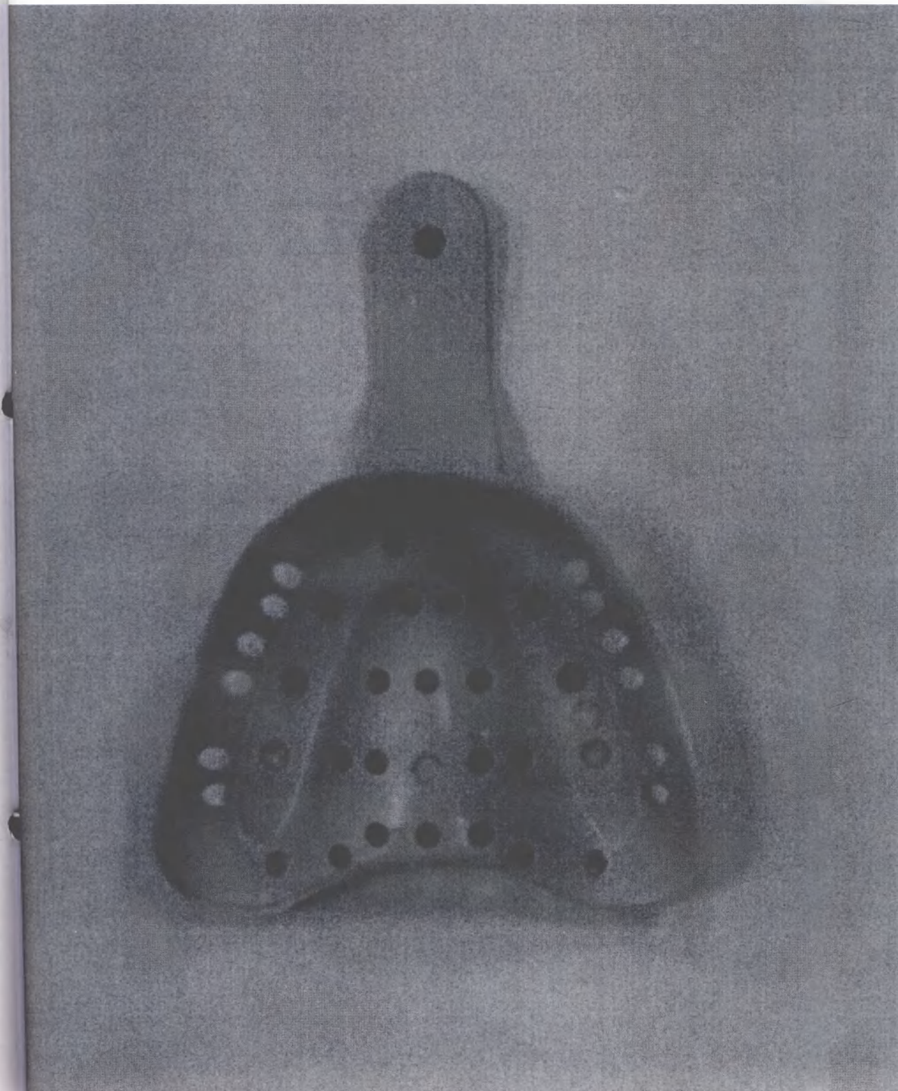
22. Общий вид изделия «Ложка стоматологическая для оттиска верхней челюсти полимерная №4».
