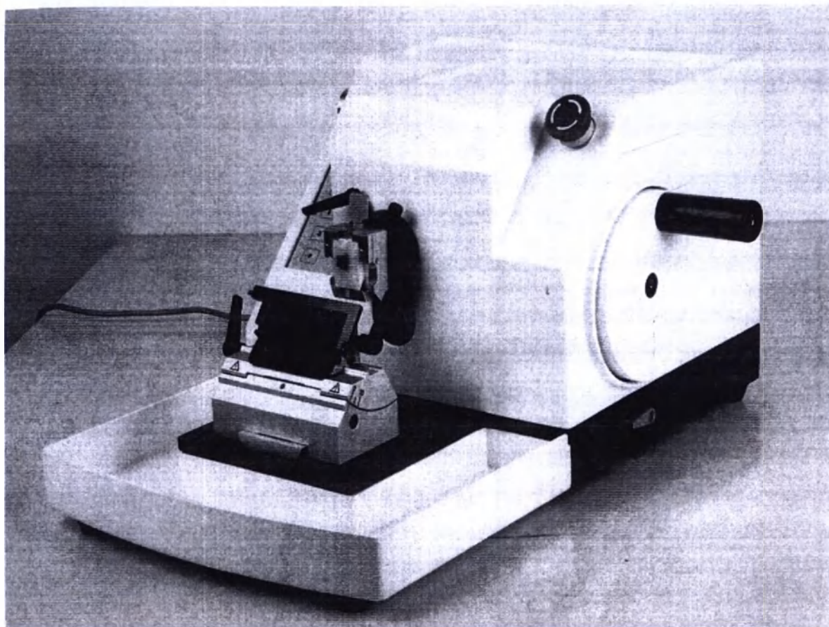
Фотографическое изображение 2. Микротом ротационный KEDEE®: микротом-автомат модели KD-3398, KD-3368AM, микротом-полуавтомат KD-3390, KD-3358 с принадлежностями. Микротом-автомат модель KD-3368AM
