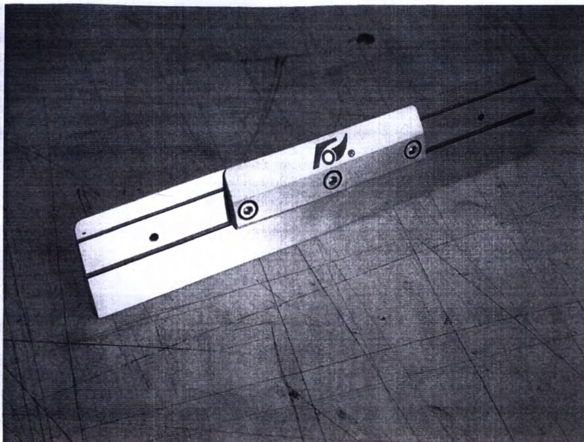
Фотографическое изображение 22. Микротом ротационный KEDEE®: микротом-автомат модели KD-3398, KD-3368AM, микротом-полуавтомат KD-3390, KD-3358 с принадлежностями. Держатель лезвий сменный KD-16A
