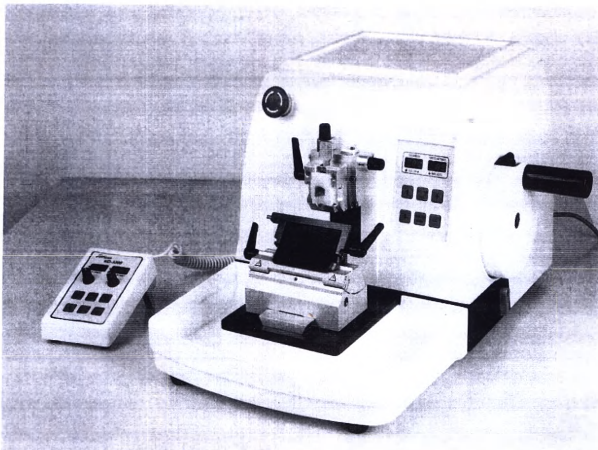
Фотографическое изображение 1. Микротом ротационный KEDEE®: микротом-автомат модели KD-3398, KD-3368AM, микротом-полуавтомат KD-3390, KD-3358 с принадлежностями. Микротом-автомат модель KD-3398
