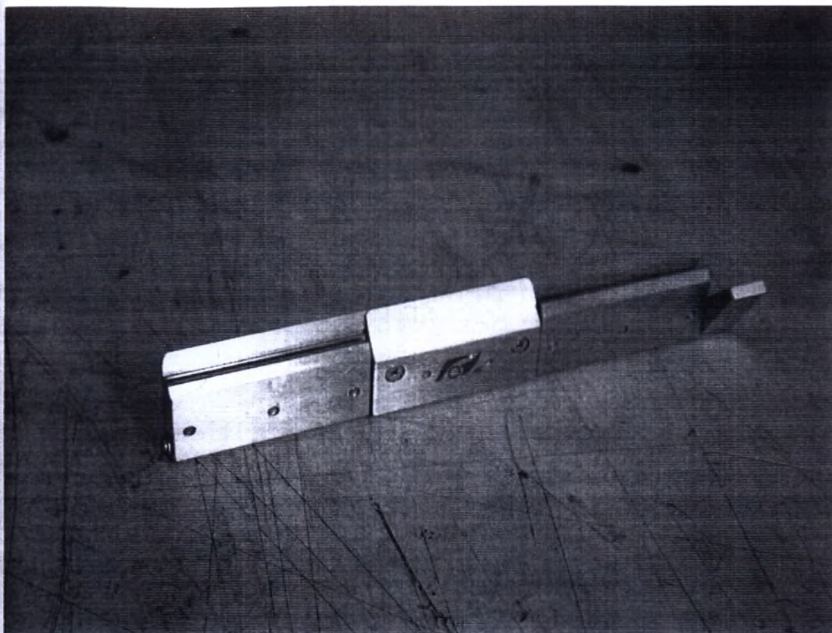
Фотографическое изображение 23. Микротом ротационный KEDEE®: микротом-автомат модели KD-3398, KD-3368AM, микротом-полуавтомат KD-3390, KD-3358 с принадлежностями. Держатель лезвий сменный KD-16B
