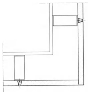
Односторонние панели Single wall panel
