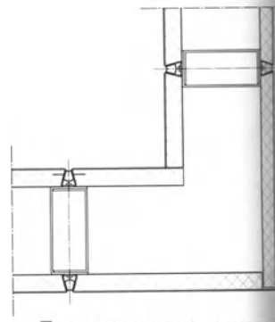
Двусторонние панели Double wall panels
