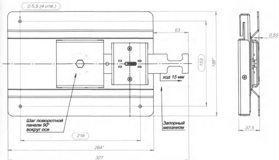
Рисунок 9. Чертеж кронштейна в сборе
