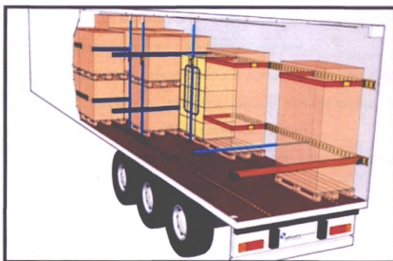
Рисунок 29. Пример крепления груза.
