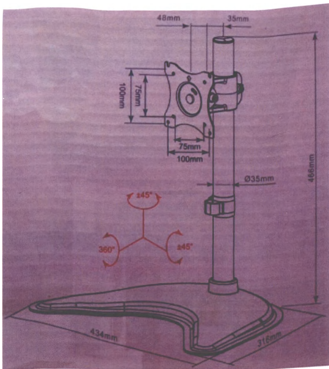
Рисунок 11. Чертеж подставки
