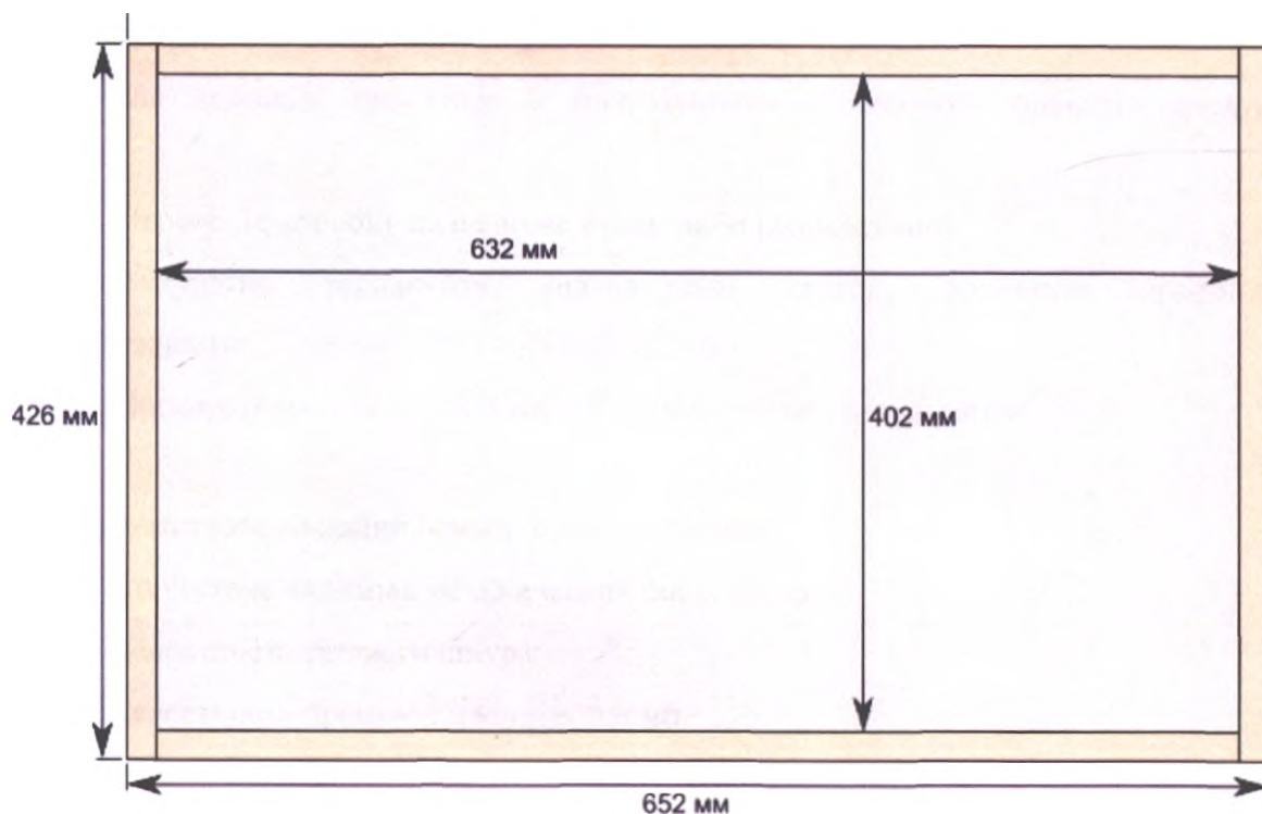
Рисунок 14. Чертёж защитного кожуха
