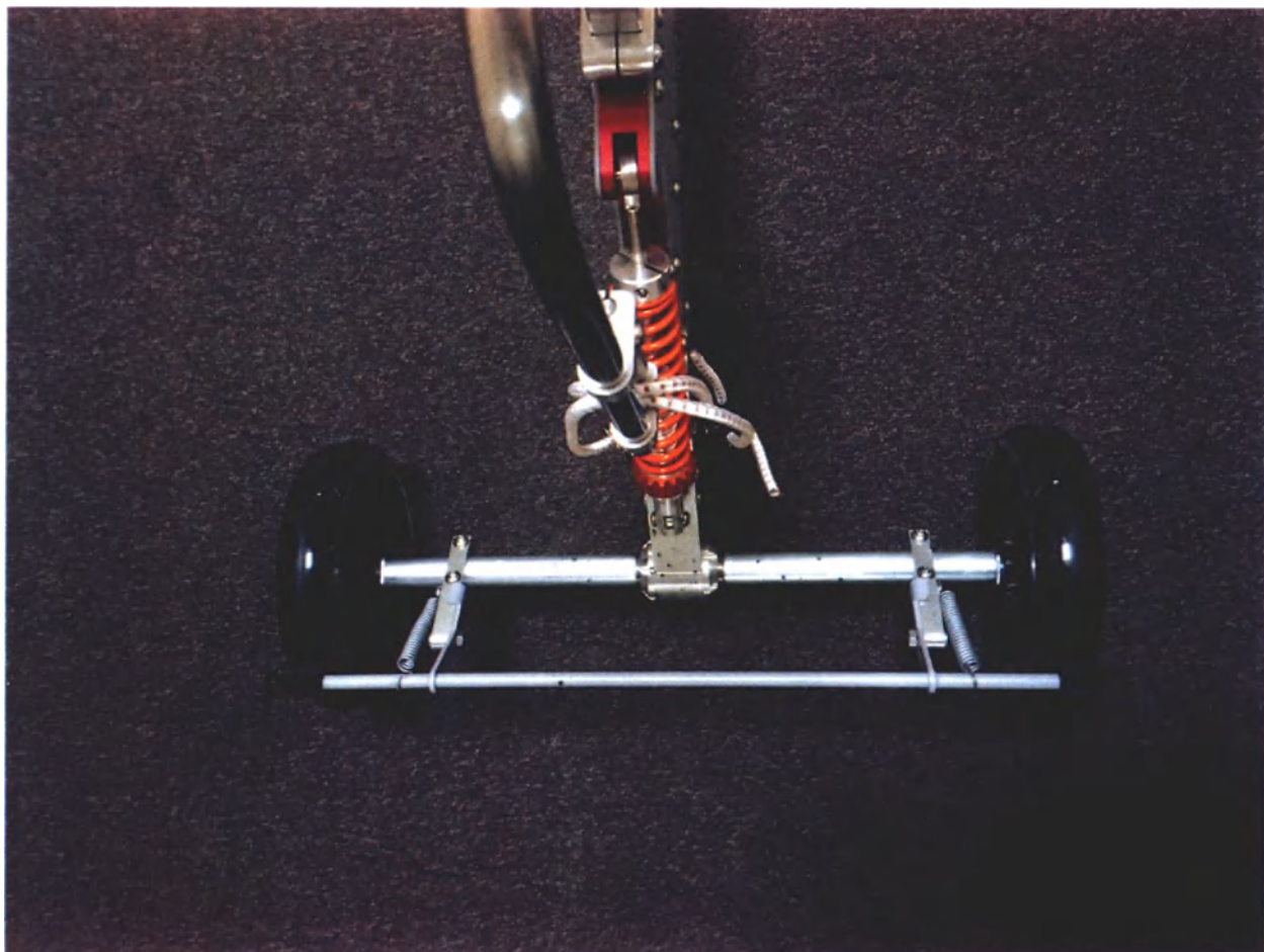
Рисунок 2 - Фотографическое изображение: динамическая платформа в сборе
