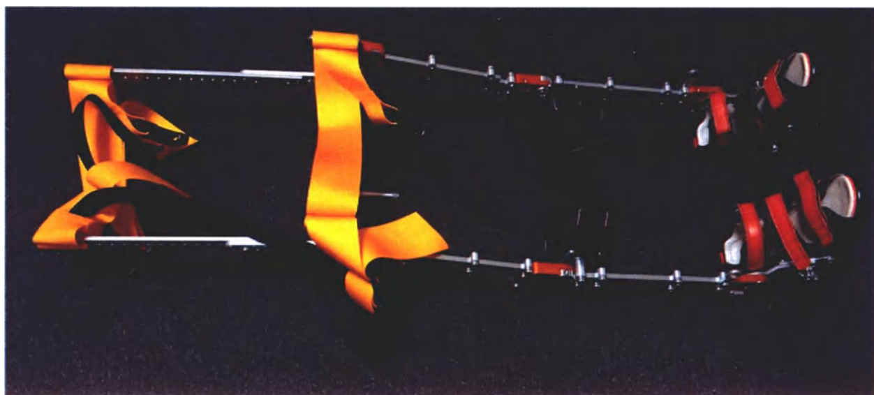
Рисунок 2 - Фотографическое изображение: динамическая платформа в сборе
