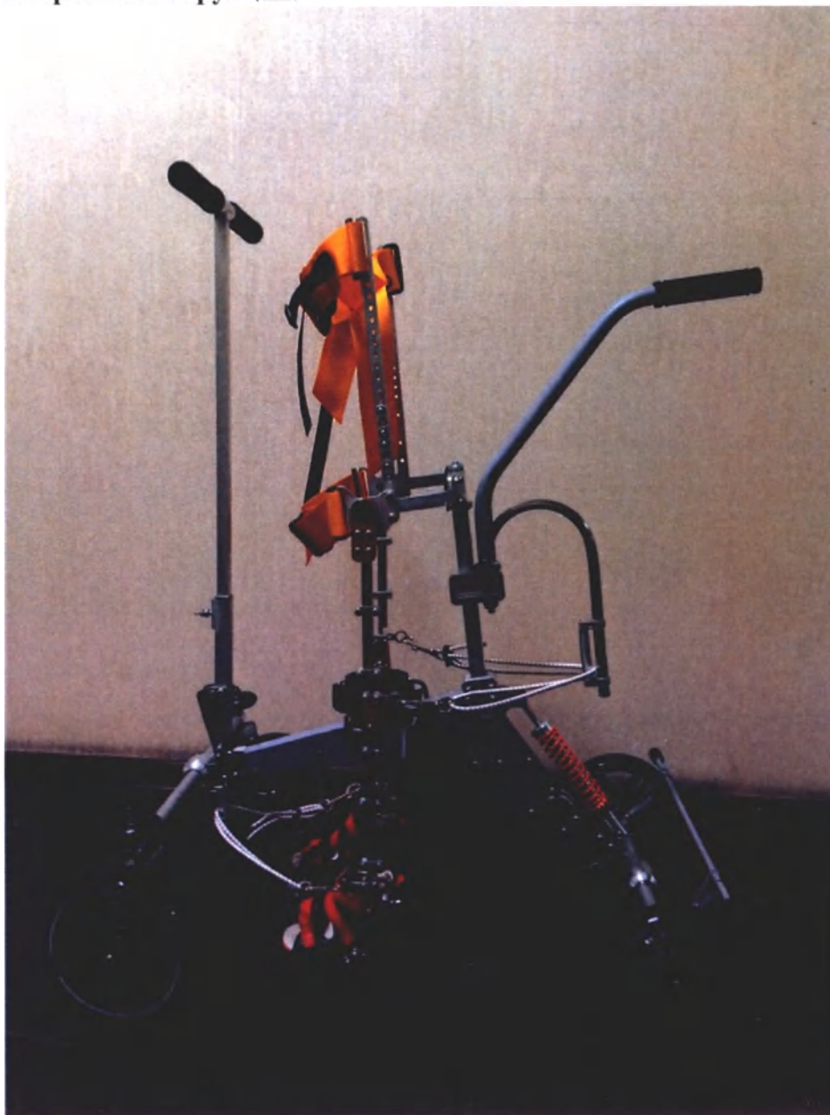
Рисунок 1 - Фотографическое изображение: Аппарат на нижние конечности и туловище (ортез) «ЭкзоБот» по ТУ 32.50.22-001-29664790-2020 в сборе, без дополнительных опций
