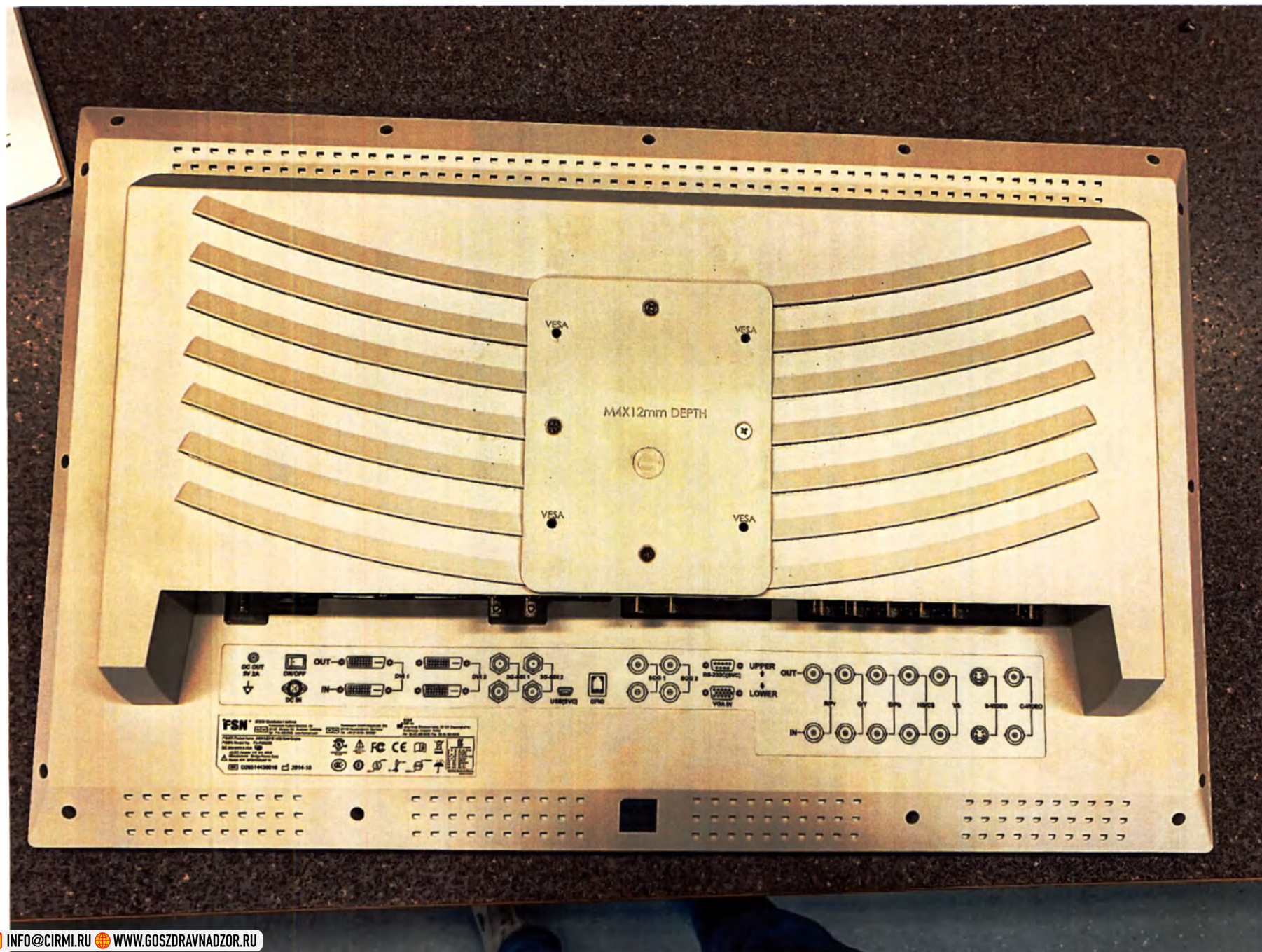
Монитор LCD медицинского назначения, модель FS-P2603D с диагональю 26'' (66,04 см): Тыльная сторона
