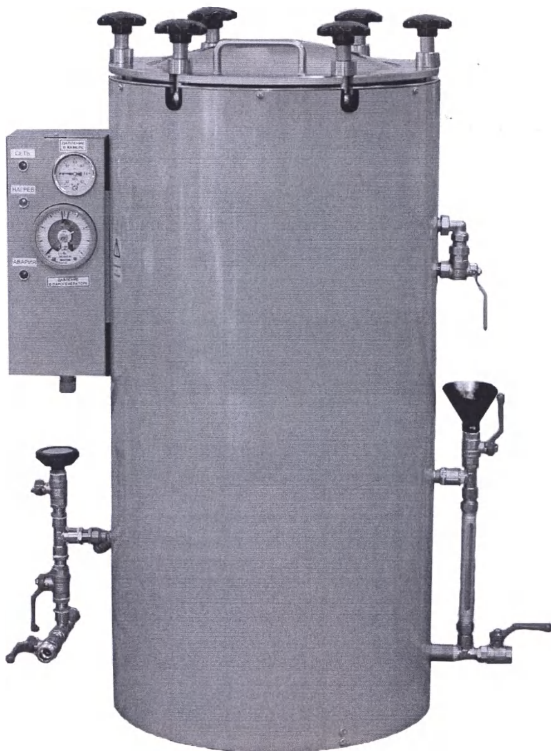
Фотографическое изображение 3. Стерилизатор паровой ВКа-75-ПЗ в варианте исполнения КИУС.942711.001-01. Внешний вид.
