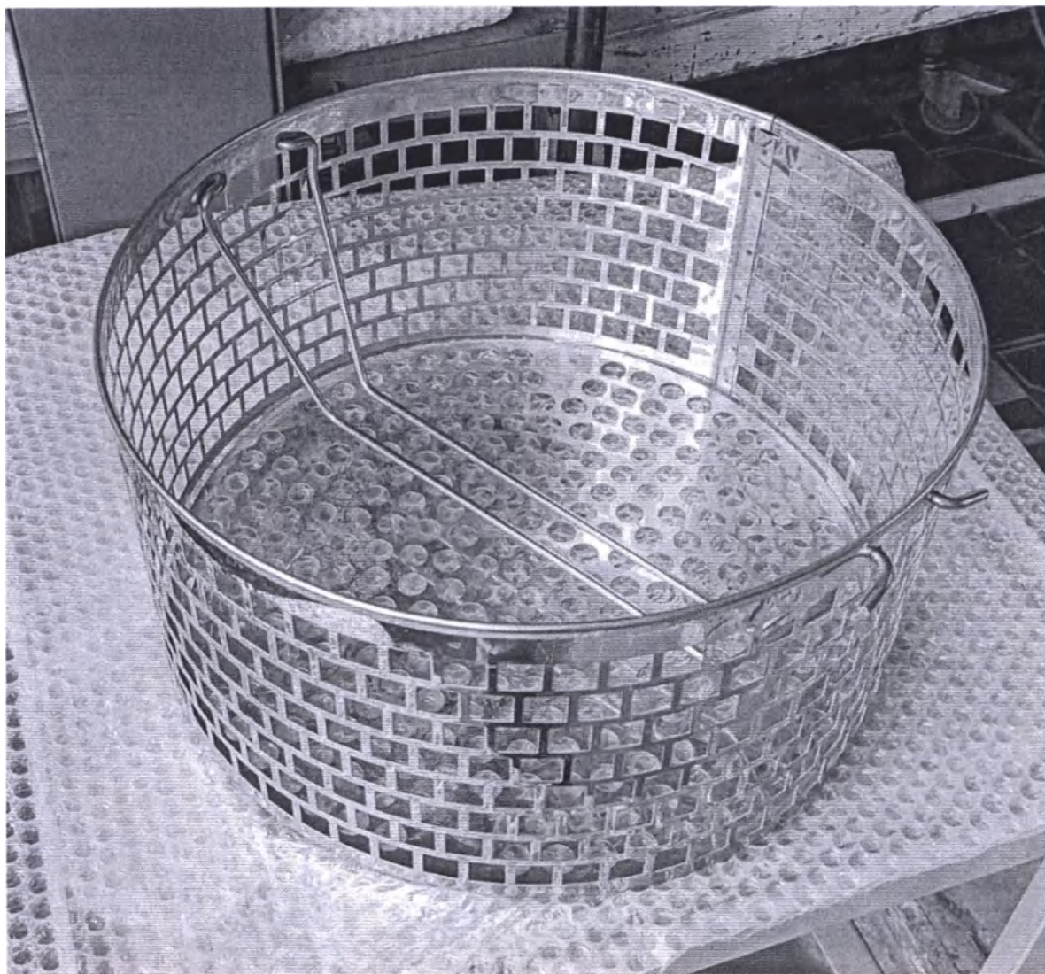
Фотографическое изображение 11. Корзина загрузочная.
