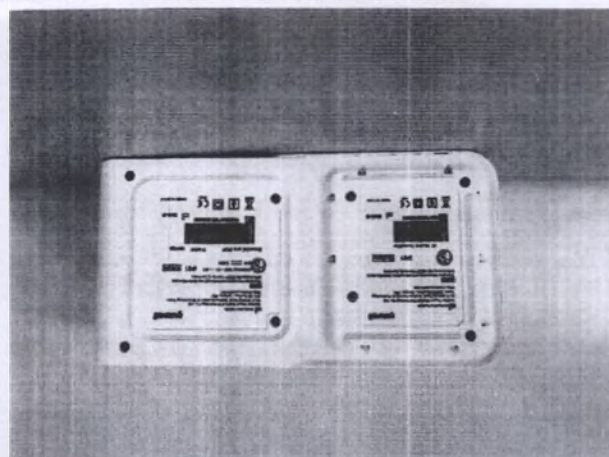
Корпус основной ПМ-720 (в корпусе установочном) в открытом виде
