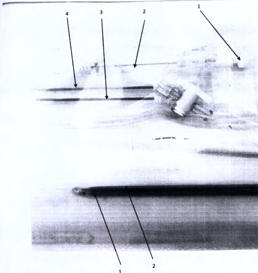
1 – толкатель; 2 - канюля установочная; 3 – устройство коррекции установки стента; 4 - устройство извлечения
