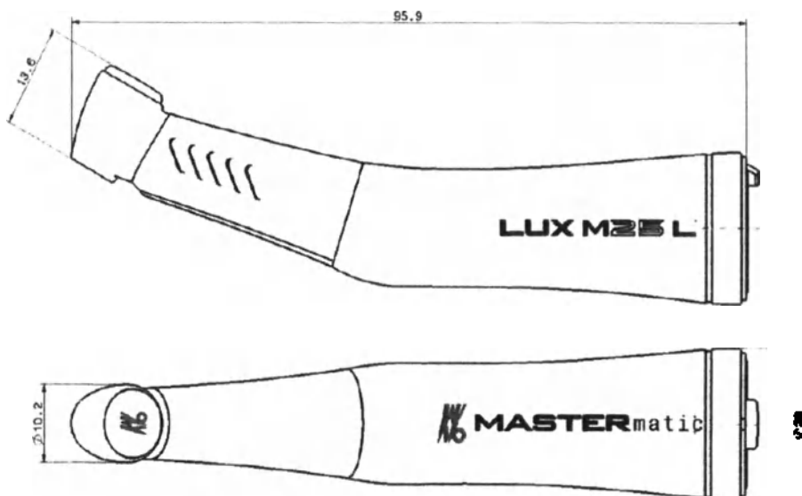
MASTERmatic LUX M25 L (Арт. № 1.009.3630)
