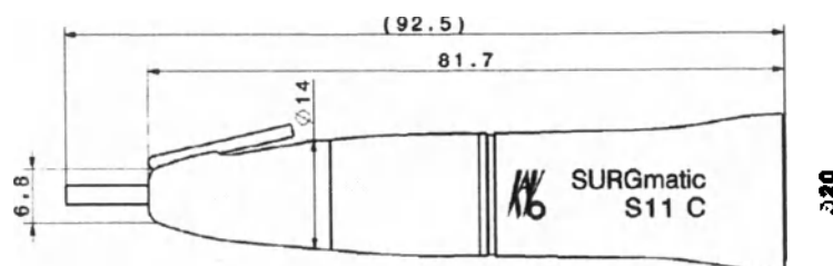
SURGmatic S11 C (Арт. № 1.009.1005)
