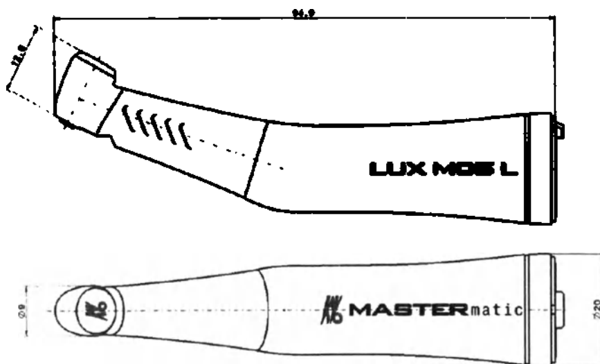
MASTERmatic LUX M05 L (Арт. № 1.009.3640)
