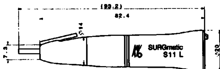
SURGmatic S 11L (Арт. № 1.009.1010)
