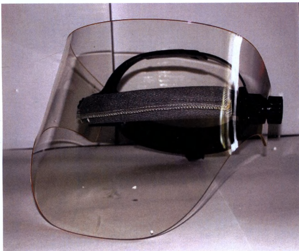
Рис. 23 – Маска рентгенозащитная
