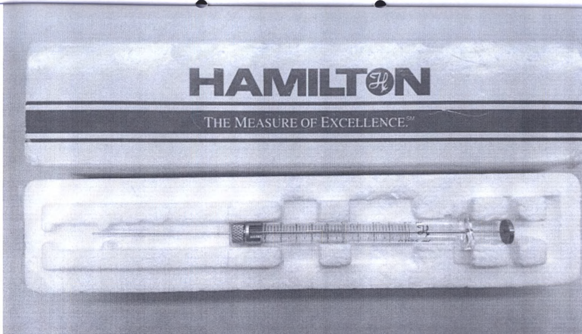
Фотографическое изображение 6 – Шприц для введения пробы, 25 мкл (Hamilton)
