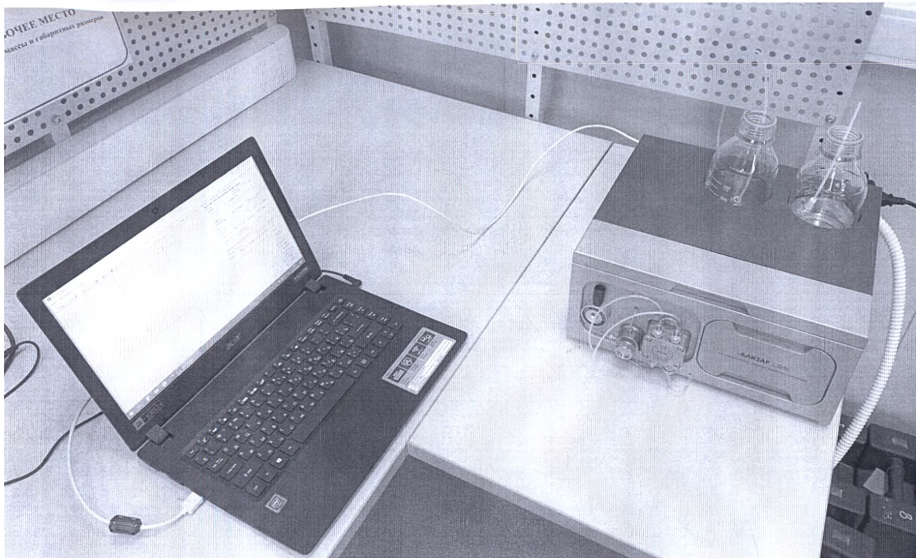
Фотографическое изображение 1 – Общий вид образца изделия Хроматограф жидкостный портативный «Близар CDT» (на фотографии Хроматограф жидкостный портативный «Близар CDT», USB-кабель, Бутыли для элюентов)
