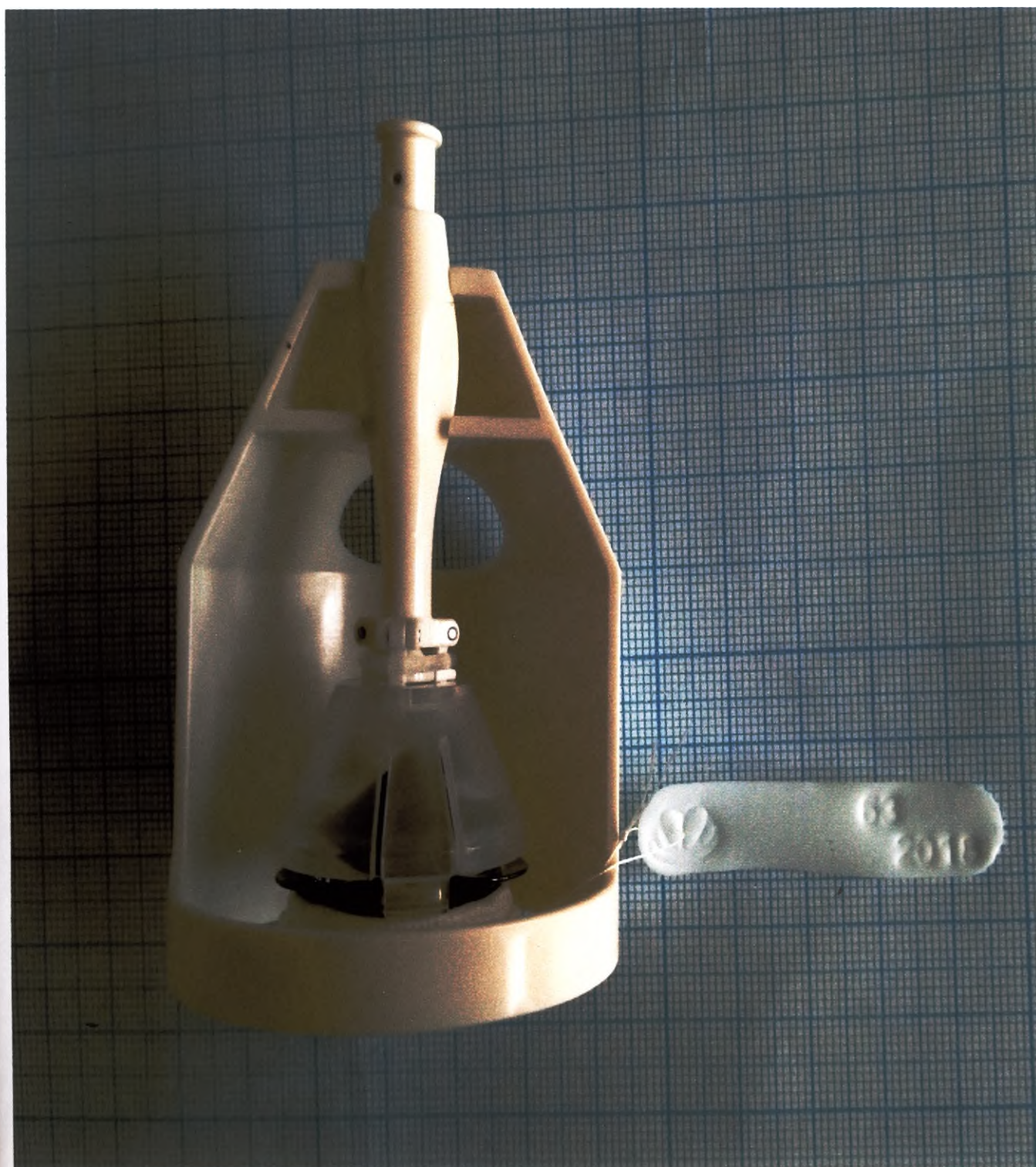
Фото 8. Протез клапана сердца "ТриЛИКС-Турбо" с технологическим ярлыком на держателе в кожухе
