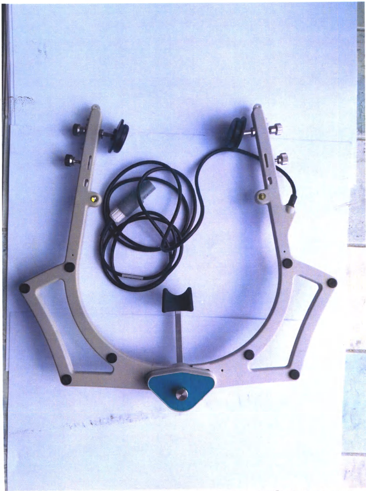
Фото 3. Дуга лицевая с опорами и кабелем подсоединения к блоку управления.
