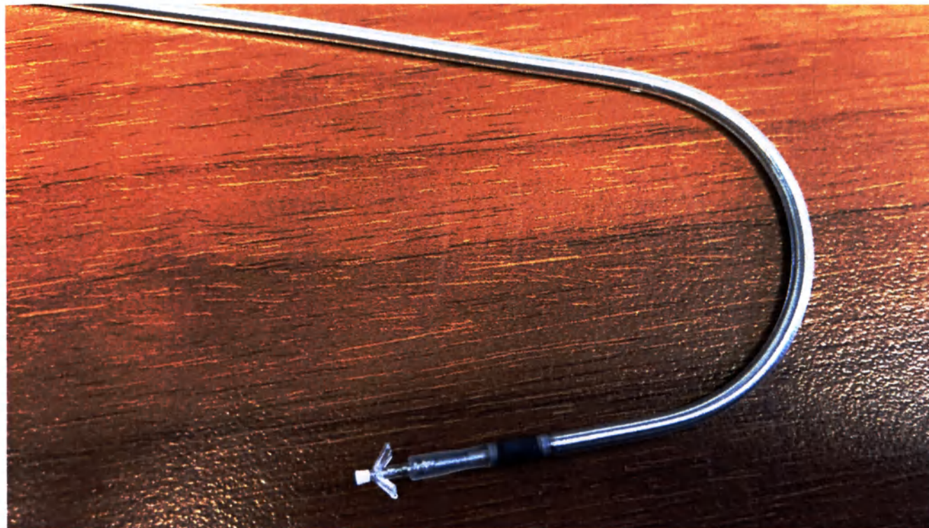
Электрод имплантируемый эндокардиальный Solia JT 53 (дистальный полюс)
