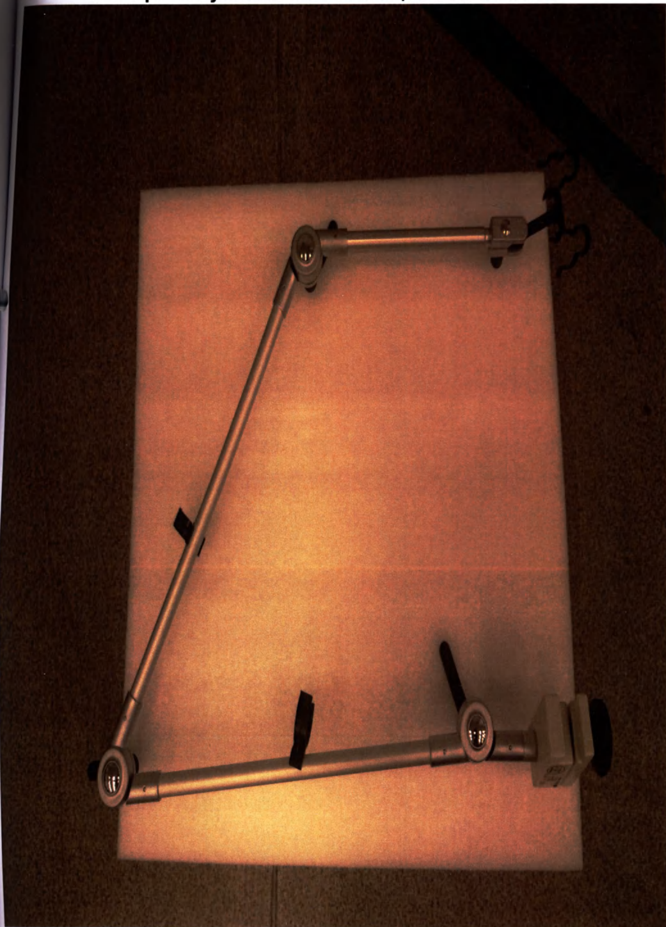
Фото 12 – Перчататель дыхательного контура в сборе.
