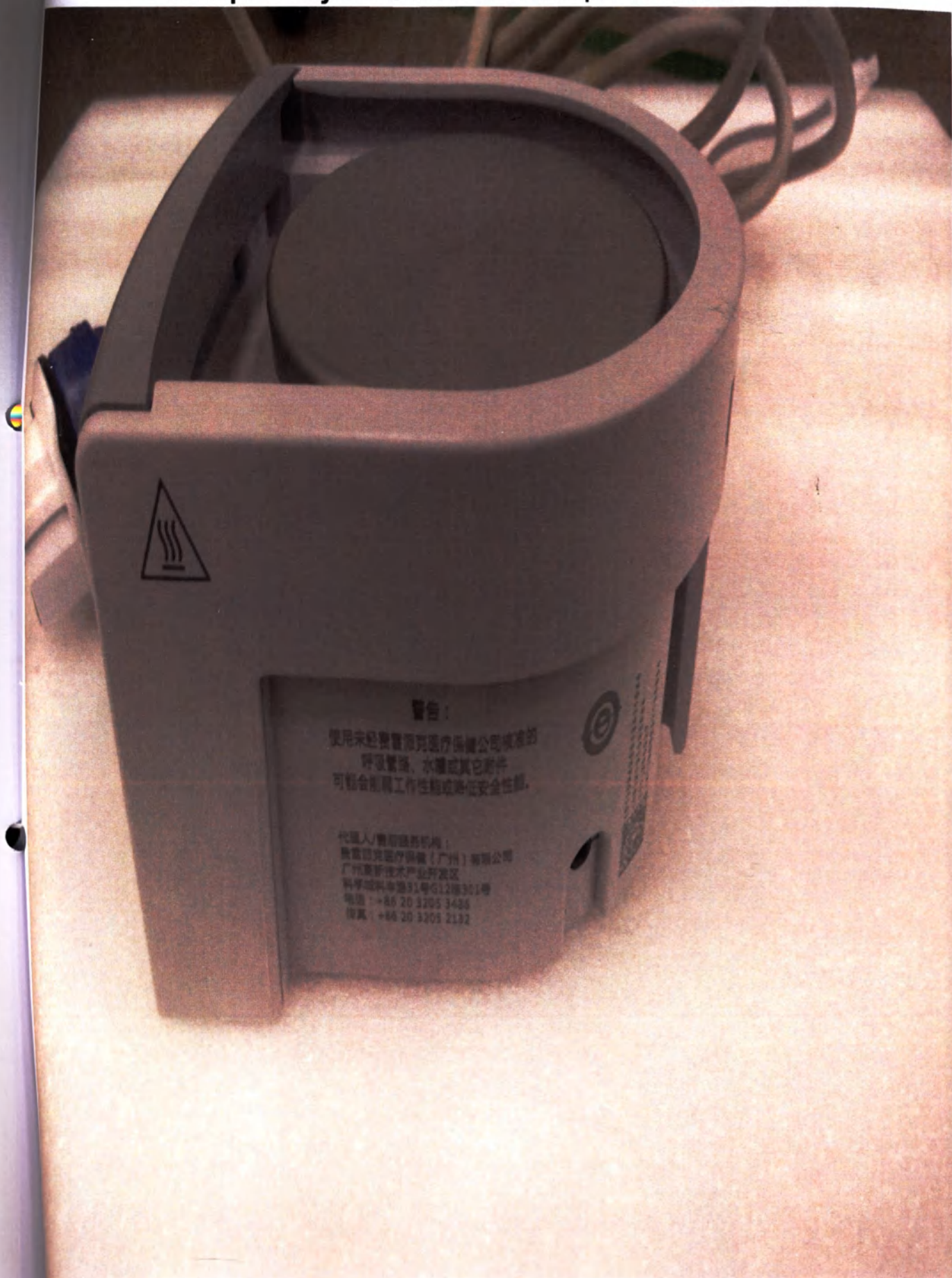
Фото 25 - Нагревательный блок увлажнителя (вид сбоку).
