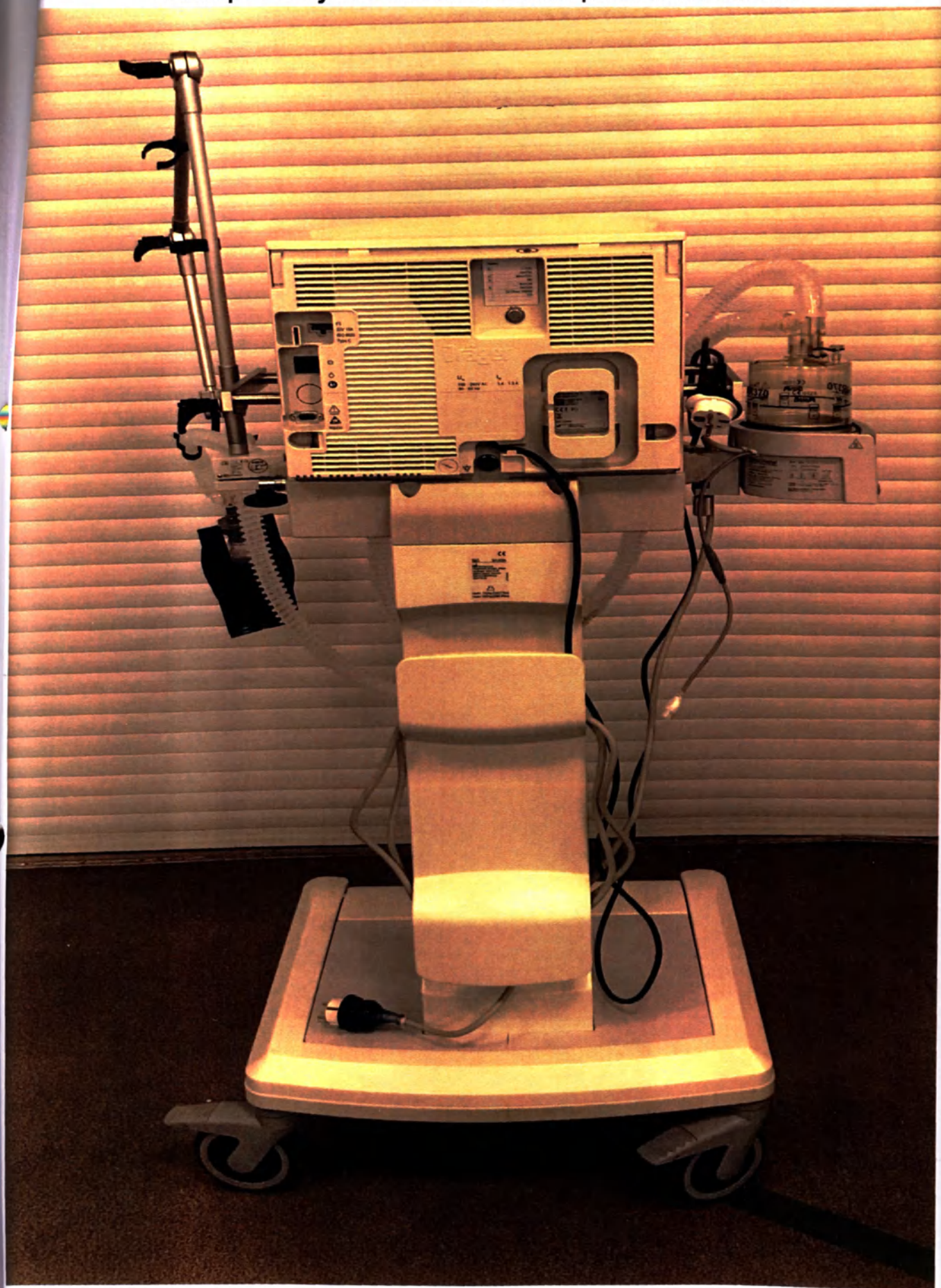
Фото 30 - Изделие в сборе (вид сзади).
