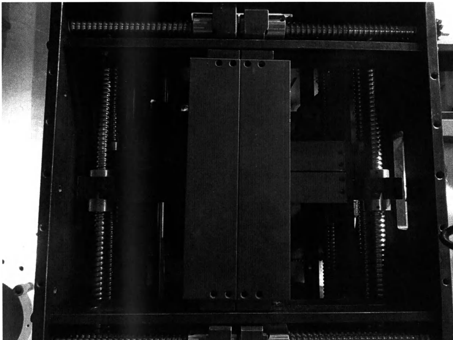
Коллиматор
