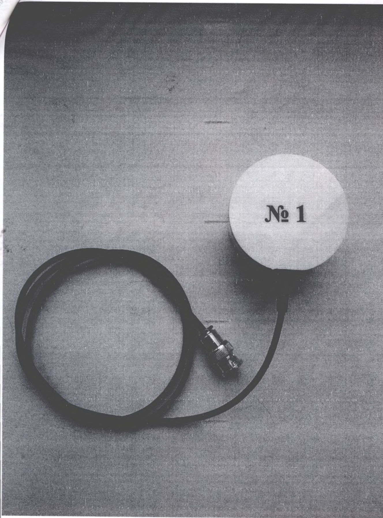
Излучатель № 1 (50 мм)
