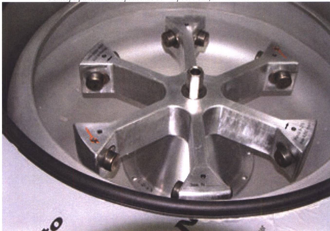
Фотографическое изображение 11 – Бакет-ротор на 6 стаканов
