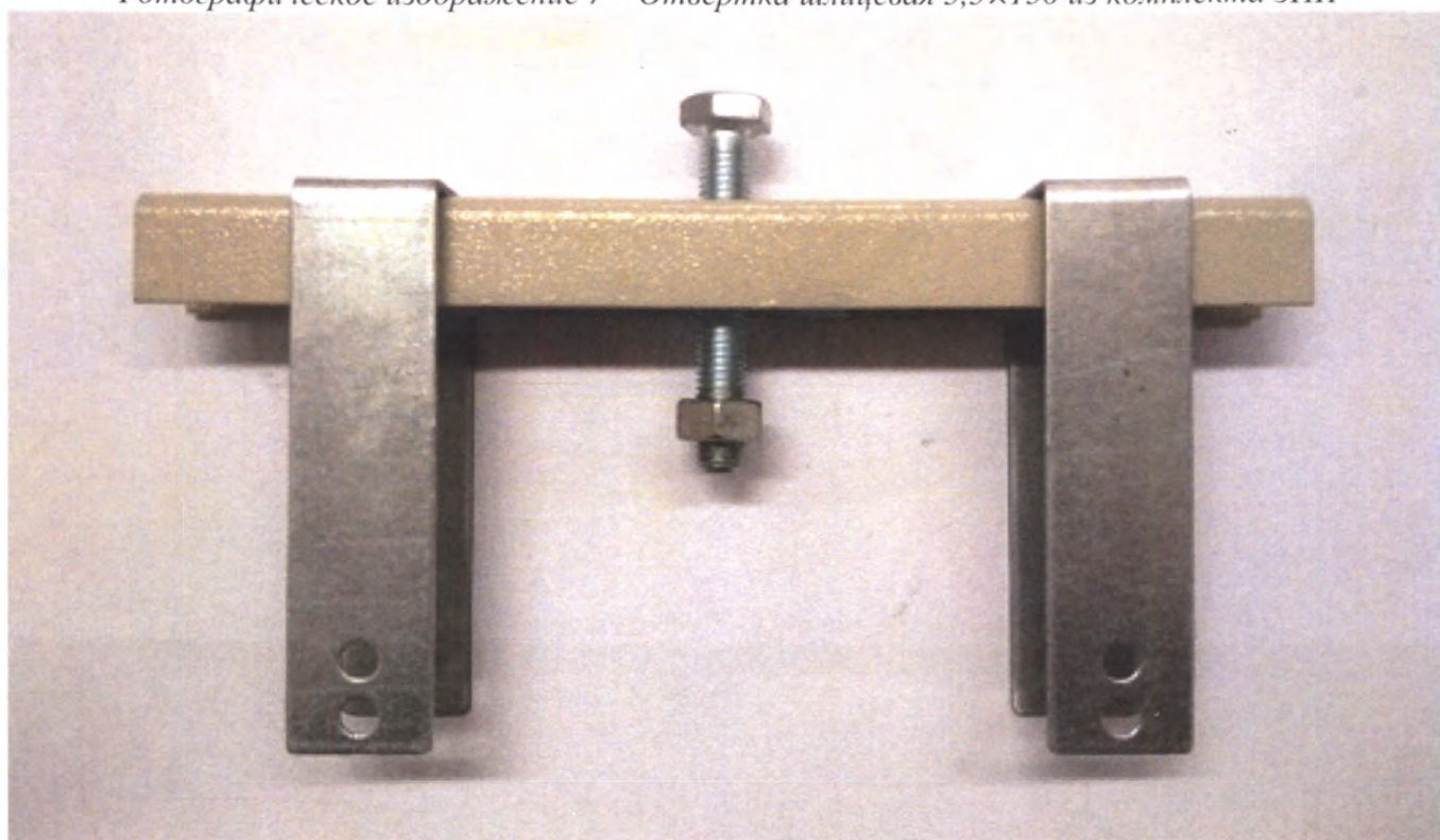
Фотографическое изображение 8 – Съёмник ротора из комплекта ЗИП
