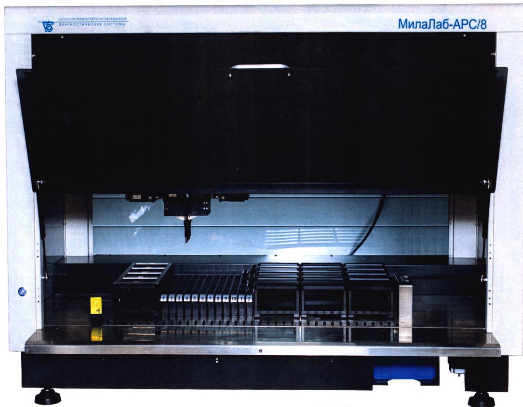
1. Станция автоматизированная раскапывающая МилаЛаб-АРС/8, общий вид
