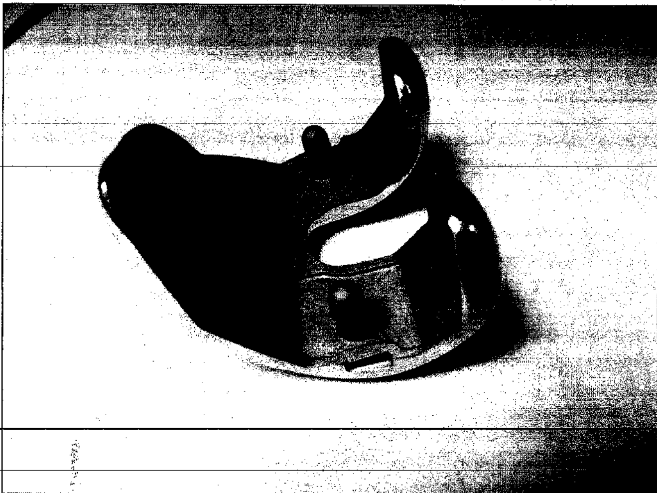
Компонент феморальный с сохранением задней крестообразной связки, левый, цементируемый (вид сверху)
