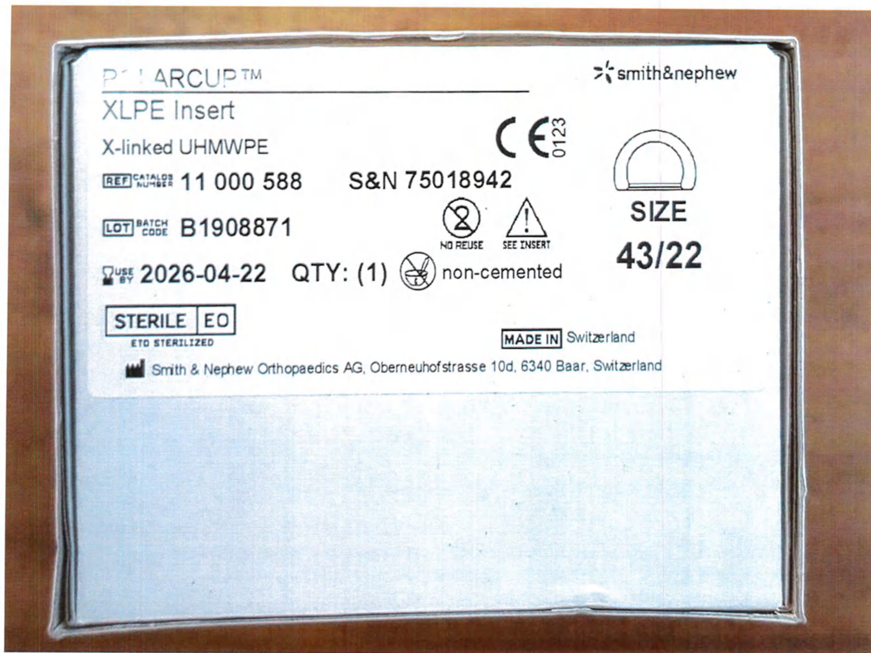
Рис. 35 – Вкладыш POLARCUP, XLPE, размер 22/43 мм, (маркировка потребительской упаковки)
