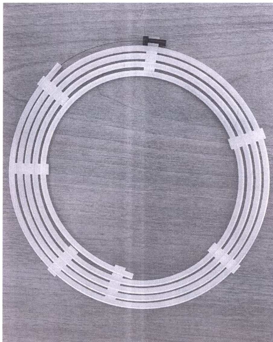
Устройство для реваскуляризации Solitaire X, варианты исполнения: Номинальный диаметр 6 мм, рабочая длина 40 мм, расстояние между маркерными полосками 10 мм – защитная спираль
