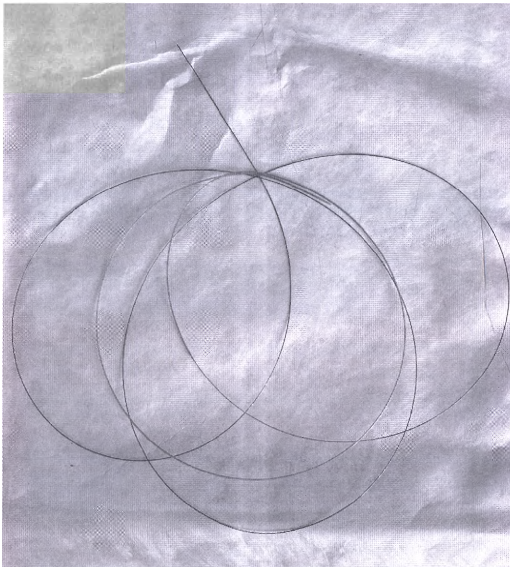
Устройство для реваскуляризации Solitaire X, варианты исполнения: Номинальный диаметр 4 мм, рабочая длина 20 мм, расстояние между маркерными полосками 5 мм – общий вид изделия
