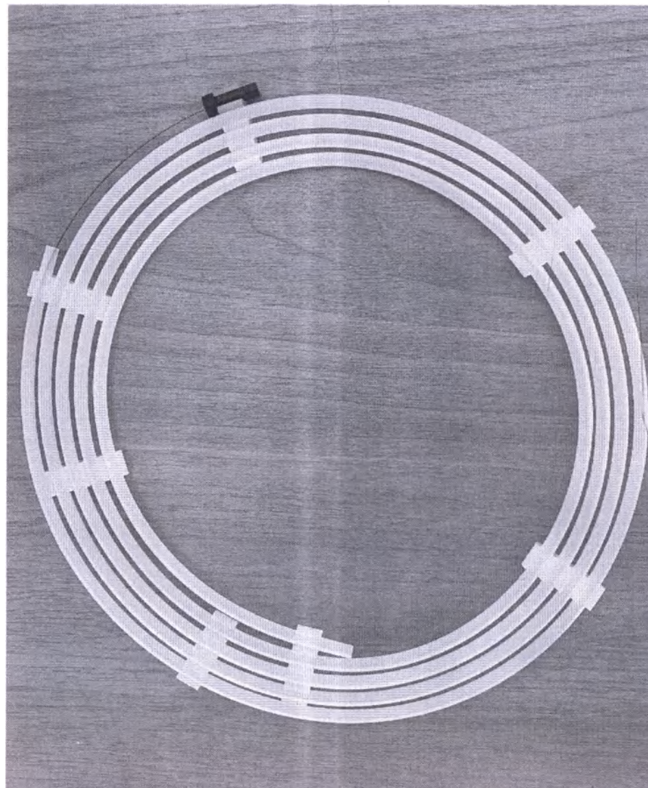
Устройство для реваскуляризации Solitaire X, варианты исполнения: Номинальный диаметр 4 мм, рабочая длина 40 мм, расстояние между маркерными полосками 10 мм – защитная спираль
