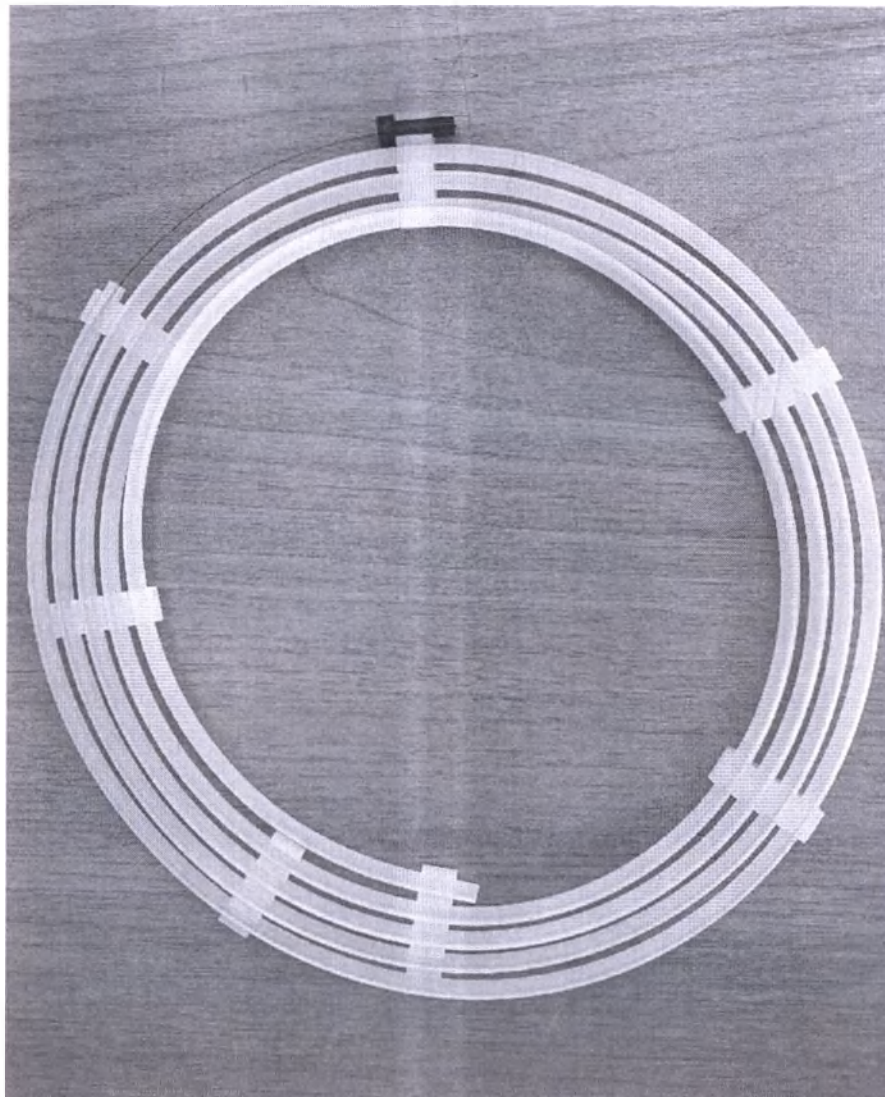
Устройство для реваскуляризации Solitaire X, варианты исполнения: Номинальный диаметр 6 мм, рабочая длина 24 мм, расстояние между маркерными полосками 6 мм – защитная спираль
